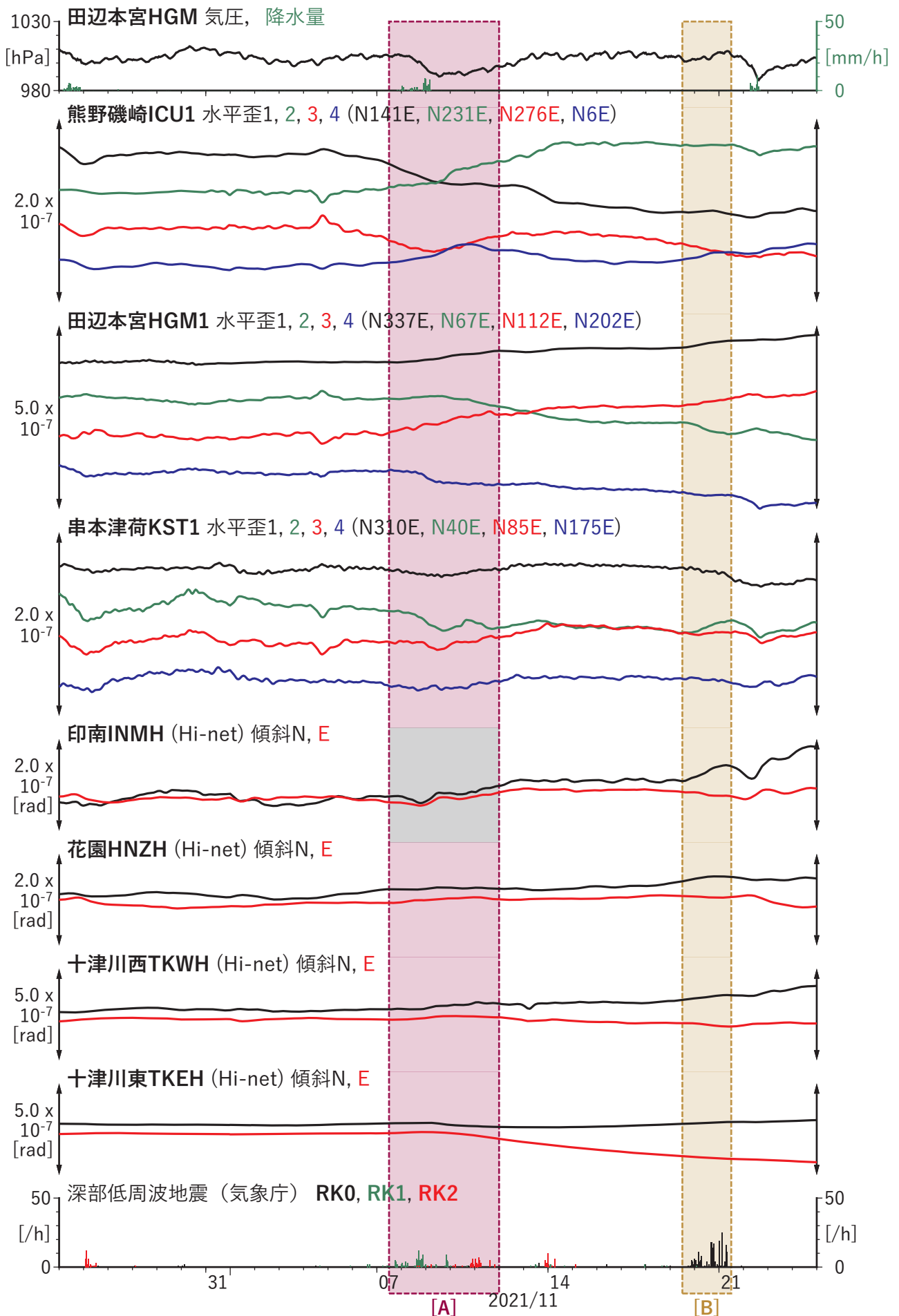
図2 歪・傾斜の時間変化 (2021/10/25 00:00-2021/11/25 00:00 (JST))
