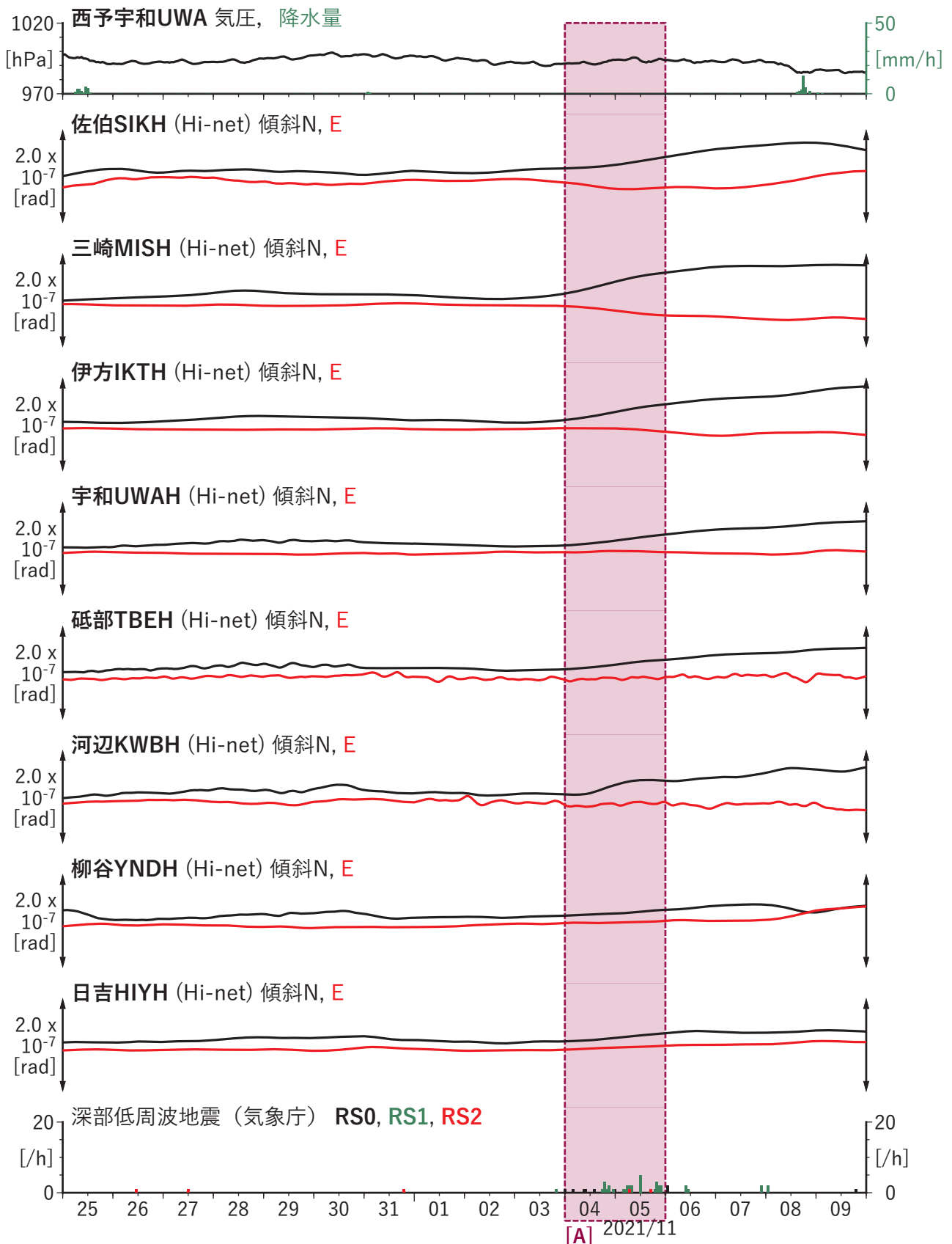
図6 歪・傾斜の時間変化(2) (2021/10/25 00:00-2021/11/10 00:00 (JST))
