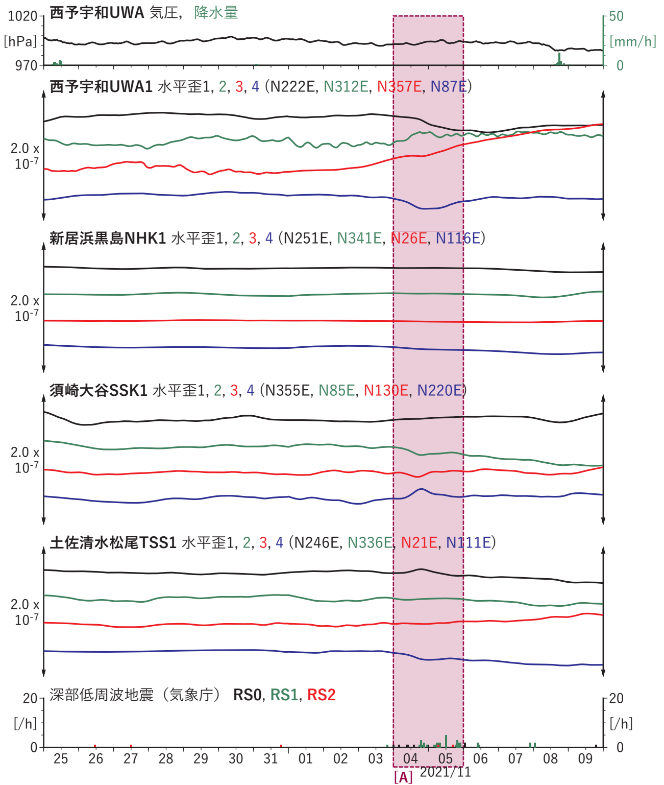
図6 歪・傾斜の時間変化(1) (2021/10/25 00:00-2021/11/10 00:00 (JST))
