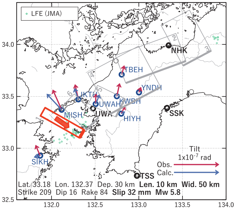
図7 2021/11/04-05の歪・傾斜変化（図6[A]）を説明する断層モデル。
