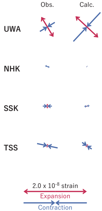
図7 2021/11/04-05の歪・傾斜変化（図6[A]）を説明する断層モデル。
