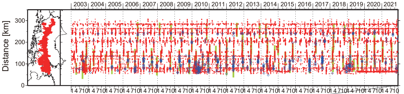
図1. 四国における2003年1月～2021年12月4日までの深部低周波微動の時空間分布(上図). 赤丸はエンベロープ相関・振幅ハイブリッド法 (Maeda and Obara, 2009) およびクラスタ処理 (Obara et al., 2010) によって1時間毎に自動処理された微動分布の重心である. 青菱形は
