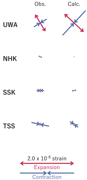
図3 2021/11/04-05の歪・傾斜変化（図2[A]）を説明する断層モデル。
