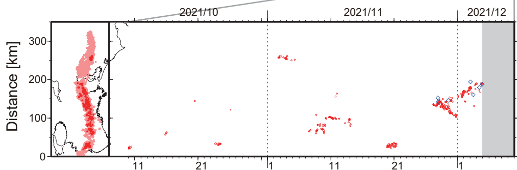
図1. 紀伊半島・東海地域における2003年1月～2021年12月4日までの深部低周波微動の時空間分布(上図). 赤丸はエンベロープ相関・振幅ハイブリッド法(Maeda and Obara, 2009)およびクラスタ処理(Obara et al., 2010)によって1時間毎に自動処理された微動分布の重心である. 青菱形は周期20秒に卓越する超低周波地震(Ito et al., 2007)である. 黄緑色の太線はこれまでに検出された短期的スロースリップイベント(SSE)を示す. 下図は2021年11月を中心とした期間の拡大図である.
