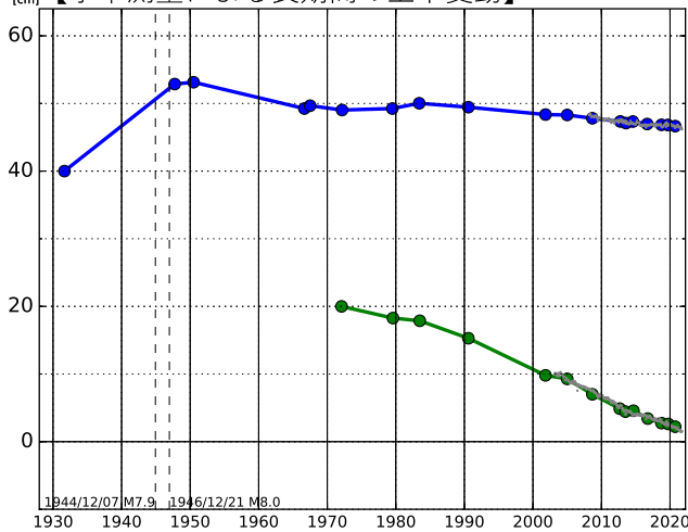
【水准測量による長期間の上下変動】
