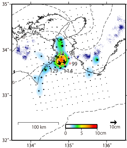
すべり量(カラー)及びすべりベクトルは水平面に投影したものを示す。 推定したすべり量が標準偏差 ( \sigma ) の3倍以上のグリッドを黒色表示している。
