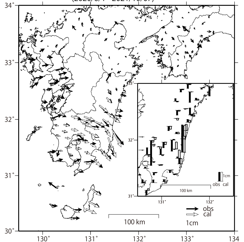
観測値 (黒) と計算値 (白) の比較 (2020/6/1 - 2021/10/07)
