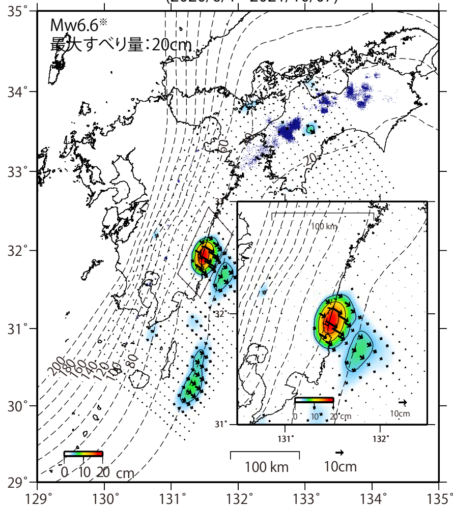
推定すべり分布 (2020/6/1 - 2021/10/07)
