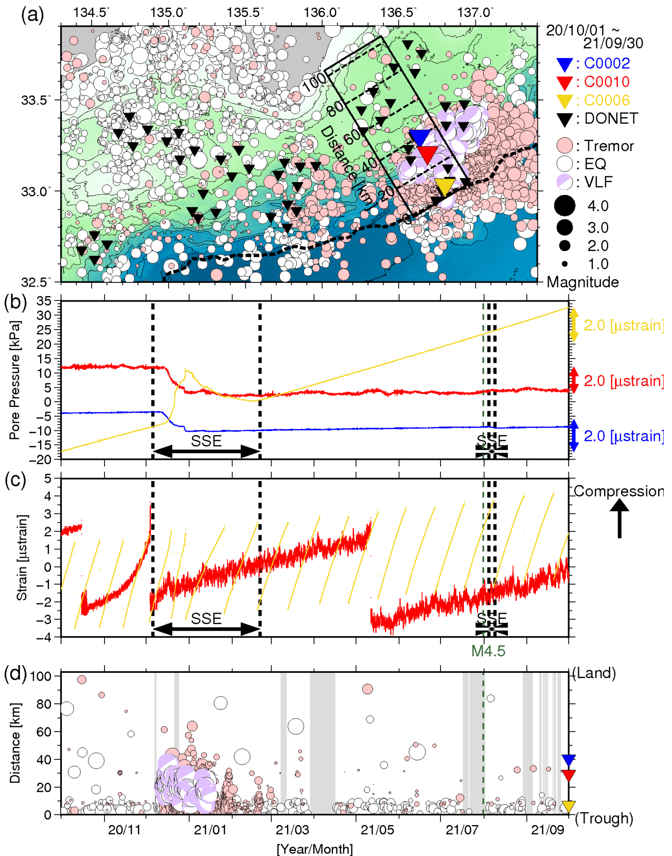
図4 直近1年間のSSE・低周波微動モニタリング(2020年10月1日~2021年9月30日)。図3と同様のシンボルにて表示している。(a)低周波微動の震央分布図。(b)間隙水圧変化。(c)体積歪変化。(d)低周波微動の時空間分布。超低周波地震のメカニズム解(●)についても低周波微動と同様に示す。体積歪変化は、基準値を超えると歪計内のバルブを開けてリセットするため、相対値のみを使用。灰色は、2020年12月7日~8日、21日~24日はサーバ不具合・入替期間、その他はエアガン発振期間を示す。(b-d)の緑点線は、2021年7月31日に発生した徳島県南部地震を示す。
