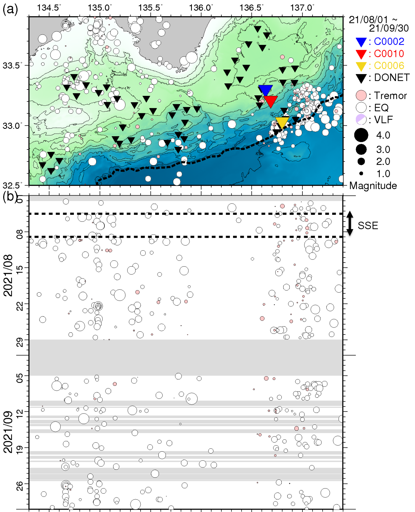
図5 直近2ヵ月間において熊野灘から室戸沖にて発生した低周波微動の時空間分布(2021年8月1日~2021年9月30日)。図3と同様のシンボルにて表示している。(a)低周波微動の震央分布図。(b)aに示した震央を経度方向へ投影した低周波微動の時空間分布図。
