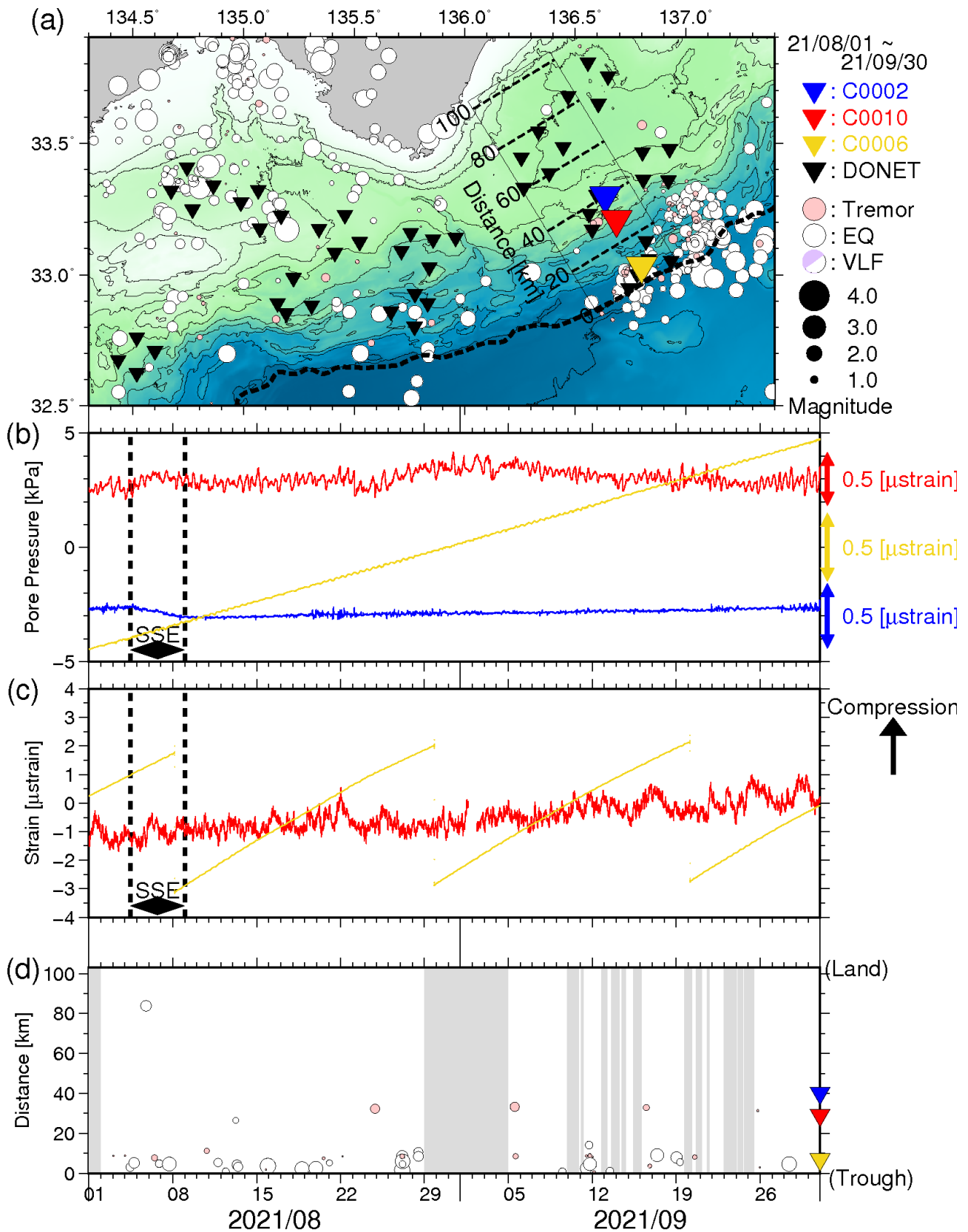
図3 直近2ヶ月間のSSE・低周波微動モニタリング(2021年8月1日~2021年9月30日)。(a) 低周波微動と通常の地震の震央分布図(●:低周波微動、○:通常の地震)。それぞれの震源深さが、0~15 km及び0~60 kmの範囲に決まったイベントのみを示す。▼▼▼は、それぞれC0002・C0010・C0006・DONET観測点を示す。破線はトラフ軸を示す。(b) 長期孔内観測点における間隙水圧変化(—:C0002、—:C0010、—:C0006)。(c) 長期孔内観測点における体積歪変化(—:C0010、—:C0006)。(d) 図3a中に実線で示した矩形領域内における、低周波微動と通常地震の時空間分布。灰色はエアガン発振期間。縦軸は、トラフ軸からの距離(km)を示す。
