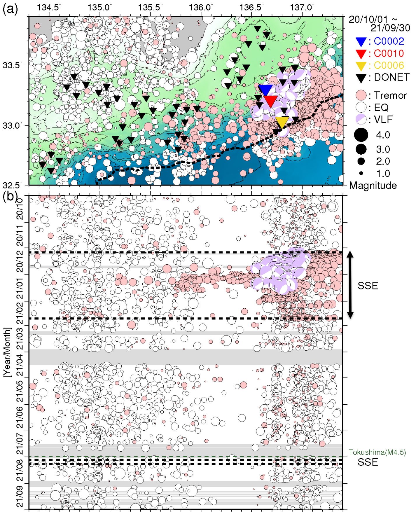
図6 直近1年間において熊野灘から室戸沖にて発生した低周波微動の時空間分布(2020年10月1日~2021年9月30日)。図4と同様のシンボルにて表示している。(a)低周波微動の震央分布図。(b)aに示した震央を経度方向へ投影した低周波微動の時空間分布図。超低周波地震のメカニズム解についても低周波微動と同様に示す。
