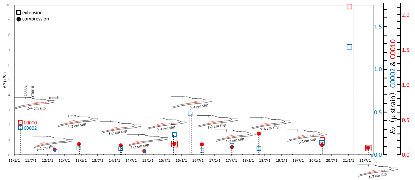
図7 孔内観測点において観測されたSSE発生時の間隙水圧変化(Araki et al., 2017; Ariyoshi et al. 2021)を加筆・修正)。間隙水圧変化( \Delta P )とそれらを体積歪( \epsilon_v )に換算したスケールを縦軸に示している。●・□は、それぞれ圧縮・伸長方向の間隙水圧変化を示す。青・赤のシンボルは、それぞれC0002・C0010の間隙水圧変化を示す。
