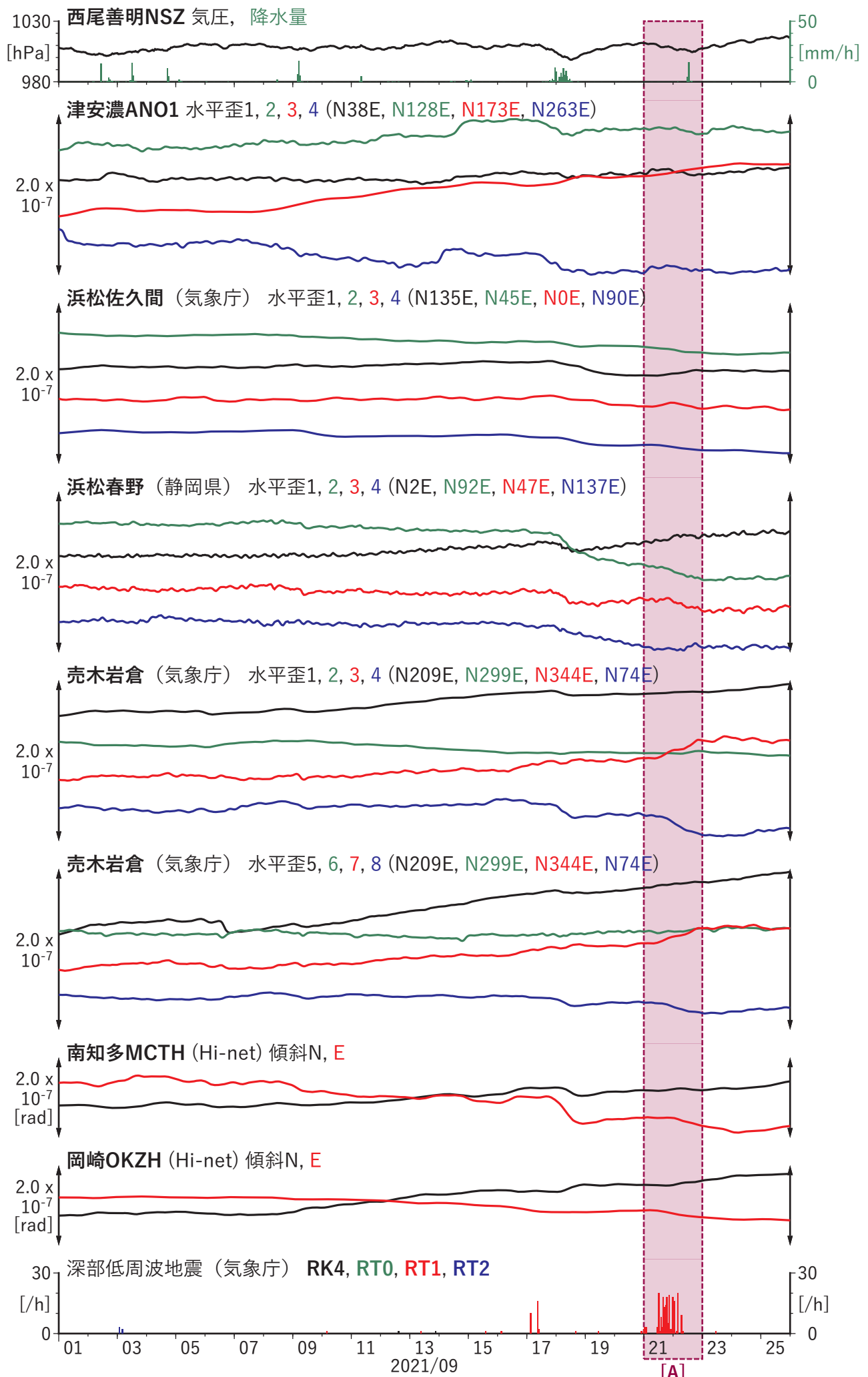
図3 歪・傾斜の時間変化 (2021/09/01 00:00 - 2021/09/26 00:00 (JST))
