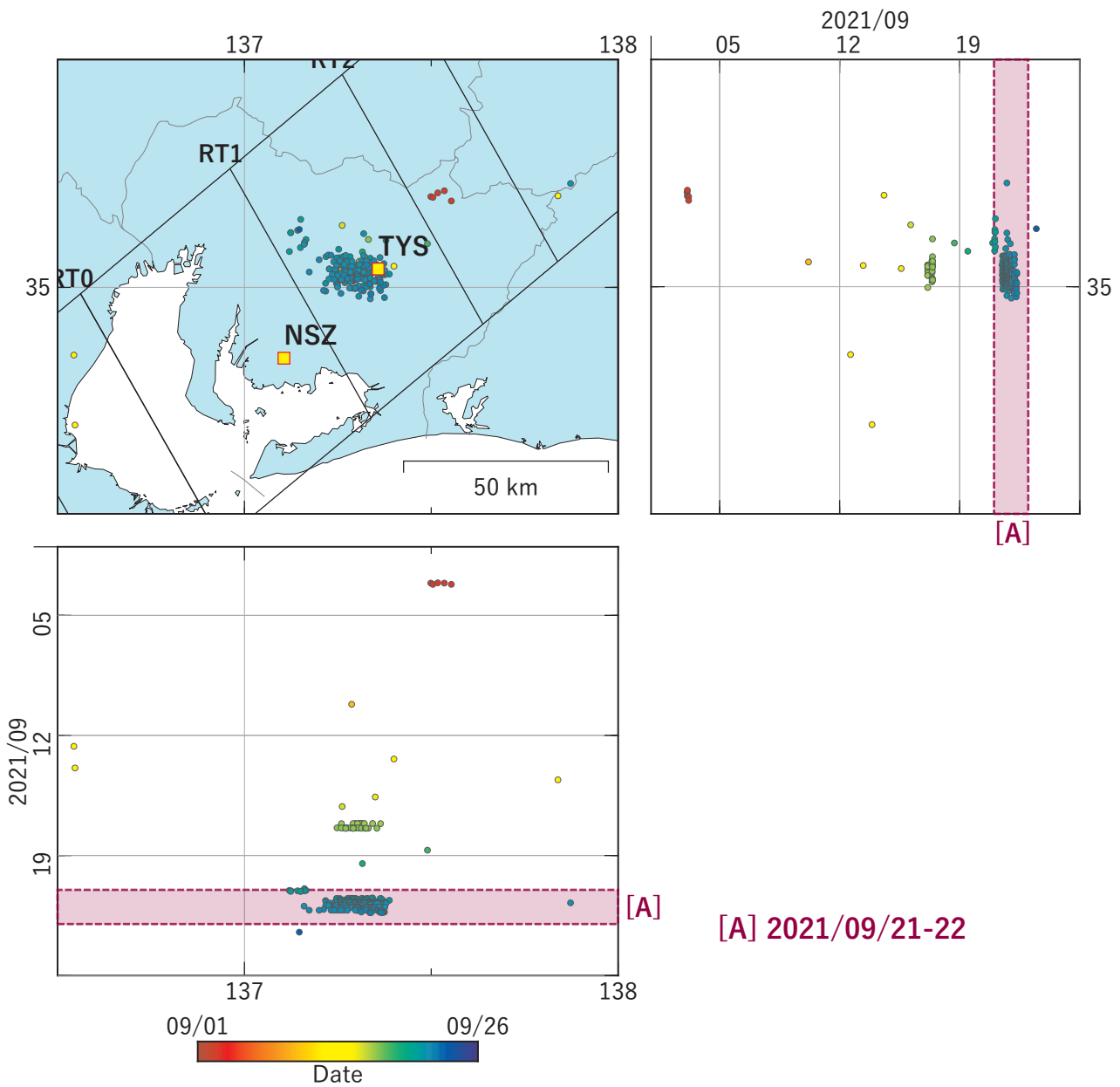
図1 東海地方における深部低周波地震の時空間分布図。 (2021/09/01 00:00 - 2021/09/26 00:00 (JST)) 気象庁カタログによる。
