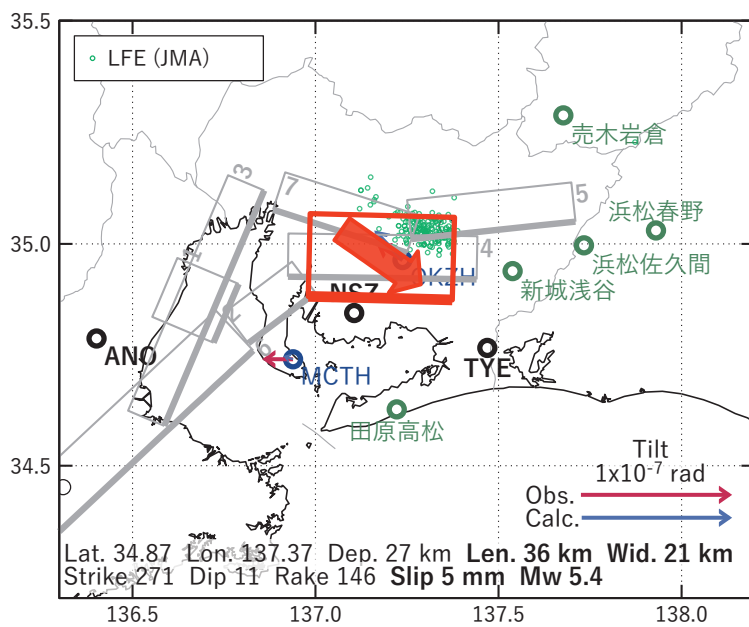
図4 2021/09/21-22 の歪・傾斜変化 (図2, 3[A]) を説明する断層モデル。
