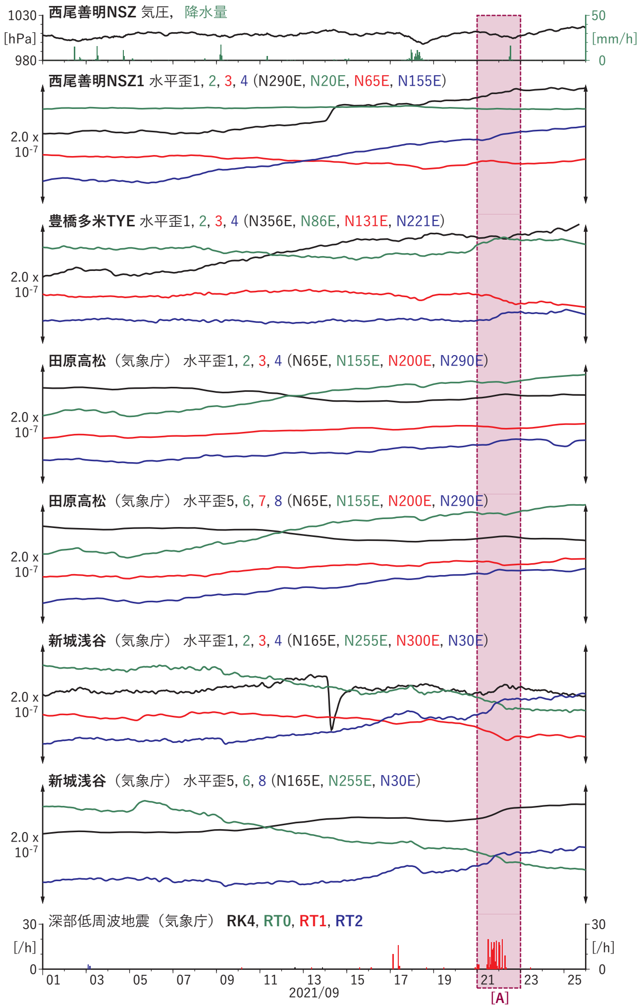
図2 歪の時間変化 (2021/09/01 00:00 - 2021/09/26 00:00 (JST))
