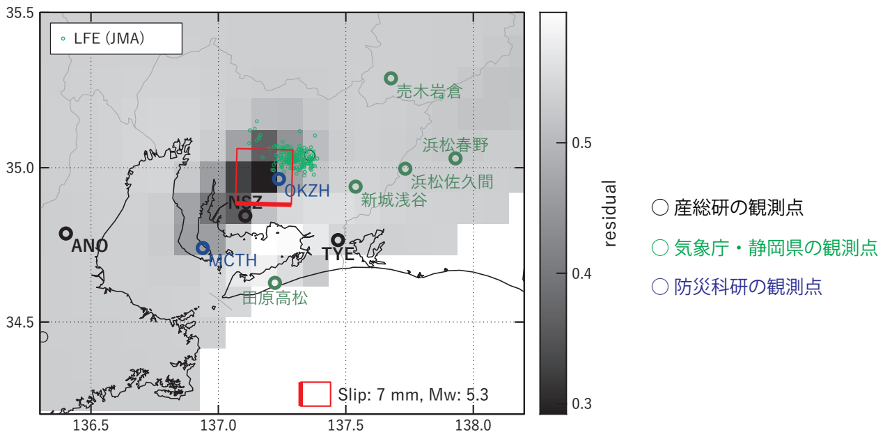
(b1) 推定した断層モデル
