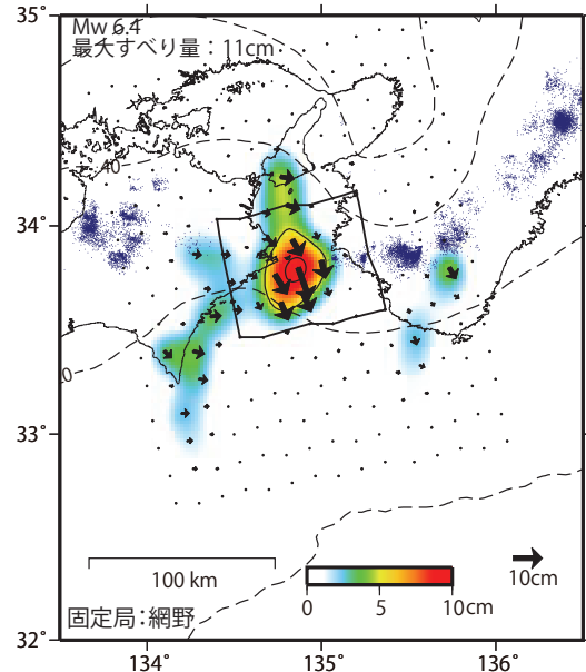
(C) 2019/1/1-2021/9/7 (全期間)
