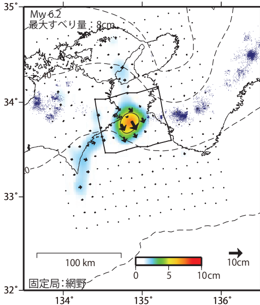
(B) 2019/1/1-2020/6/1 (前回)
