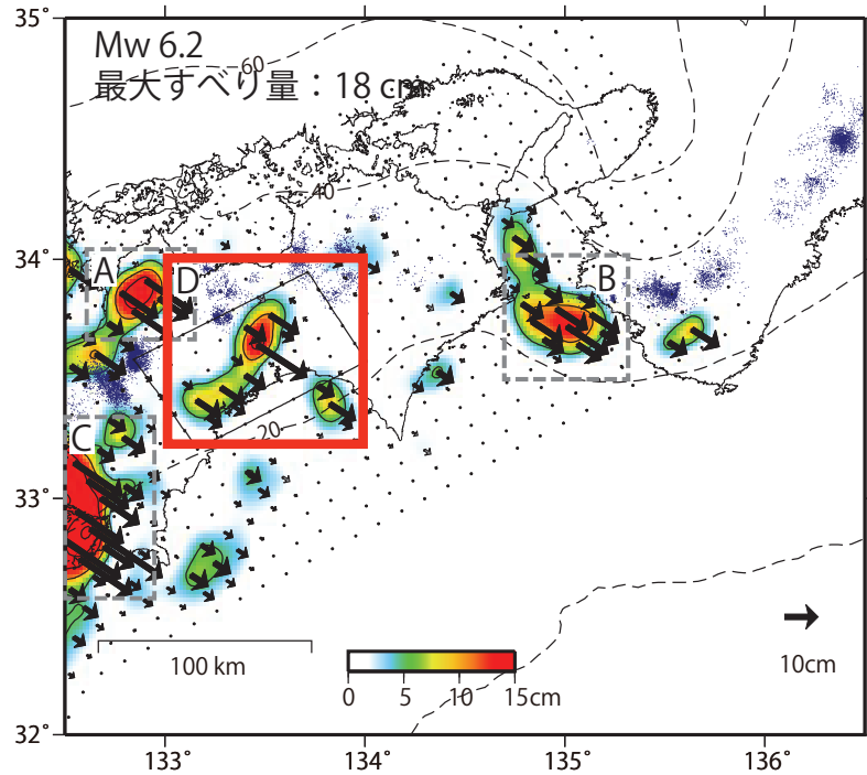
推定すべり分布 (2019/1/1 - 2021/9/9)
