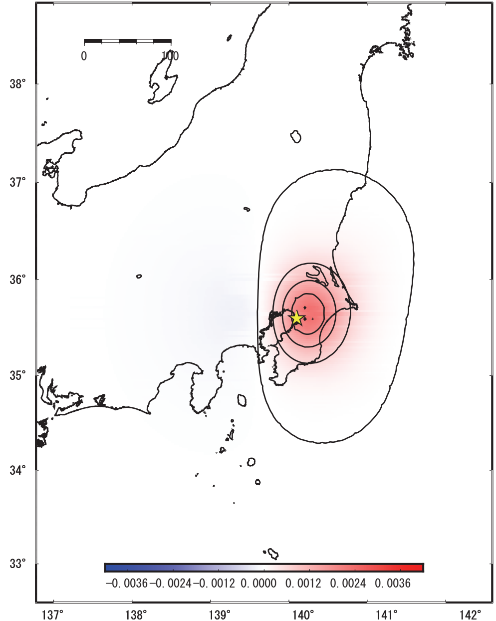
上下変動
