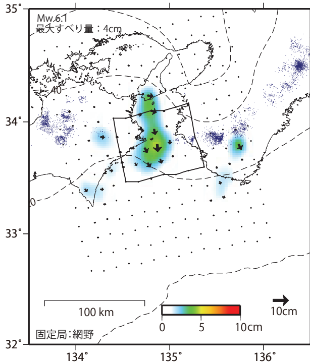
(B) 2019/1/1-2020/6/1 (前回)
