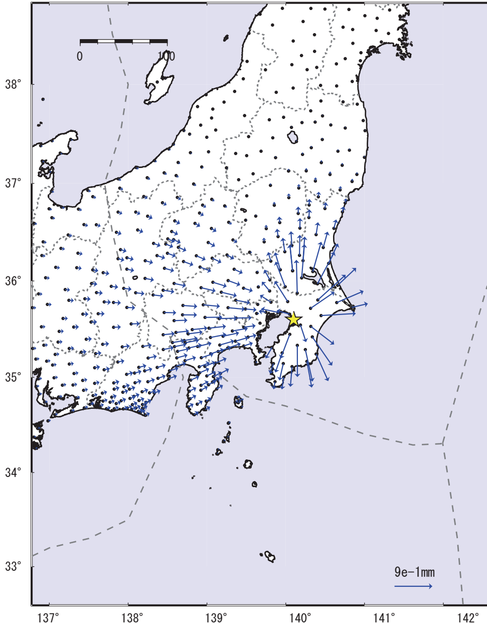
水平変動
