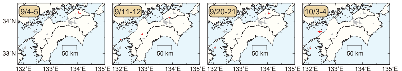
図2. 各期間に発生した微動分布 (赤丸). 灰丸は図1の拡大図で示した期間の微動分布.
