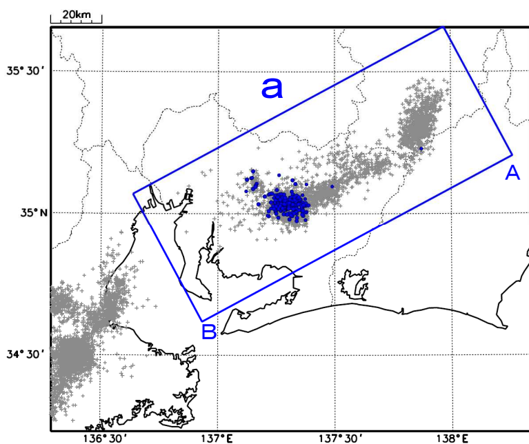
震央分布図(2018年4月1日～2021年9月26日、 深さ0～60km、Mすべて) 灰:2018年4月1日～2021年9月14日、 青:2021年9月15日以降
