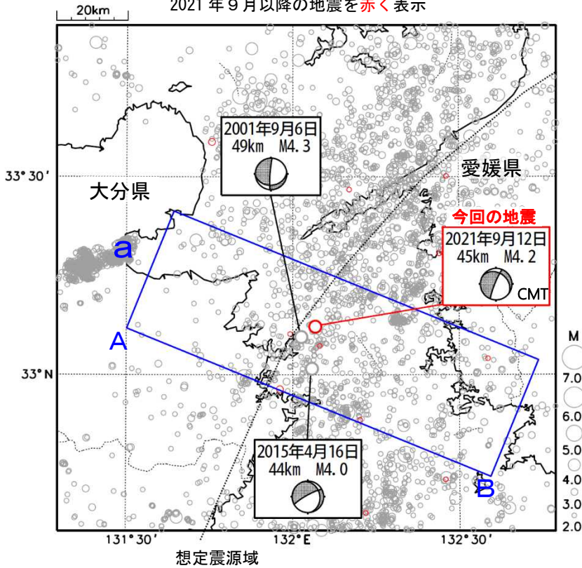
震央分布図 (1997年10月1日～2021年9月30日、 深さ0～90km、 M \geq 2.0 ) 2021年9月以降の地震を赤く表示
