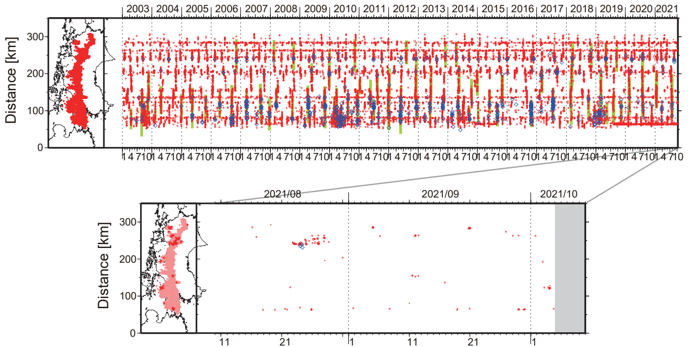
図1. 四国における2003年1月～2021年10月4日までの深部低周波微動の時空間分布(上图). 赤丸はエンベロープ相関・振幅ハイブリッド法 (Maeda and Obara, 2009) およびクラスタ処理 (Obara et al., 2010) によって1時間毎に自動処理された微動分布の重心である. 青菱形は周期20秒に卓越する超低周波地震 (Ito et al., 2007) である. 黄緑色太線は、これまでに検出された短期的スロースリップイベント (SSE) を示す. 下图は2021年9月を中心とした期間の拡大図である. 顕著な活動はとくにみられなかったものの、9月4～5日頃には香川県において、9月11～12日頃には愛媛県中部において、同じく11～12日頃には香川・徳島県境付近において、9月20～21日頃には香川県において、10月3～4日頃には愛媛県西部において、それぞれごく小規模な活動がみられた. このうち、9月11～12日頃の愛媛県中部の活動については、9月11日11:52頃に徳島県の深さ42kmで発生したM4.0 (Hi-net 暫定値) の地震後、12時頃より開始した.
