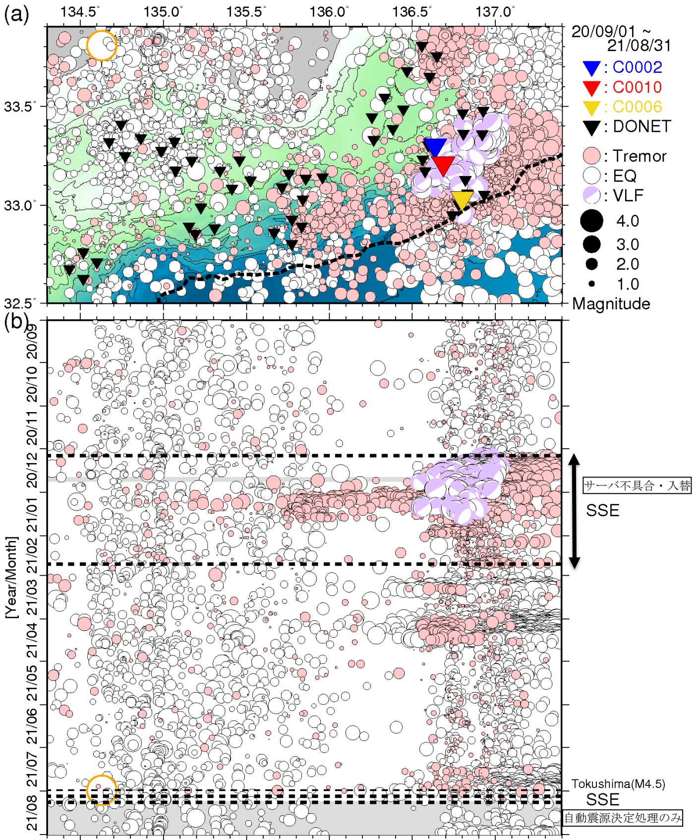
図6 直近1年間において熊野灘から室戸沖にて発生した低周波微動の時空間分布(2020年9月1日~2021年8月31日)。図3と同様のシンボルにて表示している。(a)低周波微動の震央分布図。(b)aに示した震央を経度方向へ投影した低周波微動の時空間分布図。超低周波地震のメカニズム解についても低周波微動と同様に示す。また、3月8日~4月及び7月11日~現在(9月7日まで実施予定)はエアガン信号が含まれているが、これに関連する発振点情報が入手できていないため、未解析となっている。
