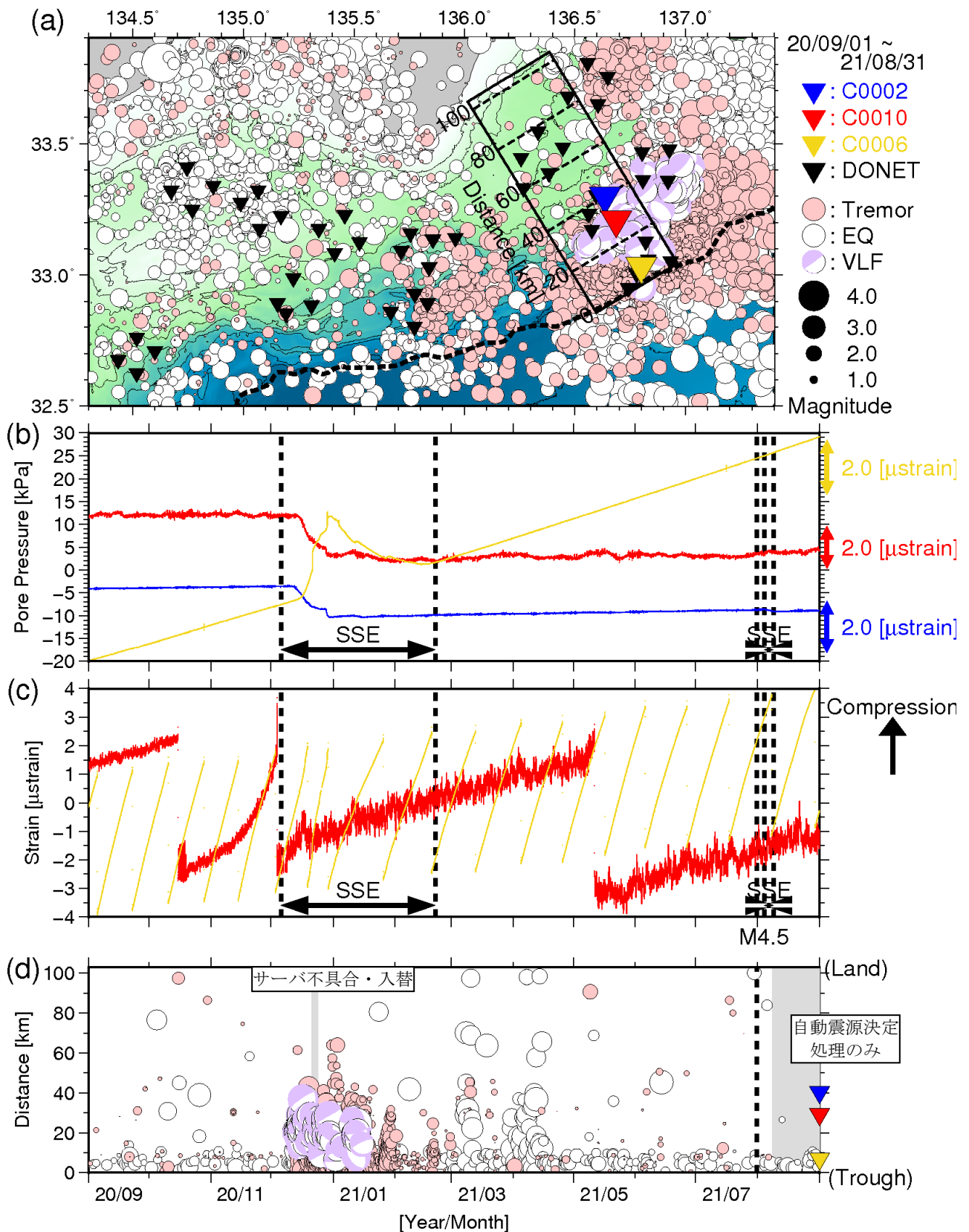
図4 直近1年間のSSE・低周波微動モニタリング(2020年9月1日~2021年8月31日)。図3と同様のシンボルにて表示している。(a)低周波微動の震央分布図。(b)間隙水圧変化。(c)体積歪変化。(d)低周波微動の時空間分布。超低周波地震のメカニズム解(●)についても低周波微動と同様に示す。体積歪変化は、基準値を超えると歪計内のバルブを開けてリセットするため、相対値のみを使用。なお、2020年12月7日~8日、21日~24日はサーバ不具合・入替のため、8月8日以降はネットワーク障害のため、各期間においてデータ解析が一部未処理となっている。点線で示す地震情報については、図3および図6を参照。
