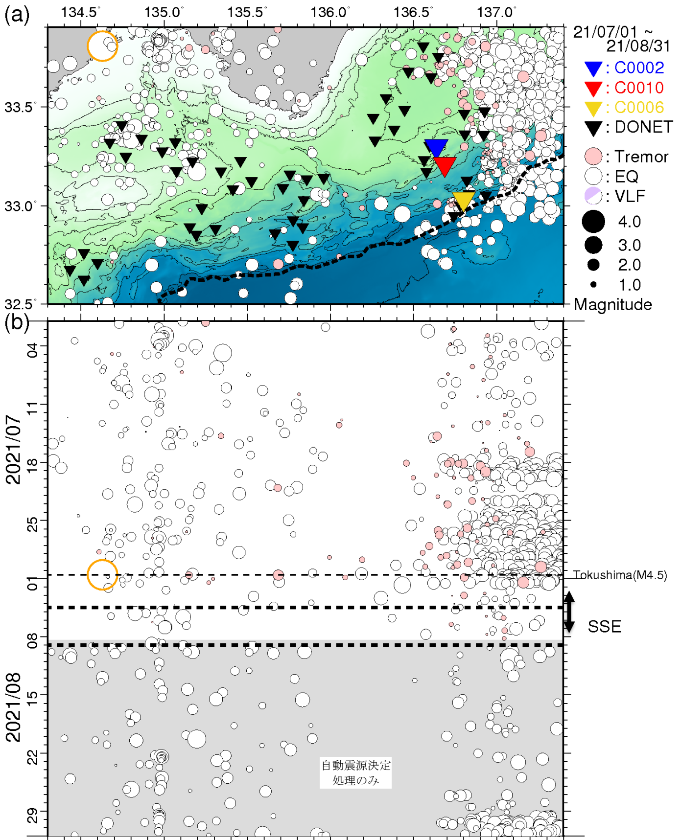
図5 直近2ヵ月間において熊野灘から室戸沖にて発生した低周波微動の時空間分布(2021年7月1日~2021年8月31日)。図3と同様のシンボルにて表示している。(a)低周波微動の震央分布図。(b)aに示した震央を経度方向へ投影した低周波微動の時空間分布図。2021年8月8日以降はネットワーク障害のため、微動と地震カタログの照合は一部未処理である。○は2021年7月31日に発生した徳島県南部地震を示す。
