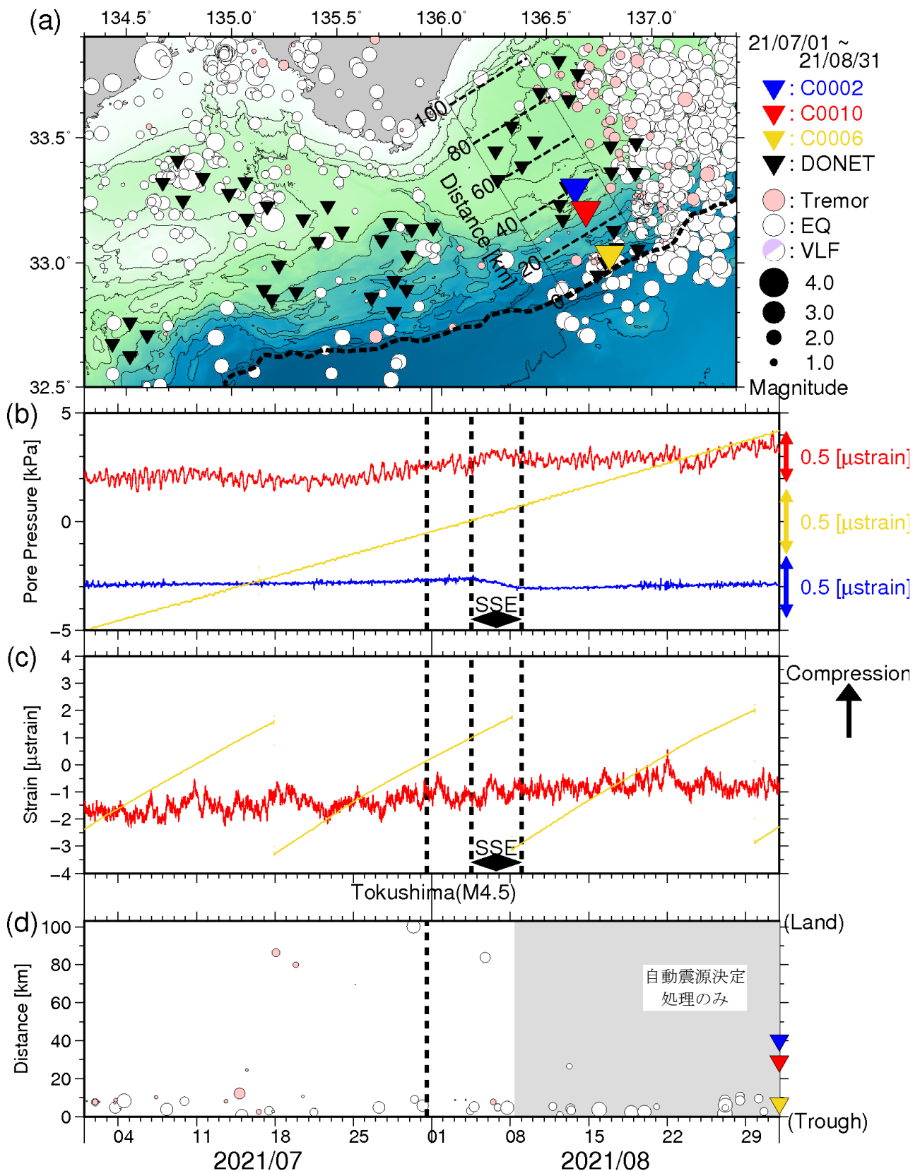
図3 直近2ヶ月間のSSE・低周波微動モニタリング(2021年7月1日~2021年8月31日)。(a) 低周波微動と通常の地震の震央分布図(●:低周波微動、○:通常の地震)。それぞれの震源深さが、0~15 km及び0~60 kmの範囲に決まったイベントのみを示す。▼▼▼▼は、それぞれC0002・C0010・C0006・DONET観測点を示す。破線はトラフ軸を示す。(b) 長期孔内観測点における間隙水圧変化(—:C0002、—:C0010、—:C0006)。(c) 長期孔内観測点における体積歪変化(—:C0010、—:C0006)。(d) 低周波微動と通常地震の時空間分布。図3a中に実線で示した矩形領域内において発生したイベントについて示す。縦軸は、トラフ軸からの距離(km)を示す。
