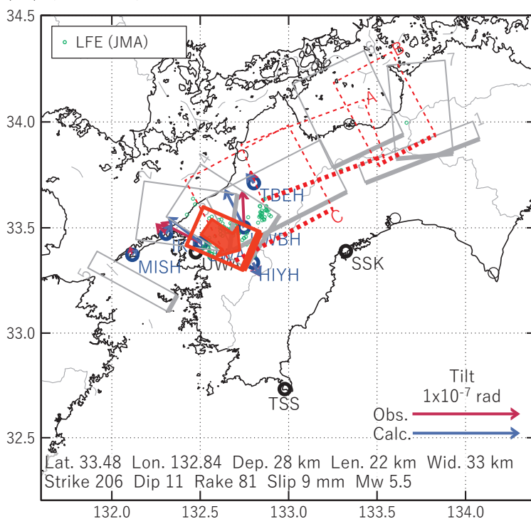
図7 2021/07/28の歪・傾斜変化（図2,3[D]）を説明する断層モデル。
