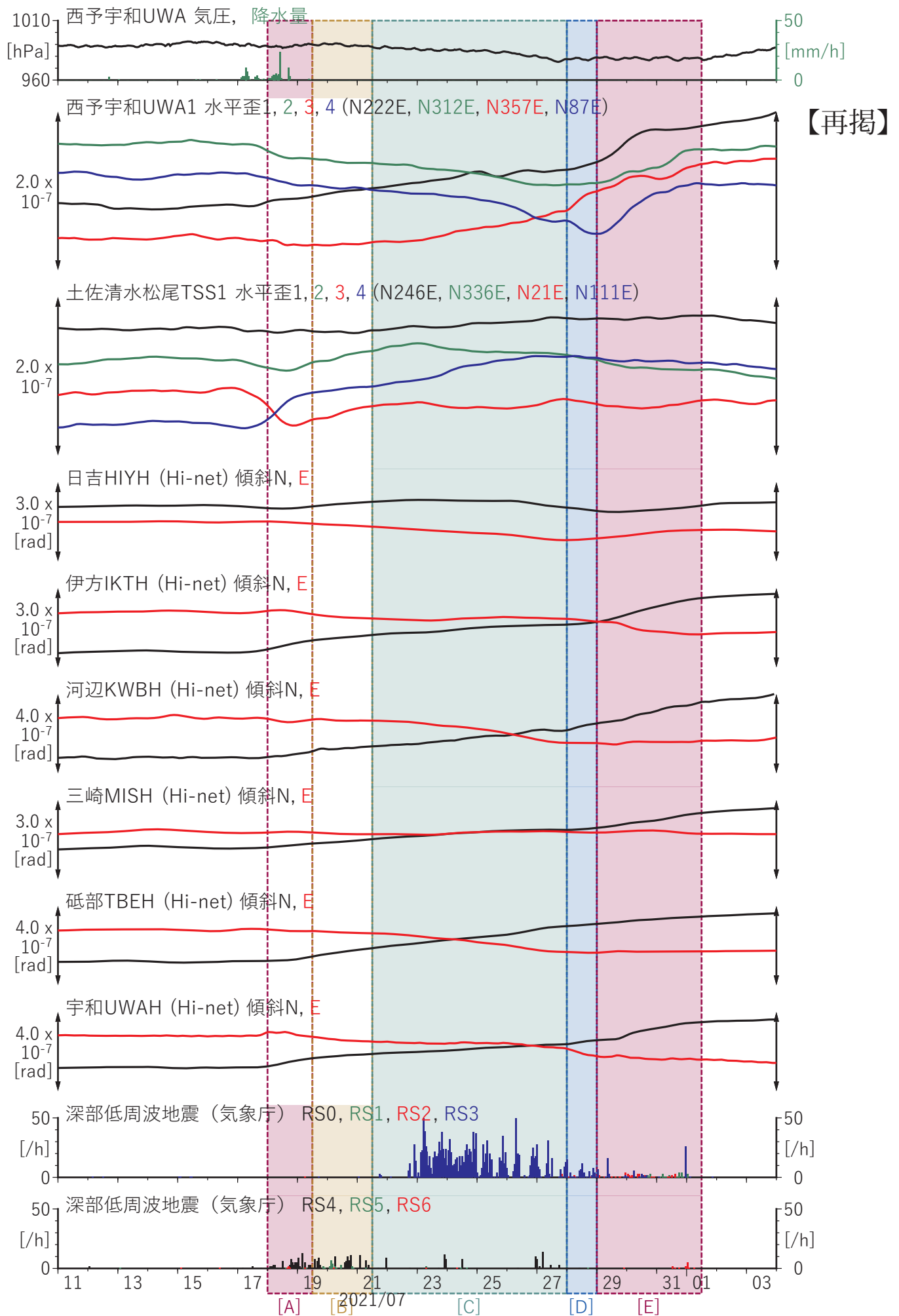
図3 四国西部における歪・傾斜の観測結果 (2021/07/11 00:00 - 2021/08/03 00:00 (JST))
