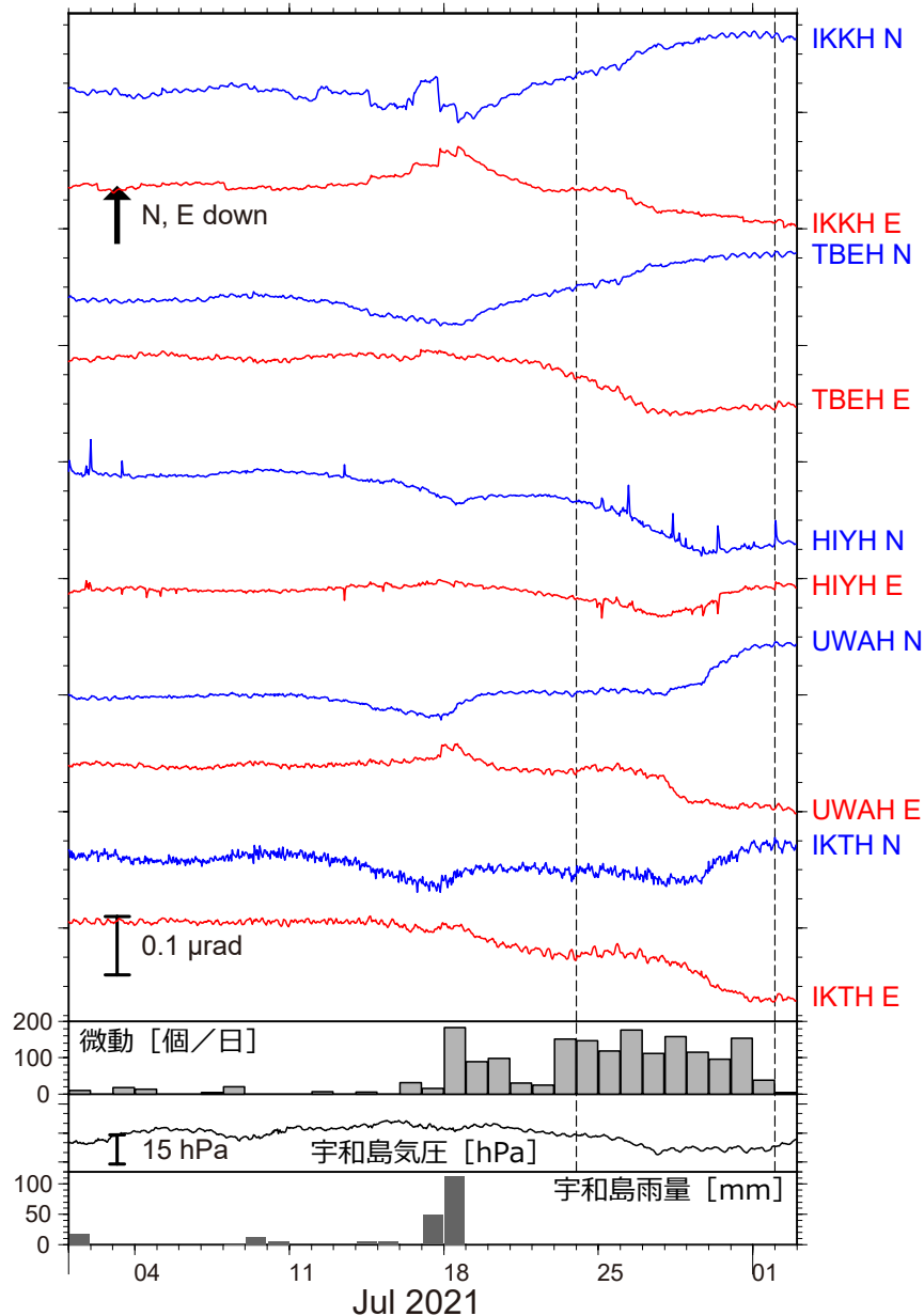
図 1：2021 年 7 月 1 日～8 月 2 日の傾斜時系列。上方向への変化が北・東下がりの傾斜変動を表し、BAYTAP-G により潮汐・気圧応答成分を除去した。7 月 24 日～8 月 1 日の傾斜変化ベクトルを図 2 に示す。四国中西部での微動活動度・気象庁宇和島観測点の気圧・雨量をあわせて示す。
