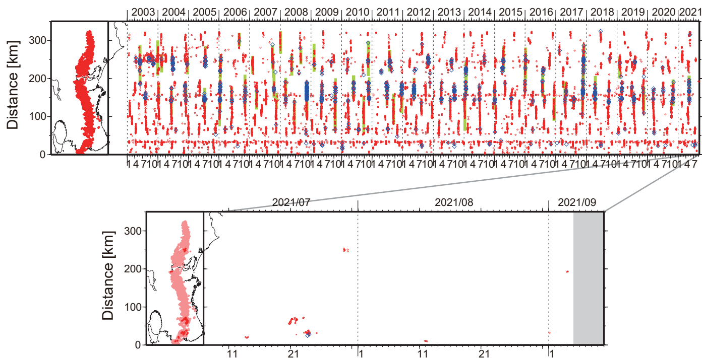
図 1. 紀伊半島・東海地域における 2003 年 1 月～2021 年 9 月 4 日までの深部低周波微動の時空間分布 (上図). 赤丸はエンベロープ相関・振幅ハイブリッド法 (Maeda and Obara, 2009) およびクラスタ処理 (Obara et al., 2010) によって 1 時間毎に自動処理された微動分布の重心である. 青菱形は周期 20 秒に卓越する超低周波地震 (Ito et al., 2007) である. 黄緑色の太線はこれまでに検出された短期的スロースリップイベント (SSE) を示す. 下図は 2021 年 8 月を中心とした期間の拡大図である. 顕著な活動はとくにみられなかったものの, 8 月 11～12 日頃に和歌山県中部において, ごく小規模な活動がみられた. 9 月 1 日 2:55 頃に和歌山県中部の深さ 46km で発生した M4.0 (Hi-net 暫定値) の地震後, 3 時台には, 和歌山県中部において微動活動がみられた.
