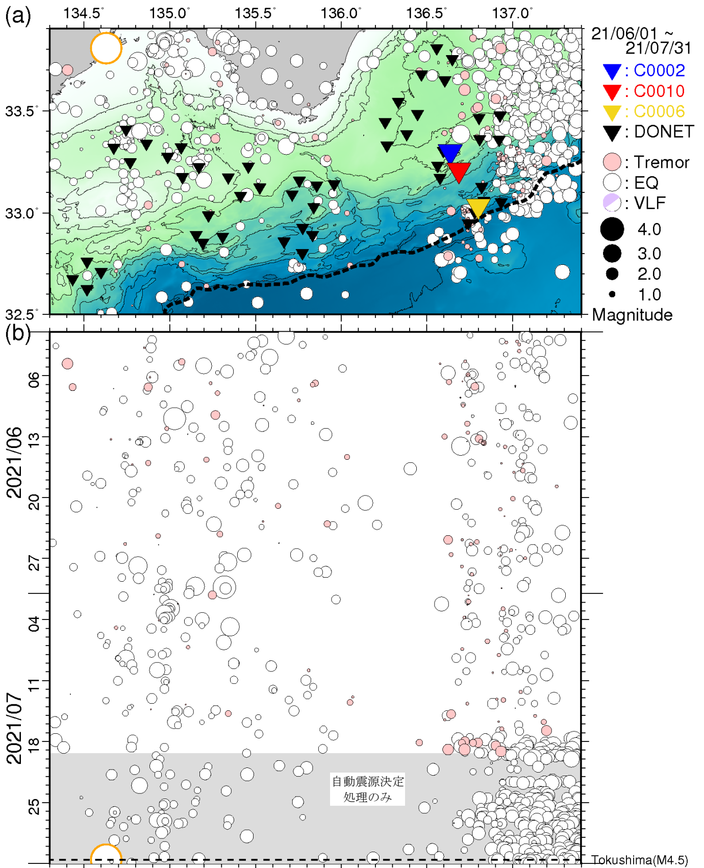
図5 直近2ヵ月間において熊野灘から室戸沖にて発生した低周波微動の時空間分布(2021年6月1日~2021年7月31日)。図3と同様のシンボルにて表示している。(a)低周波微動の震央分布図。(b)aに示した震央を経度方向へ投影した低周波微動の時空間分布図。2021年3月29日以降はネットワーク障害のため、微動と地震カタログの照合は一部未処理である。○は2021年7月31日に発生した徳島県南部地震を示す。
