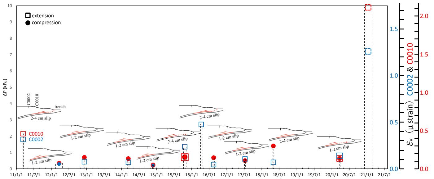
図7 孔内観測点において観測された SSE 発生時の間隙水圧変化 (Araki et al., 2017; Ariyoshi et al. 2021) を加筆・修正)。間隙水圧変化 ( \Delta P ) とそれらを体積歪 ( \epsilon_v ) に換算したスケールを縦軸に示している。●・□は、それぞれ圧縮・伸長方向の間隙水圧変化を示す。青・赤のシンボルは、それぞれ C0002・C0010 の間隙水圧変化を示す。
