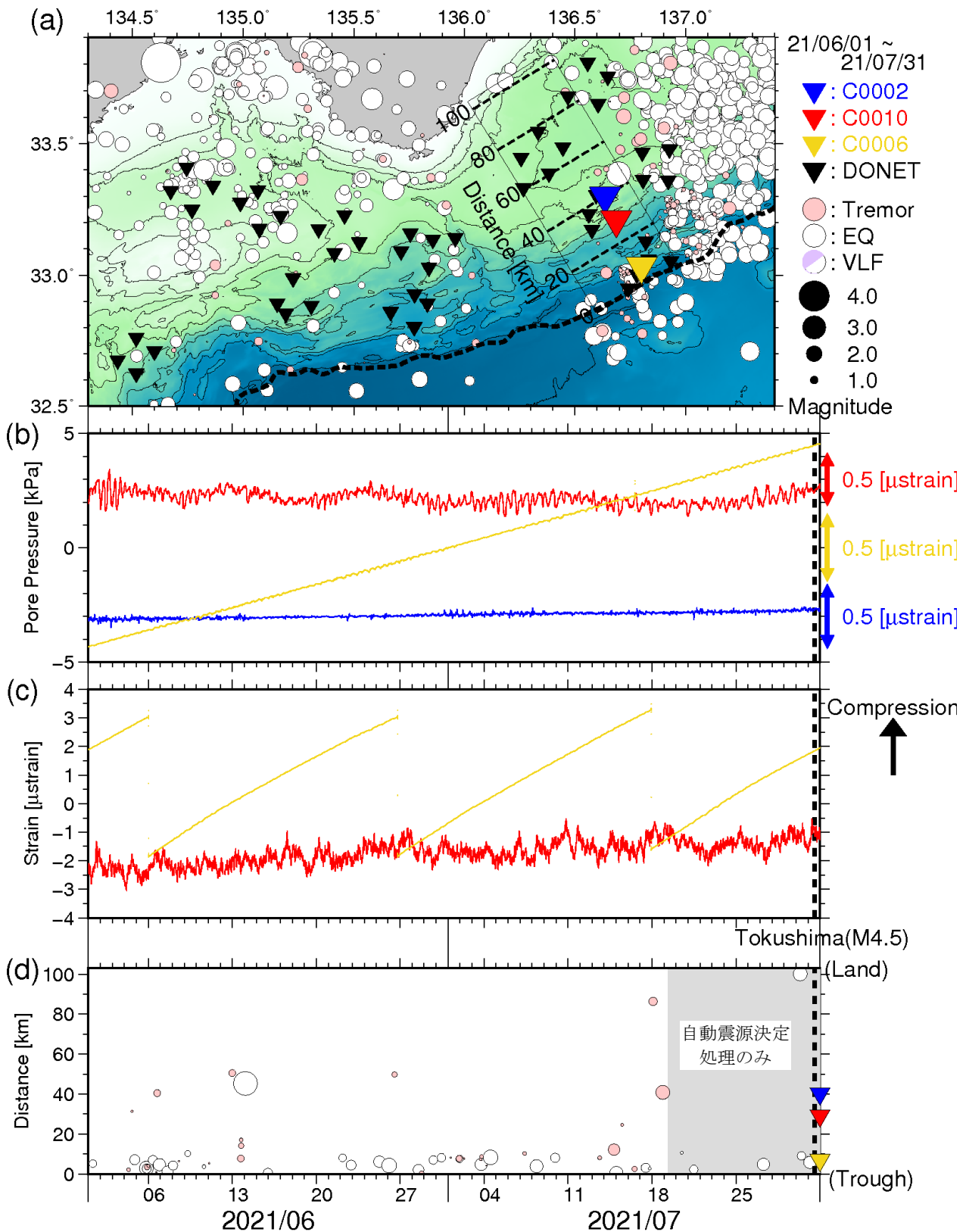
図3 直近2ヶ月間のSSE・低周波微動モニタリング(2021年6月1日~2021年7月31日)。(a) 低周波微動と通常の地震の震央分布図(●:低周波微動、○:通常の地震)。それぞれの震源深さが、0~15 km及び0~60 kmの範囲に決まったイベントのみを示す。▼、▼、▼、▼は、それぞれC0002・C0010・C0006・DONET観測点を示す。破線はトラフ軸を示す。(b) 長期孔内観測点における間隙水圧変化(—:C0002、—:C0010、—:C0006)。(c) 長期孔内観測点における体積歪変化(—:C0010、—:C0006)。(d) 低周波微動と通常地震の時空間分布。図3a中に実線で示した矩形領域内において発生したイベントについて示す。縦軸は、トラフ軸からの距離(km)を示す。
