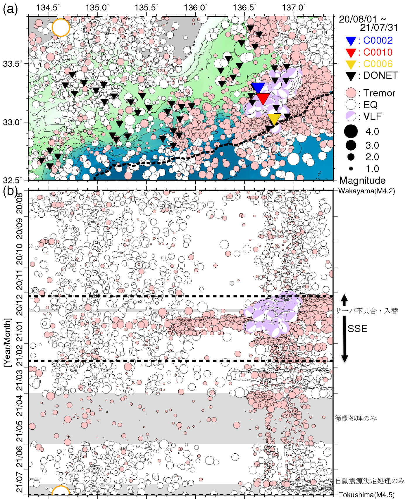
図6 直近1年間において熊野灘から室戸沖にて発生した低周波微動の時空間分布(2020年8月1日~2021年7月31日)。図3と同様のシンボルにて表示している。(a)低周波微動の震央分布図。(b)aに示した震央を経度方向へ投影した低周波微動の時空間分布図。超低周波地震のメカニズム解についても低周波微動と同様に示す。また、3月8日~4月及び7月11日~現在(9月7日まで実施予定)はエアガン信号が含まれているが、これに関連する発振点情報が入手できていないため、未解析となっている。
