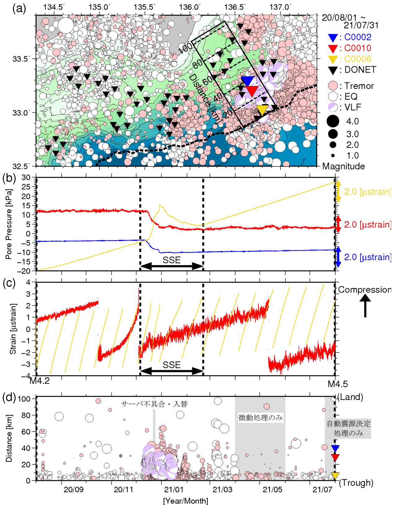
図4 直近1年間のSSE・低周波微動モニタリング(2020年8月1日~2021年7月31日)。図3と同様のシンボルにて表示している。(a)低周波微動の震央分布図。(b)間隙水圧変化。(c)体積歪変化。(d)低周波微動の時空間分布。超低周波地震のメカニズム解(●)についても低周波微動と同様に示す。体積歪変化は、基準値を超えると歪計内のバルブを開けてリセットするため、相対値のみを使用。なお、2020年12月7日~8日、21日~24日はサーバ不具合・入替のため、3月29日以降はネットワーク障害のため、各期間においてデータ解析が一部未処理となっている。点線で示す地震情報については、図3および図6を参照。
