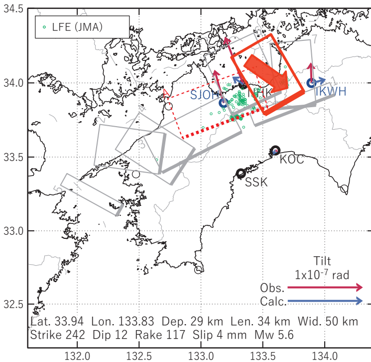
図5 2021/07/19PM-21AMの歪・傾斜変化 (図2,3[B]) を説明する断層モデル。
