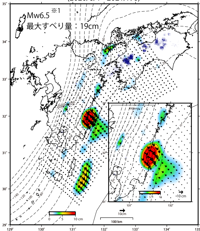
推定すべり分布 (2020/6/1 - 2021/7/6)
