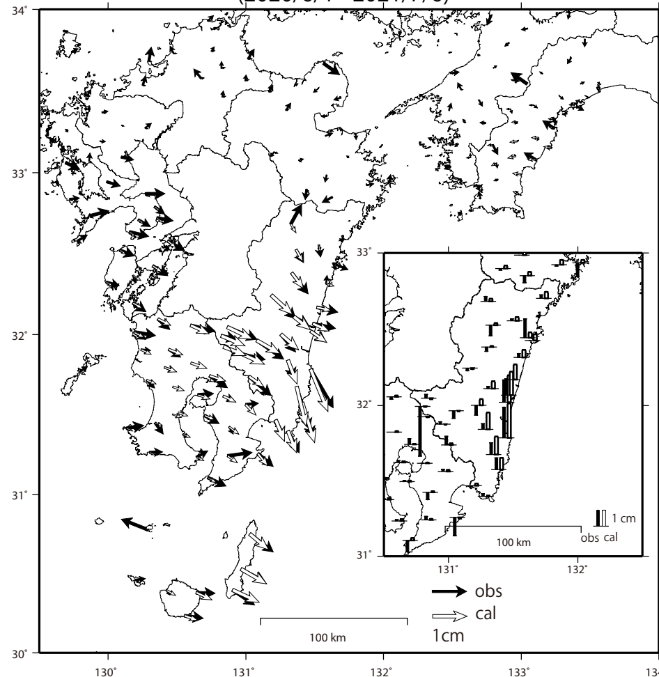
観測値 (黒) と計算値 (白) の比較 (2020/6/1 - 2021/7/6)
