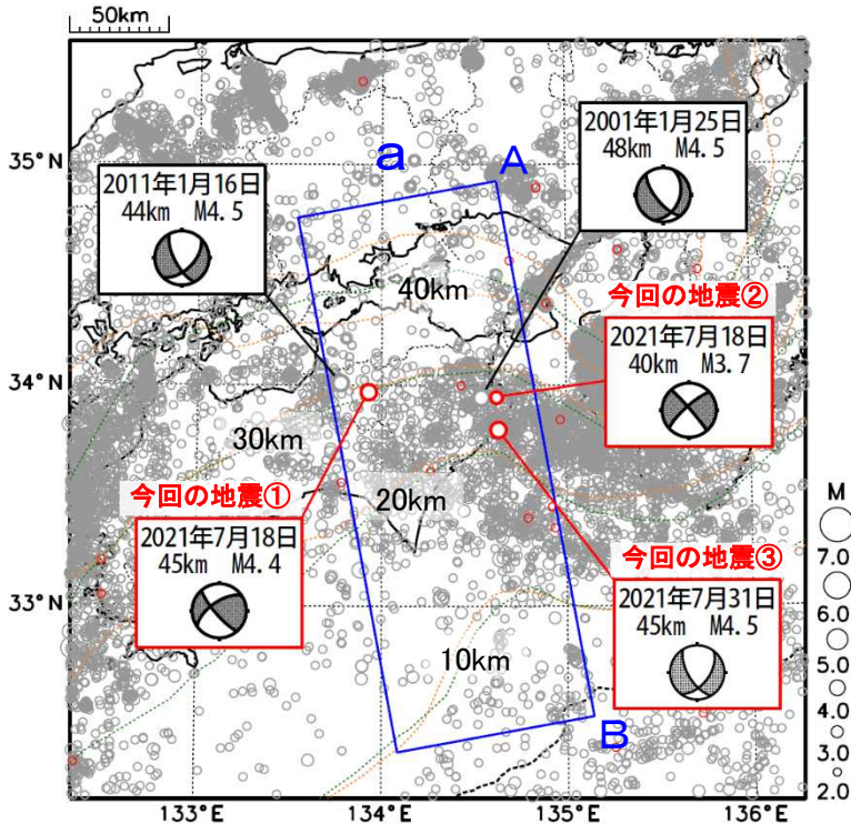
震央分布図 (1997年10月1日～2021年7月31日、 深さ0～90km、M≥2.0) 2021年7月18日以降の地震を赤く表示
