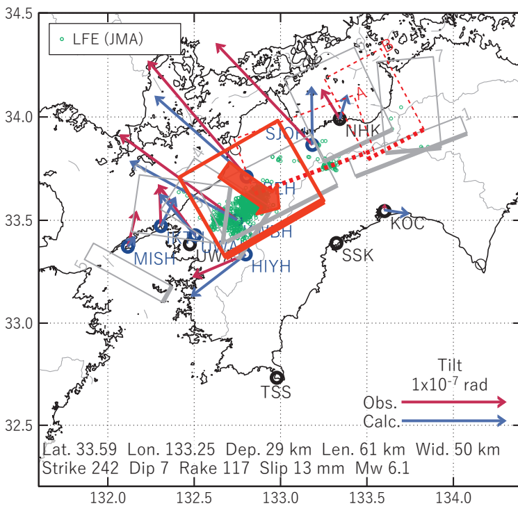
図6 2021/07/21PM-27の歪・傾斜変化 (図2,3[C]) を説明する断層モデル。
