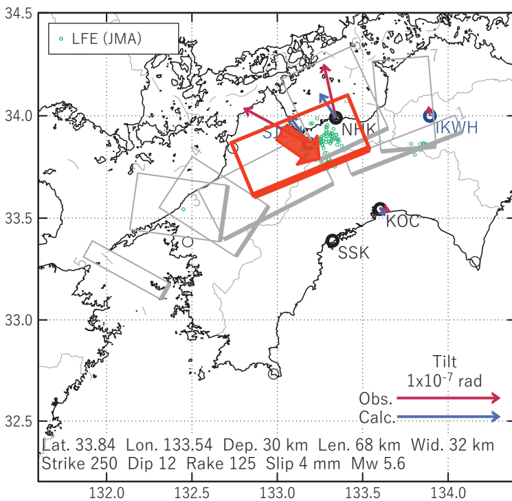
図4 2021/07/18-19AMの歪・傾斜変化 (図2,3[A]) を説明する断層モデル。
