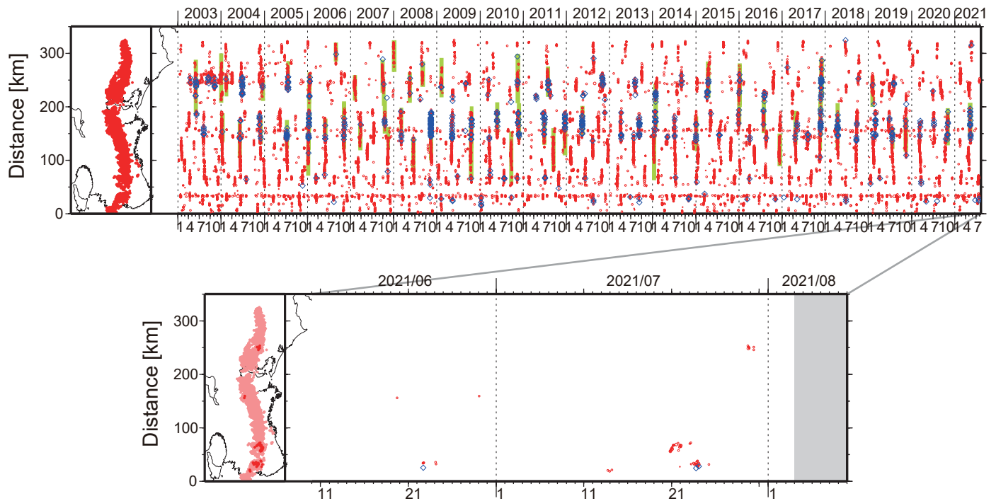
図1. 紀伊半島・東海地域における2003年1月～2021年8月3日までの深部低周波微動の時空間分布(上図). 赤丸はエンベロープ相関・振幅ハイブリッド法 (Maeda and Obara, 2009) およびクラスタ処理 (Obara et al., 2010) によって1時間毎に自動処理された微動分布の重心である. 青菱形は周期20秒に卓越する超低周波地震 (Ito et al., 2007) である. 黄緑色の太線はこれまでに検出された短期的スロースリップイベント (SSE) を示す. 下図は2021年7月を中心とした期間の拡大図である. 顕著な活動はとくにみられなかったものの, 7月20～22日頃および7月23～24日頃に, 奈良県南部から和歌山県中部において, それぞれ小規模な活動がみられた. 20～22日頃の活動は主に奈良県南部でみられ, 23～24日頃の活動は主に和歌山県中部でみられた. 7月13～14日頃には和歌山県中部において, 7月29～30日頃には愛知県東部において, それぞれごく小規模な活動がみられた.
