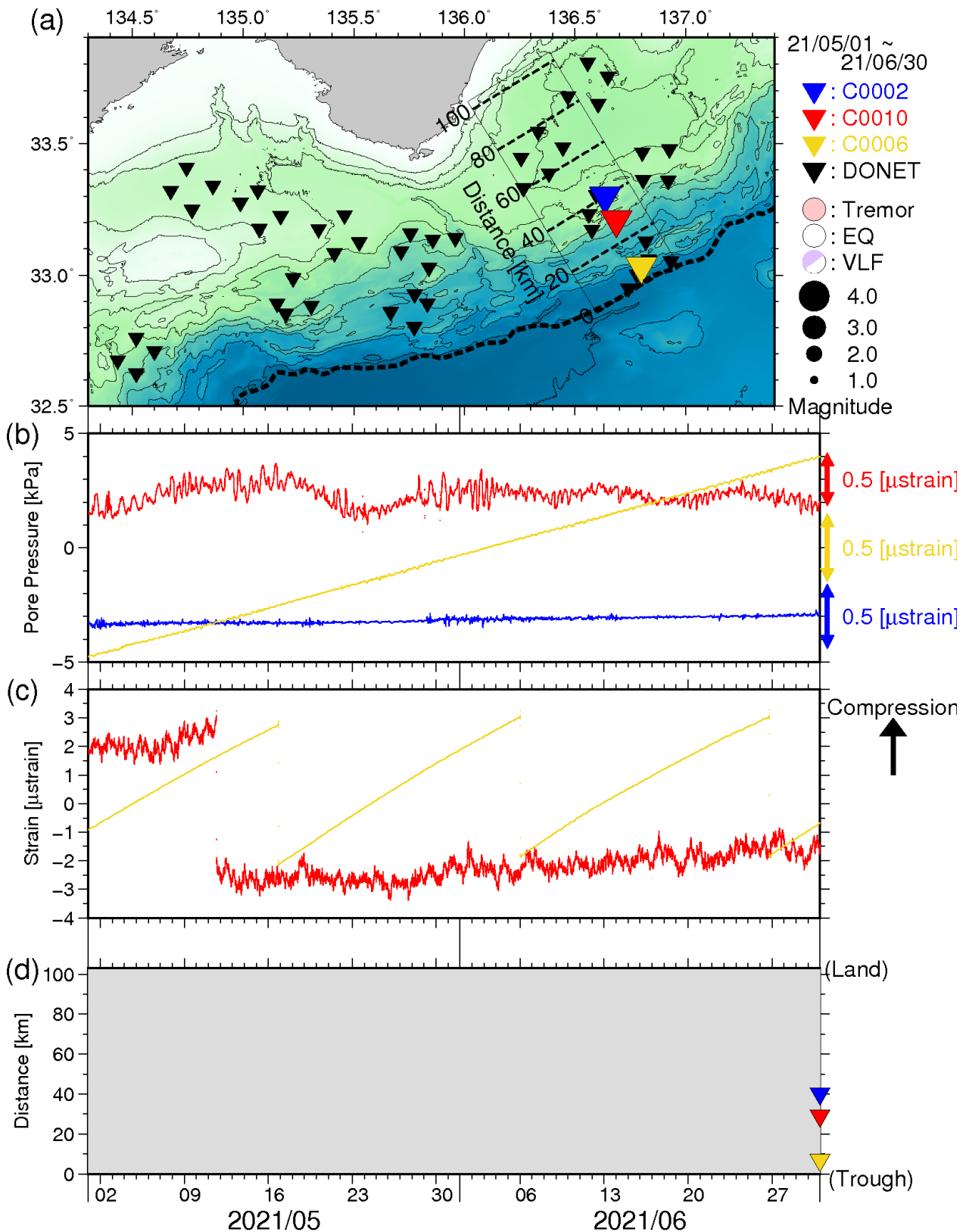
図3 直近2ヶ月間のSSE・低周波微動モニタリング(2021年5月1日~2021年6月30日)。(a) 低周波微動と通常地震の震央分布図(●:低周波微動、○:通常地震)。それぞれの震源深さが、0~15 km及び0~60 kmの範囲に決まったイベントのみを示す。▼、▼、▼、▼は、それぞれC0002・C0010・C0006・DONET観測点を示す。破線はトラフ軸を示す。(b) 長期孔内観測点における間隙水圧変化(—:C0002、—:C0010、—:C0006)。(c) 長期孔内観測点における体積歪変化(—:C0010、—:C0006)。(d) 低周波微動と通常地震の時空間分布。図3a中に実線で示した矩形領域内において発生したイベントについて示す。縦軸は、トラフ軸からの距離(km)を示す。
