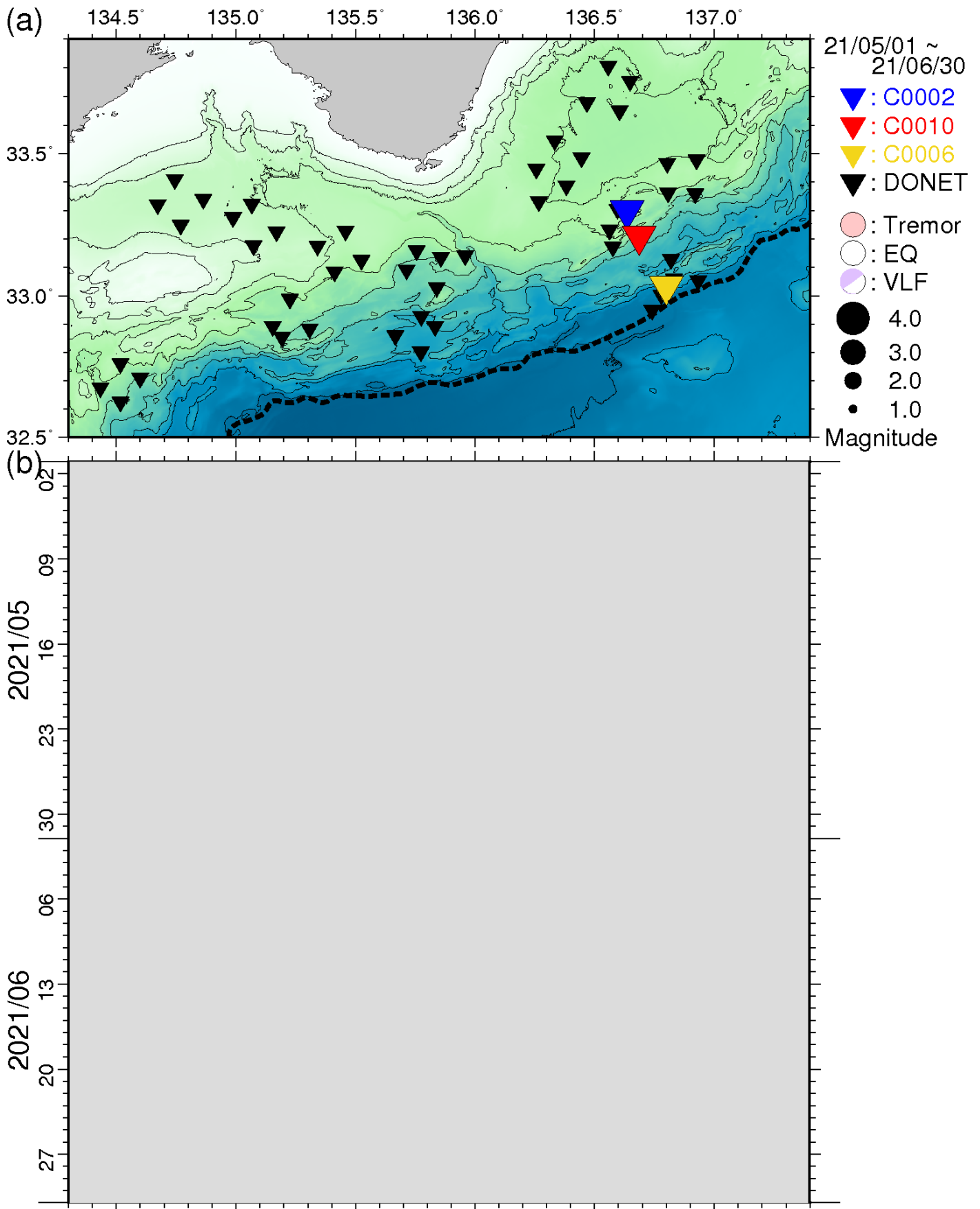
図5 直近2ヵ月間において熊野灘から室戸沖にて発生した低周波微動の時空間分布(2021年5月1日~2021年6月30日)。図3と同様のシンボルにて表示している。(a)低周波微動の震央分布図。(b)aに示した震央を経度方向へ投影した低周波微動の時空間分布図。2021年3月29日以降はネットワーク障害のため、微動と地震カタログの照合は未処理である。
