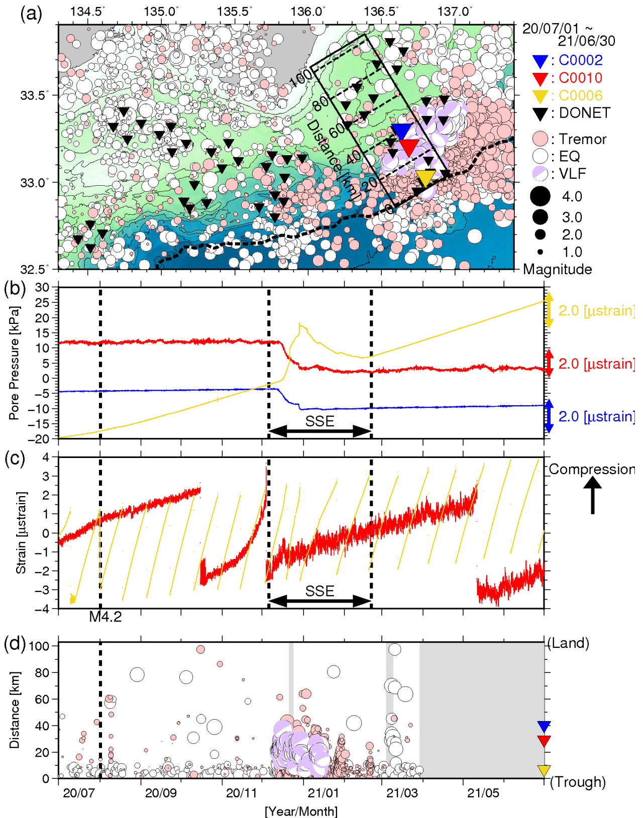
図4 直近1年間のSSE・低周波微動モニタリング(2020年7月1日~2021年6月30日)。図3と同様のシンボルにて表示している。(a)低周波微動の震央分布図。(b)間隙水圧変化。(c)体積歪変化。(d)低周波微動の時空間分布。超低周波地震のメカニズム解(●)についても低周波微動と同様に示す。体積歪変化は、基準値を超えると歪計内のバルブを開けてリセットするため、相対値のみを使用。なお、2020年12月7日~8日、21日~24日、2021年3月4日~9日はサーバ不具合・入替のため、3月29日以降はネットワーク障害のため、各期間においてデータ解析が未処理となっている。点線で示す地震情報については、図3および図6を参照。
