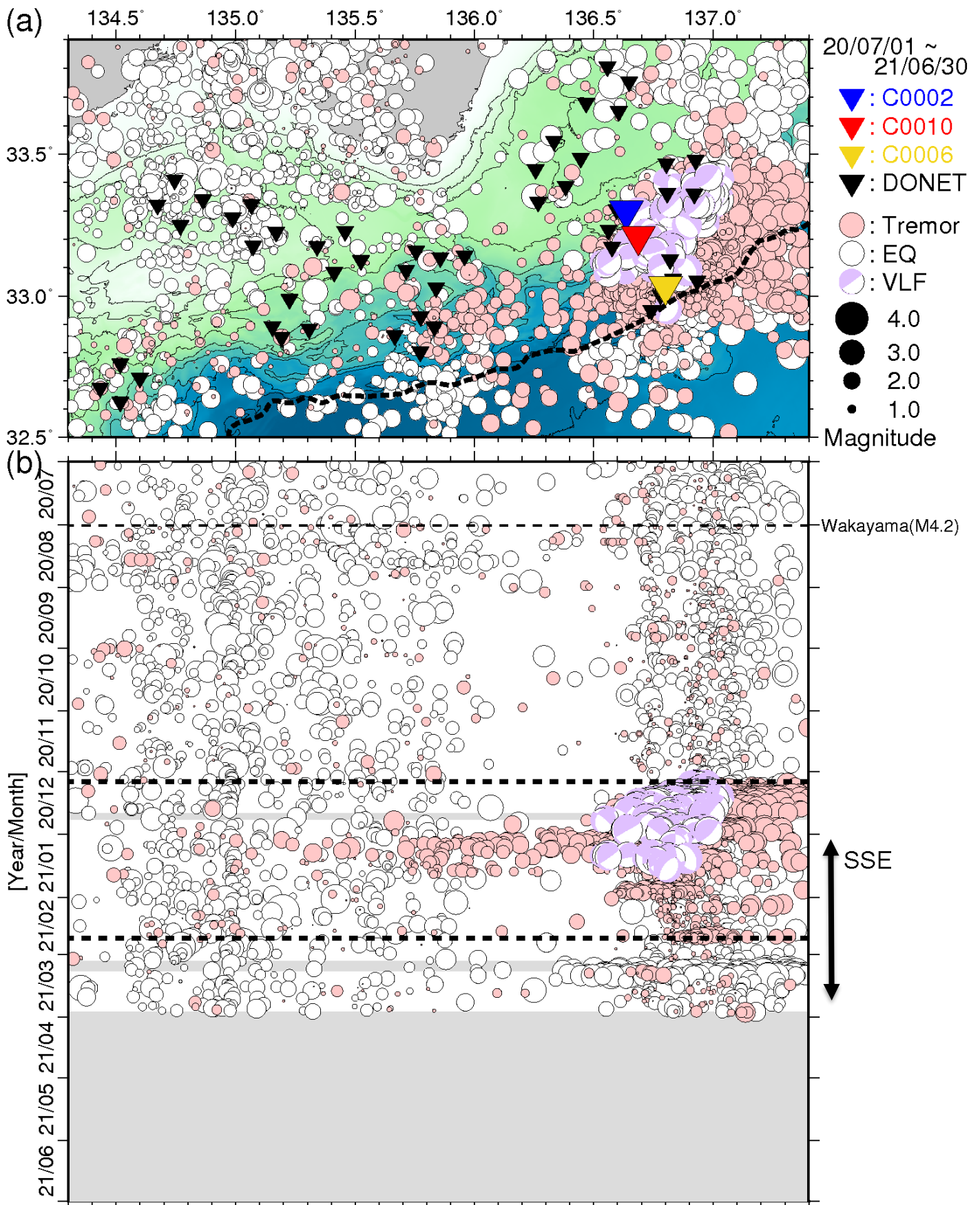
図6 直近1年間において熊野灘から室戸沖にて発生した低周波微動の時空間分布(2020年7月1日~2021年6月30日)。図3と同様のシンボルにて表示している。(a)低周波微動の震央分布図。(b)aに示した震央を経度方向へ投影した低周波微動の時空間分布図。超低周波地震のメカニズム解についても低周波微動と同様に示す。また、3月8日以降はエアガン信号が含まれていると考えられるが、これに関連する発振点情報が入手できていないため、未解析となっている。
