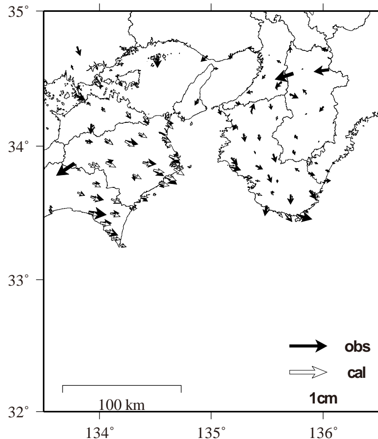
観測値（黒）と計算値（白）の比較 (2020/6/1 - 2021/6/8)
