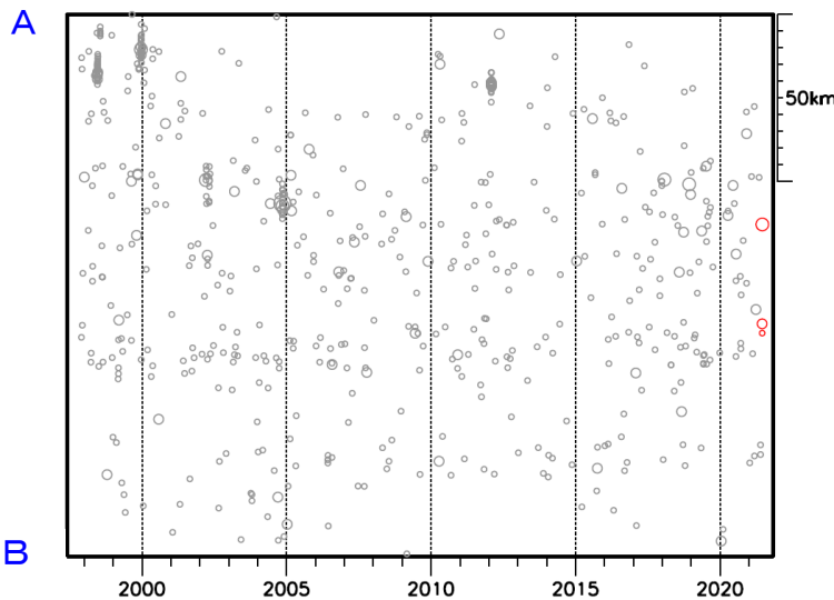
領域a内の時空間分布 (A-B投影)
