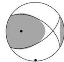
今回の地震の発震機構 (防災科研F-netによる) 深さ5km
