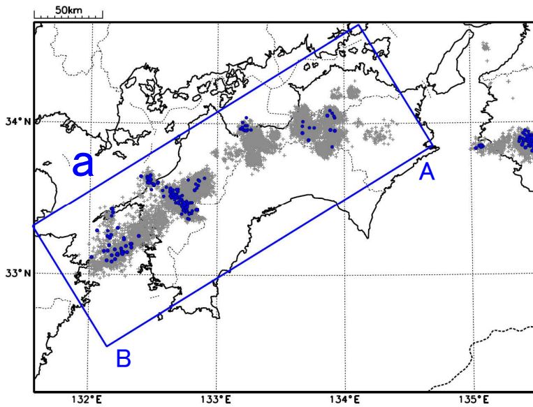
震央分布図(2018年4月1日~2021年6月24日、 深さ0~60km、Mすべて) 灰: 2018年4月1日~2021年6月3日、 青: 6月4日~6月24日
