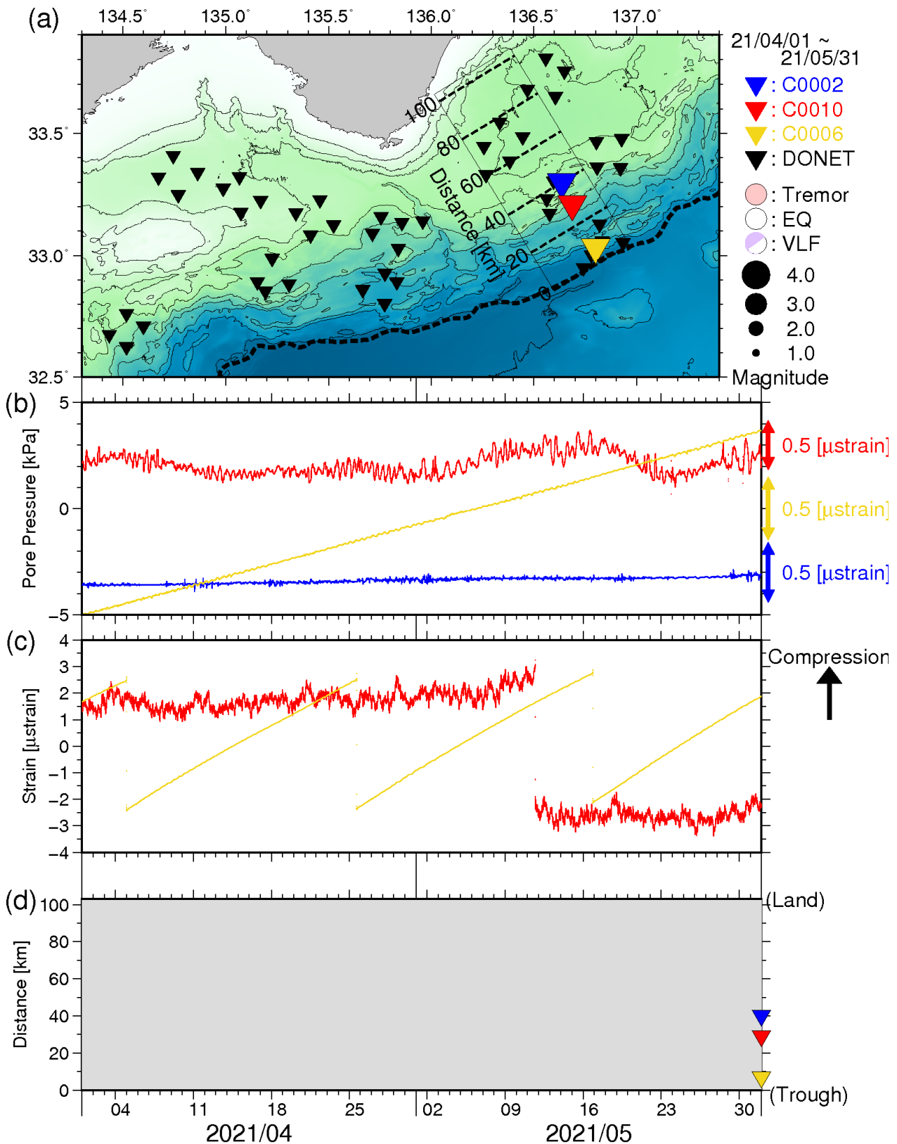
図3 直近2ヶ月間のSSE・低周波微動モニタリング(2021年4月1日~2021年5月31日)。(a) 低周波微動と通常地震の震央分布図(●:低周波微動、○:通常地震)。それぞれの震源深さが、0~15 km及び0~60 kmの範囲に決まったイベントのみを示す。▼、▼、▼、▼は、それぞれC0002・C0010・C0006・DONET観測点を示す。破線はトラフ軸を示す。(b) 長期孔内観測点における間隙水圧変化(—:C0002、—:C0010、—:C0006)。(c) 長期孔内観測点における体積歪変化(—:C0010、—:C0006)。(d) 低周波微動と通常地震の時空間分布。図3a中に実線で示した矩形領域内において発生したイベントについて示す。縦軸は、トラフ軸からの距離(km)を示す。
