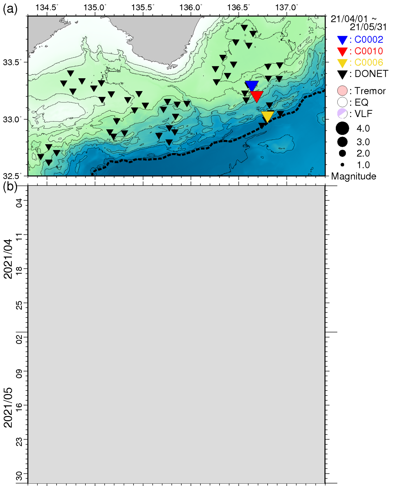
図5 直近2ヵ月間において熊野灘から室戸沖にて発生した低周波微動の時空間分布(2021年4月1日~2021年5月31日)。図3と同様のシンボルにて表示している。(a)低周波微動の震央分布図。(b)aに示した震央を経度方向へ投影した低周波微動の時空間分布図。2021年3月29日以降はネットワーク障害のため、微動と地震カタログの照合は未処理である。また、3月8日以降はエアガン信号が含まれていると考えられるが、これに関連する発振点情報が入手できていないため、未解析となっている。
