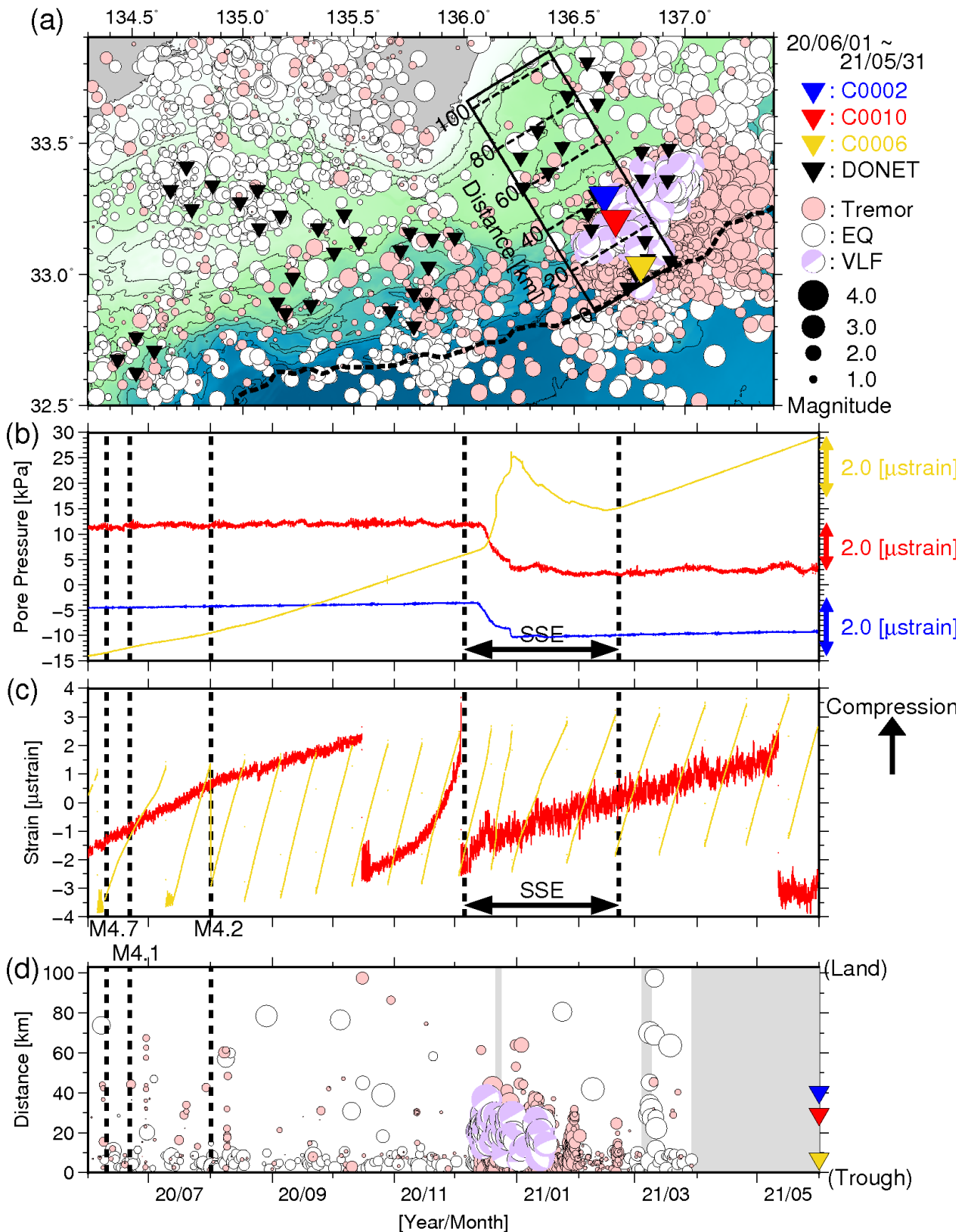
図4 直近1年間のSSE・低周波微動モニタリング(2020年6月1日~2021年5月31日)。図3と同様のシンボルにて表示している。(a)低周波微動の震央分布図。(b)間隙水圧変化。(c)体積歪変化。(d)低周波微動の時空間分布。超低周波地震のメカニズム解(●)についても低周波微動と同様に示す。体積歪変化は、基準値を超えると歪計内のバルブを開けてリセットするため、相対値のみを使用。なお、2020年6月3日、12月7日~8日、21日~24日、2021年3月4日~9日はサーバ不具合・入替のため、3月29日以降はネットワーク障害のため、各期間においてデータ解析が未処理となっている。点線で示す地震情報については、図3および図6を参照。
