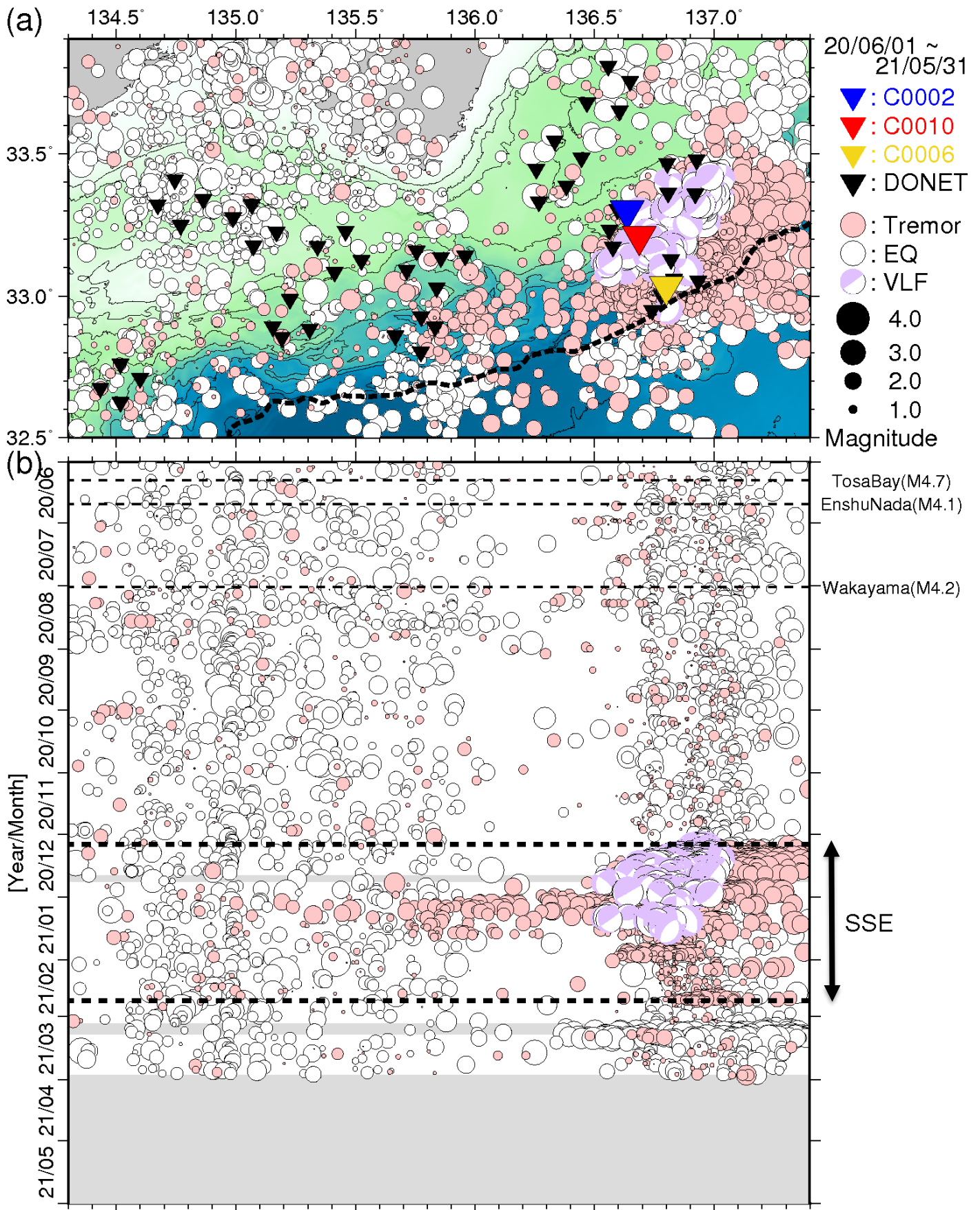
図6 直近1年間において熊野灘から室戸沖にて発生した低周波微動の時空間分布(2020年6月1日~2021年5月31日)。図3と同様のシンボルにて表示している。(a)低周波微動の震央分布図。(b)aに示した震央を経度方向へ投影した低周波微動の時空間分布図。超低周波地震のメカニズム解についても低周波微動と同様に示す。
