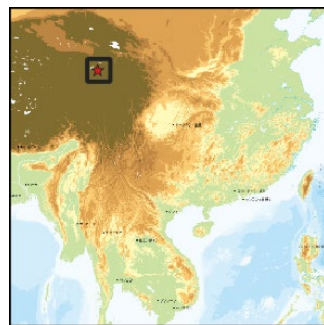
図4. 解析エリア
