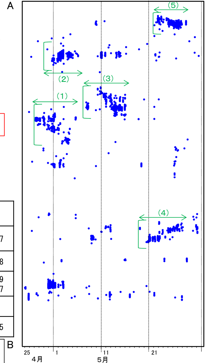
領域a(点線矩形)内の深部低周波地震(微動)の時空間分布図(A-B投影)
