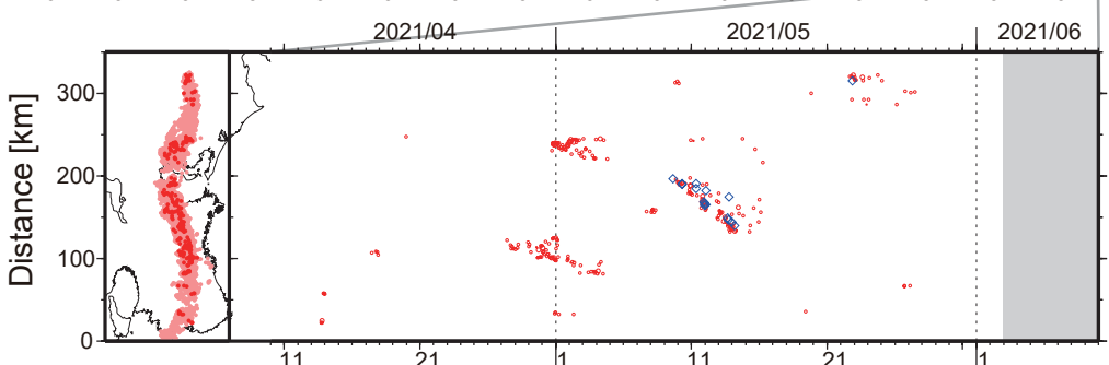
図1. 紀伊半島・東海地域における2003年1月～2021年6月2日までの深部低周波微動の時空間分布(上図). 赤丸はエンベロープ相関・振幅ハイブリッド法 (Maeda and Obara, 2009) およびクラスタ処理 (Obara et al., 2010) によって1時間毎に自動処理された微動
