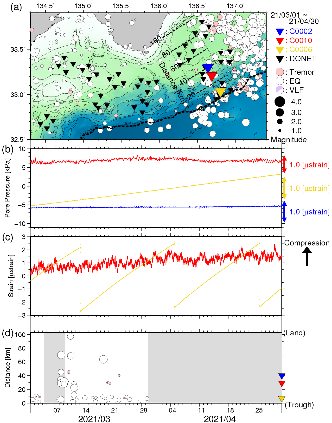
図3 直近2ヶ月間のSSE・低周波微動モニタリング(2021年3月1日~2021年4月30日)。(a) 低周波微動と通常地震の震央分布図(●:低周波微動、○:通常地震)。それぞれの震源深さが、0~15 km及び0~60 kmの範囲に決まったイベントのみを示す。▼▼▼は、それぞれC0002・C0010・C0006・DONET観測点を示す。破線はトラフ軸を示す。(b) 長期孔内観測点における間隙水圧変化(—:C0002、—:C0010、—:C0006)。(c) 長期孔内観測点における体積歪変化(—:C0010、—:C0006)。(d) 低周波微動と通常地震の時空間分布。図3a中に実線で示した矩形領域内において発生したイベントについて示す。縦軸は、トラフ軸からの距離(km)を示す。
