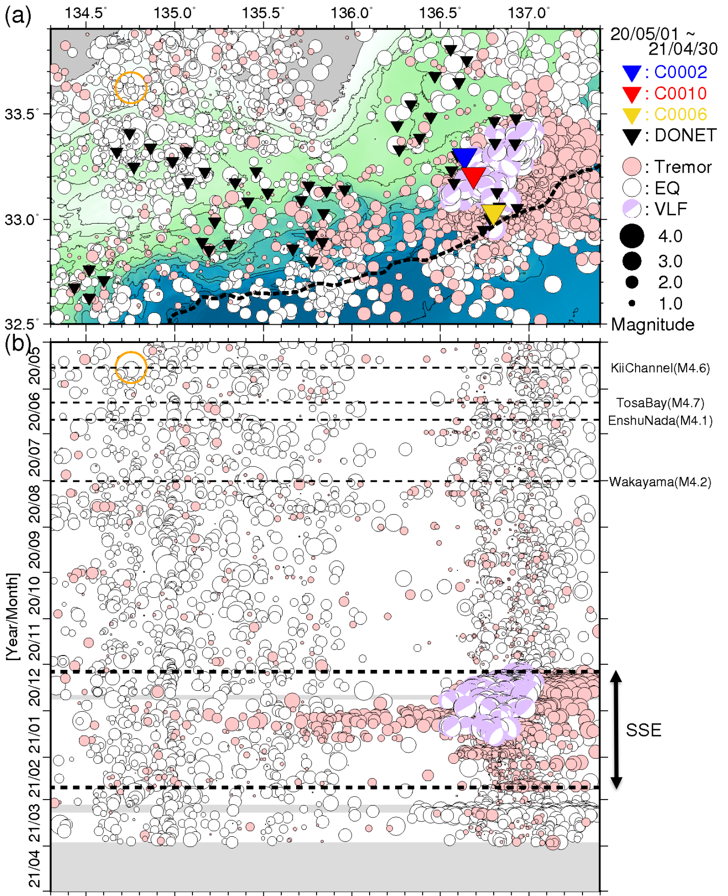
図6 直近1年間において熊野灘から室戸沖にて発生した低周波微動の時空間分布(2020年5月1日~2021年4月30日)。図3と同様のシンボルにて表示している。(a)低周波微動の震央分布図。(b)aに示した震央を経度方向へ投影した低周波微動の時空間分布図。超低周波地震のメカニズム解についても低周波微動と同様に示す。○は2020年5月17日に発生した紀伊水道地震を示す。
