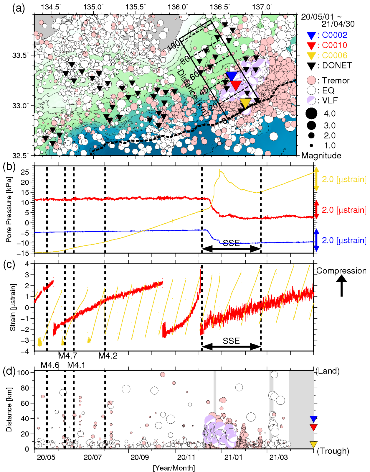
図4 直近1年間のSSE・低周波微動モニタリング(2020年5月1日~2021年4月30日)。図3と同様のシンボルにて表示している。(a)低周波微動の震央分布図。(b)間隙水圧変化。(c)体積歪変化。(d)低周波微動の時空間分布。超低周波地震のメカニズム解(●)についても低周波微動と同様に示す。体積歪変化は、基準値を超えると歪計内のバルブを開けてリセットするため、相対値のみを使用。なお、2020年5月10日~12日および6月3日、12月7日~8日、21日~24日、2021年3月4日~9日はサーバ不具合・入替のため、3月29日以降はネットワーク障害のため、各期間においてデータ解析が未処理となっている。点線で示す地震情報については、図3および図6を参照。
