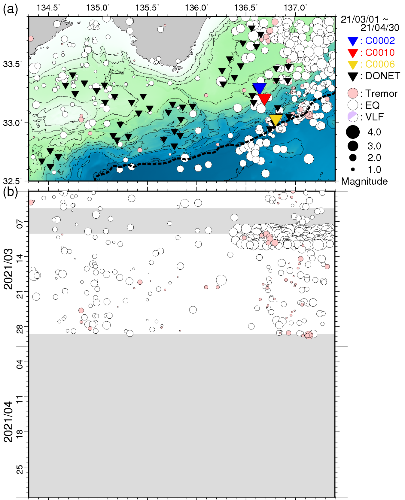
図5 直近2ヵ月間において熊野灘から室戸沖にて発生した低周波微動の時空間分布(2021年3月1日~2021年4月30日)。図3と同様のシンボルにて表示している。(a)低周波微動の震央分布図。(b)aに示した震央を経度方向へ投影した低周波微動の時空間分布図。2021年3月4日~9日はサーバ不具合のため、3月29日以降はネットワーク障害のため、微動と地震カタログの照合は未処理である。また、3月8日以降はエアガン信号が含まれていると考えられるが、これに関連する発振点情報が入手できていないため、未解析となっている。
