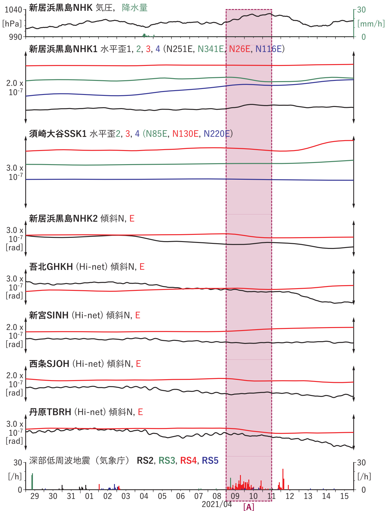
図2 歪・傾斜の時間変化 (2021/03/29 00:00 - 2021/04/16 00:00 (JST))
