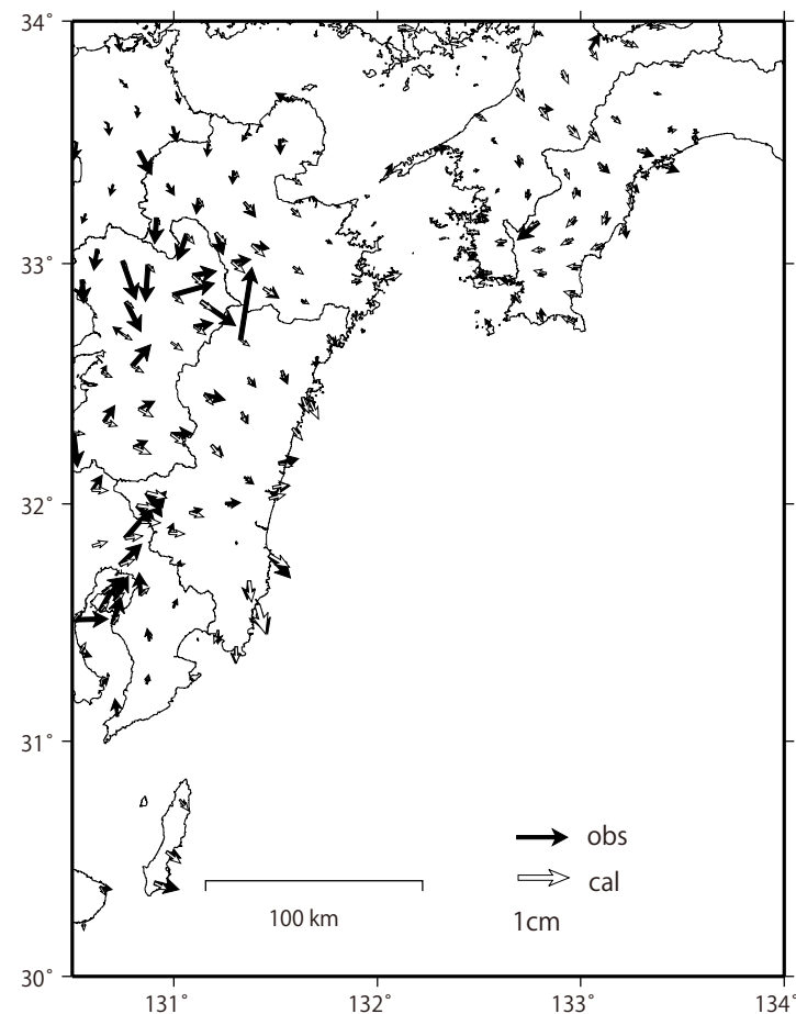
観測値(黒)と計算値(白)の比較 (2020/6/1 - 2021/3/11)
