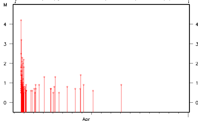
2021年4月13日～30日、 M \geq 0.5 、M-T図のみ
