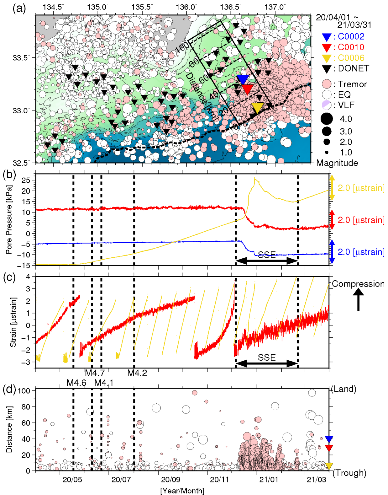
図4 直近1年間のSSE・低周波微動モニタリング(2020年4月1日~2021年3月31日)。図3と同様のシンボルにて表示している。(a)低周波微動の震央分布図。(b)間隙水圧変化。(c)体積歪変化。(d)低周波微動の時空間分布。超低周波地震のメカニズム解(●)についても低周波微動と同様に示す。体積歪変化は、基準値を超えると歪計内のバルブを開けてリセットするため、相対値のみを使用。なお、2020年4月16日は測器の状態確認や再起動のため、2020年5月10日~12日および6月3日、12月7日~8日、21日~24日、2021年3月4日~9日はサーバ不具合・入替のため、3月29日以降はネットワーク障害のため、各期間において一部データが欠測している。点線で示す地震情報については、図3および図6を参照。
