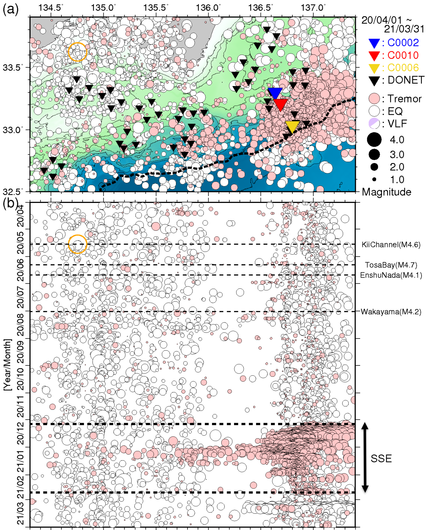
図6 直近1年間において熊野灘から室戸沖にて発生した低周波微動の時空間分布(2020年4月1日~2021年3月31日)。図3と同様のシンボルにて表示している。(a)低周波微動の震央分布図。(b)aに示した震央を経度方向へ投影した低周波微動の時空間分布図。超低周波地震のメカニズム解についても低周波微動と同様に示す。○は2020年5月17日に発生した紀伊水道地震を示す。
