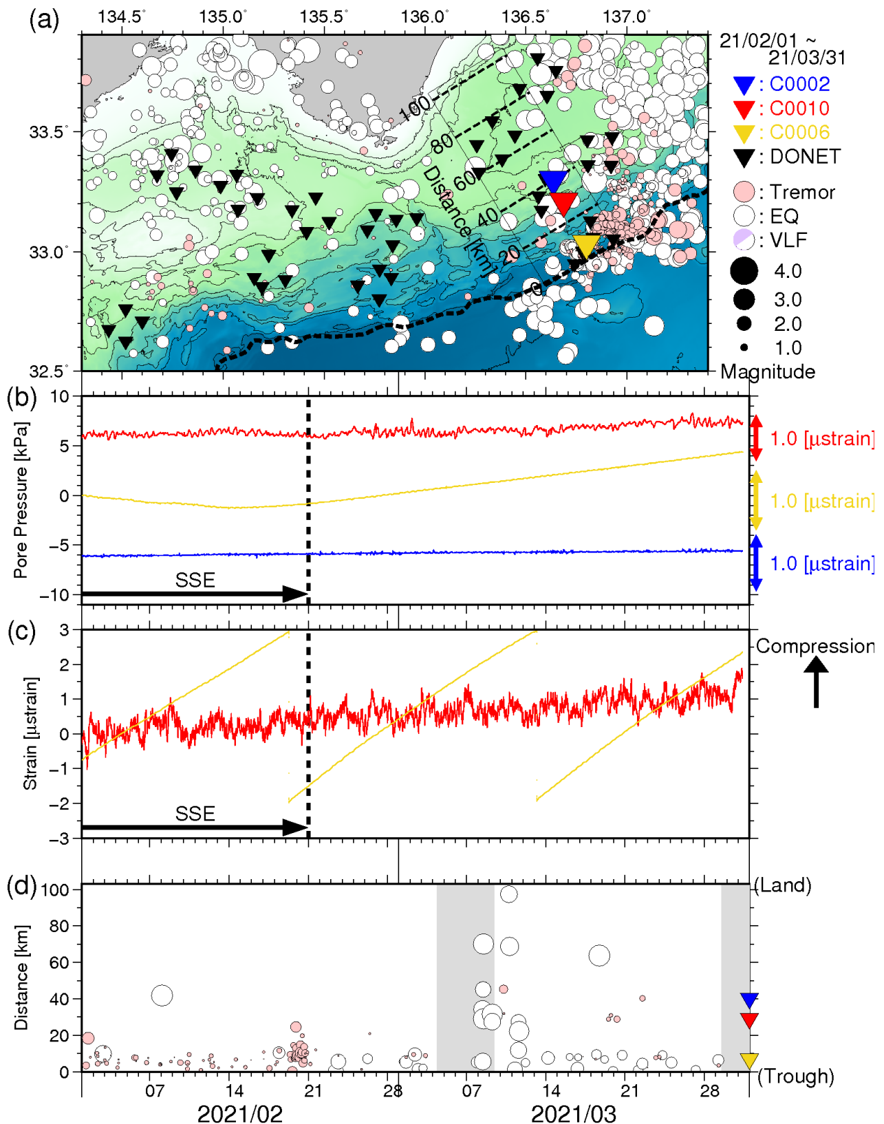
図3 直近2ヶ月間のSSE・低周波微動モニタリング(2021年2月1日~2021年3月31日)。(a)低周波微動と通常の地震の震央分布図(●:低周波微動、○:通常の地震)。それぞれの震源深さが、0~15 km及び0~60 kmの範囲に決まったイベントのみを示す。▼▼▼は、それぞれC0002・C0010・C0006・DONET観測点を示す。破線はトラフ軸を示す。(b)長期孔内観測点における間隙水圧変化(—:C0002、—:C0010、—:C0006)。(c)長期孔内観測点における体積歪変化(—:C0010、—:C0006)。(d)低周波微動と通常地震の時空間分布。図3a中に実線で示した矩形領域内において発生したイベントについて示す。縦軸は、トラフ軸からの距離(km)を示す。
