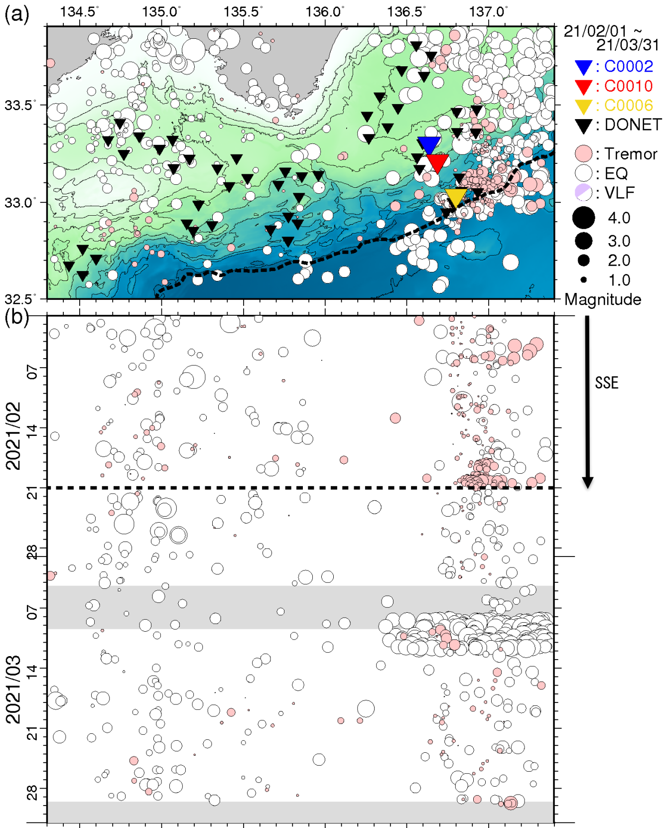
図5 直近2ヵ月間において熊野灘から室戸沖にて発生した低周波微動の時空間分布(2021年2月1日~2021年3月31日)。図3と同様のシンボルにて表示している。(a)低周波微動の震央分布図。(b)aに示した震央を経度方向へ投影した低周波微動の時空間分布図。2021年3月4日~9日はサーバ不具合のため、3月29日以降はネットワーク障害のため、微動と地震カタログの照合は未処理である。また、3月8日以降はエアガン信号が含まれていると考えられるが、これに関連する発振点情報が入手できていないため、未解析となっている。
