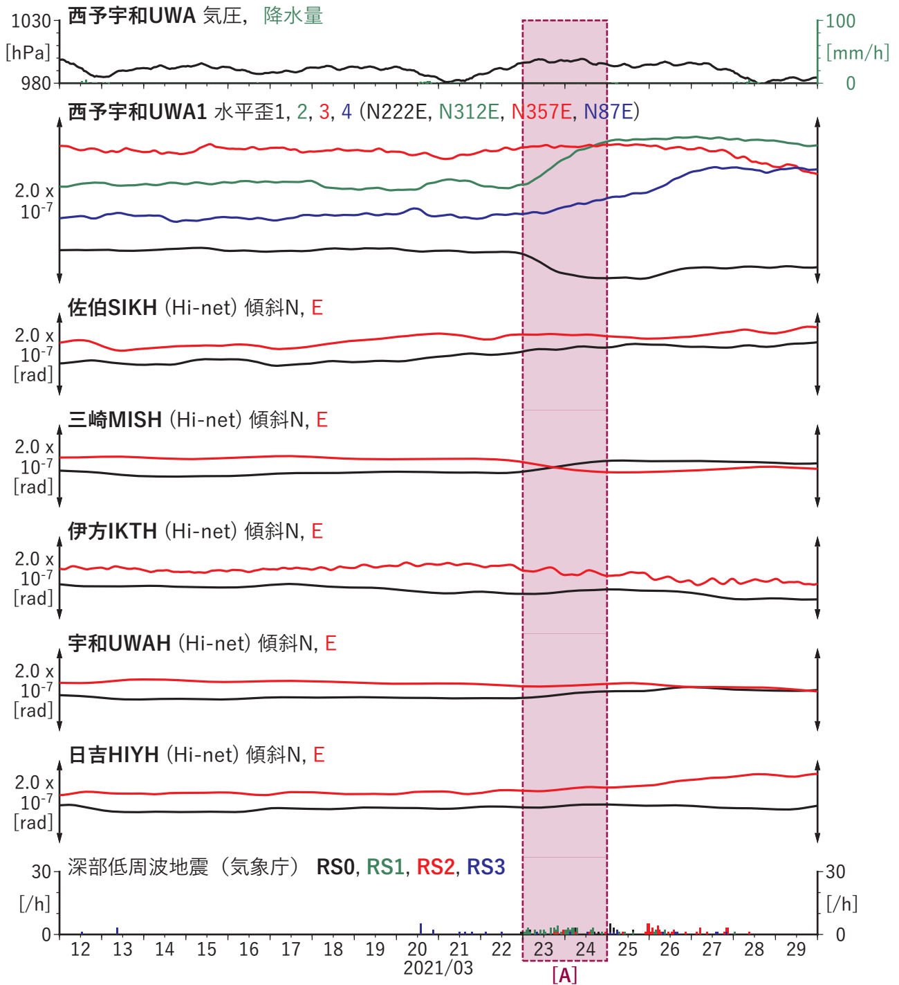
図5 歪・傾斜の時間変化 (2021/03/12 00:00 - 2021/03/30 00:00 (JST))
