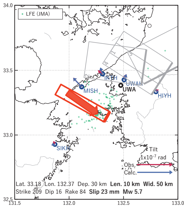
図6 2021/03/23 - 24 の歪・傾斜変化 (図5[A]) を説明する断層モデル。
