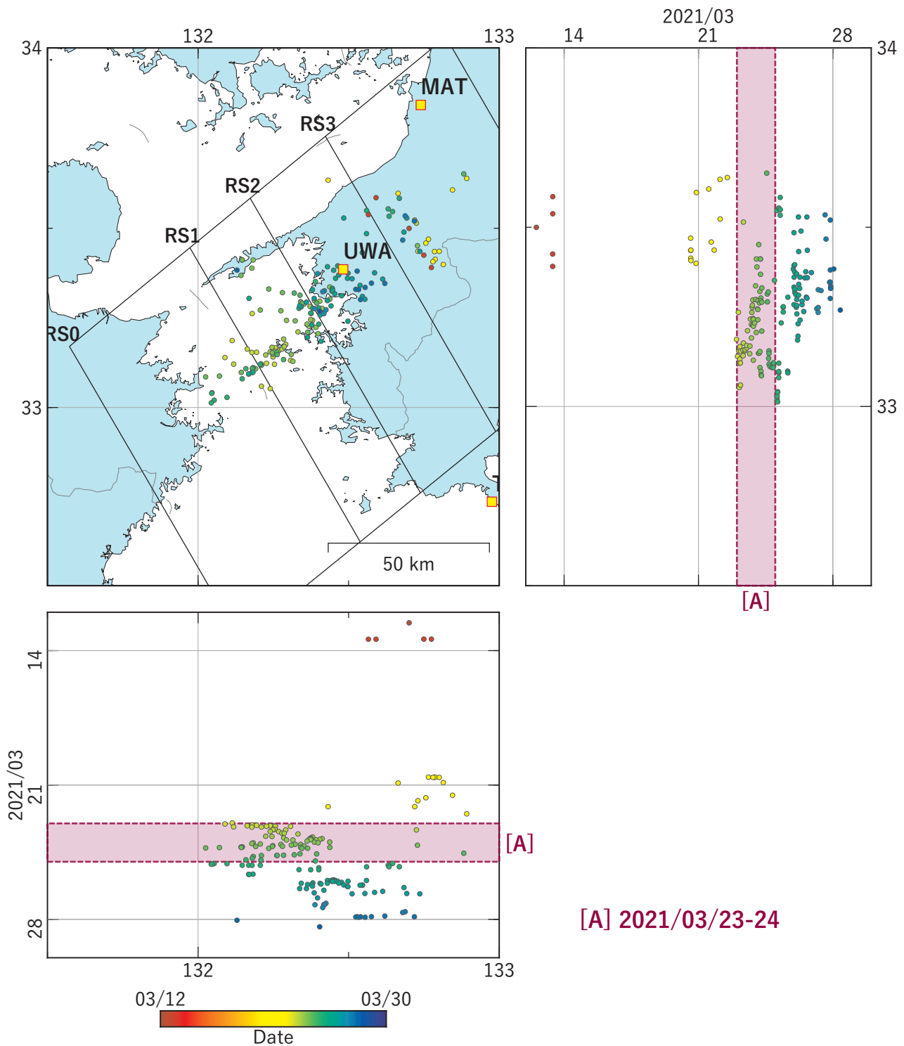
図4 四国における深部低周波地震の時空間分布図。 (2021/03/12 00:00 - 2021/03/30 00:00 (JST)) 気象庁カタログによる。
