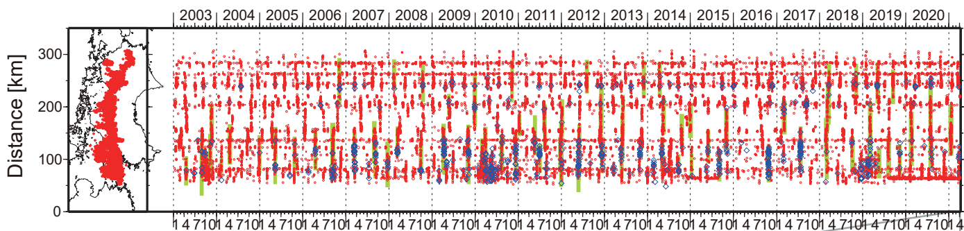
図1. 四国における2003年1月～2021年4月4日までの深部低周波微動の時空間分布(上図). 赤丸はエンベロープ相関・振幅ハイブリッド法 (Maeda and Obara, 2009) およびクラスタ処理 (Obara et al., 2010) によって1時間毎に自動処理された微動分布の重心である. 青菱形は周期20秒
