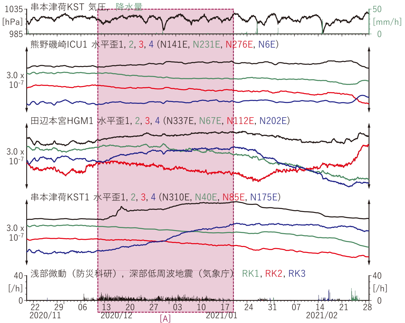
図10 紀伊半島における歪観測結果 (2020/11/20 00:00 - 2021/03/01 00:00 (JST)). 微動データは防災科学技術研究所提供. 歪データは気圧応答・潮位偏差応答・1次トレンド除去. 潮位偏差データは気象庁提供.
