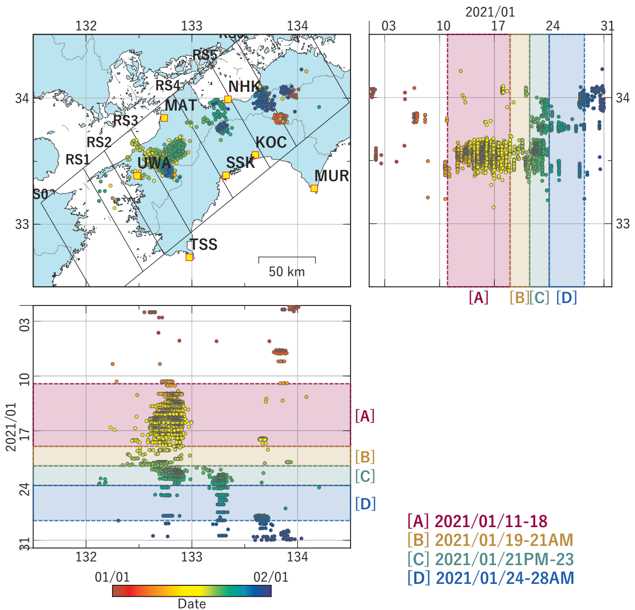
図1 四国地方における深部低周波地震の時空間分布図。 (2021/01/01 00:00 - 2021/02/01 00:00 (JST)) 気象庁カタログによる。
