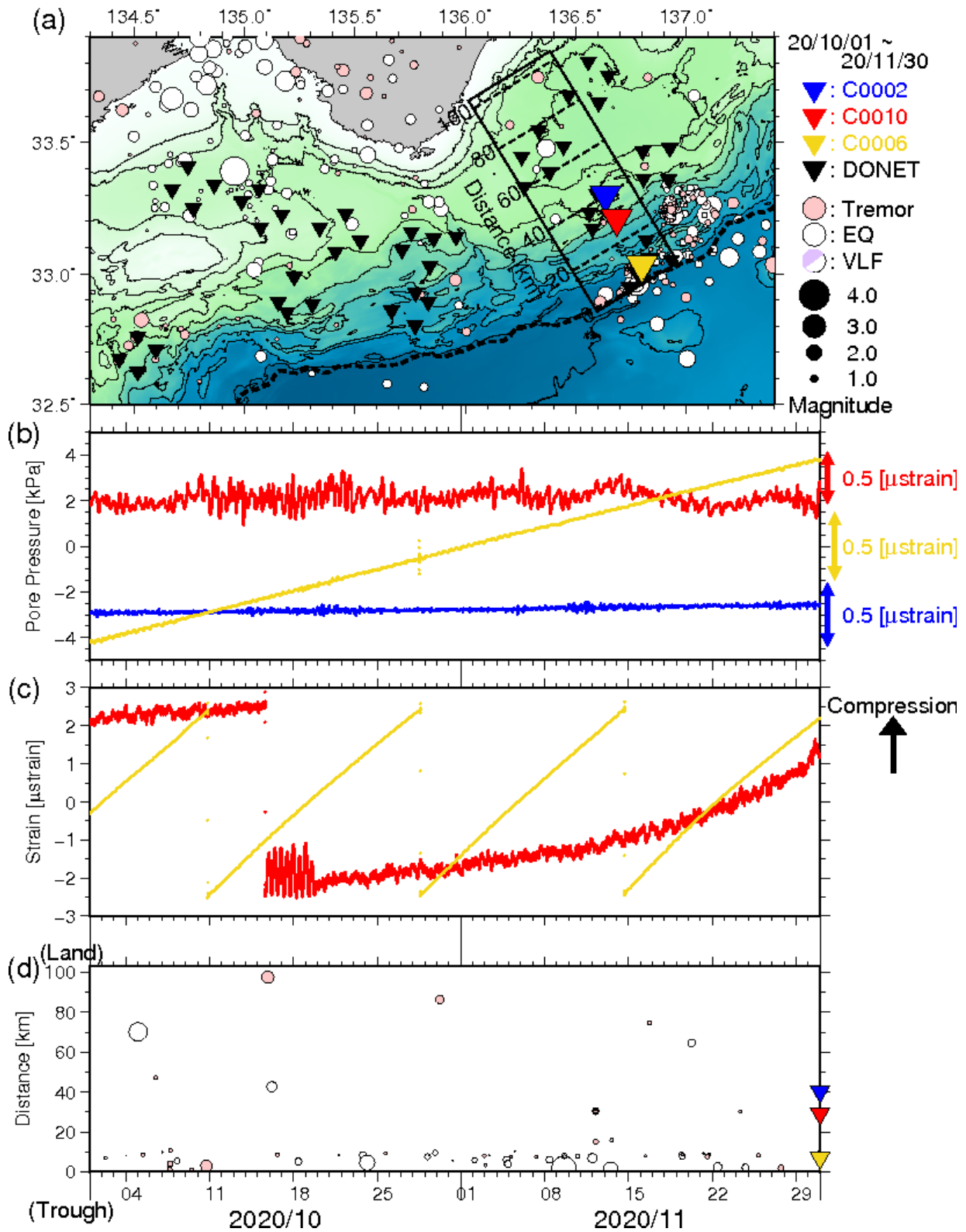
図3 直近2ヶ月間のSSE・低周波微動モニタリング(2020年10月1日~2020年11月30日)。 (a) 低周波微動と通常の地震の震央分布図(●:低周波微動、○:通常の地震)。それぞれの震源深さが、0~15 km及び0~60 kmの範囲に決まったイベントのみを示す。●は、超低周波地震のメカニズム解を示す。▼ ▼ ▼ ▼は、それぞれC0002・C0010・C0006・DONET観測点を示す。破線はトラフ軸を示す。(b) 長期孔内観測点における間隙水圧変化(—:C0002、—:C0010、—:C0006)。(c) 長期孔内観測点における体積歪変化(—:C0010、—:C0006)。(d) 低周波微動と通常地震の時空間分布。図3a中に実線で示した矩形領域内において発生したイベントについて示す。縦軸は、トラフ軸からの距離(km)を示す。
