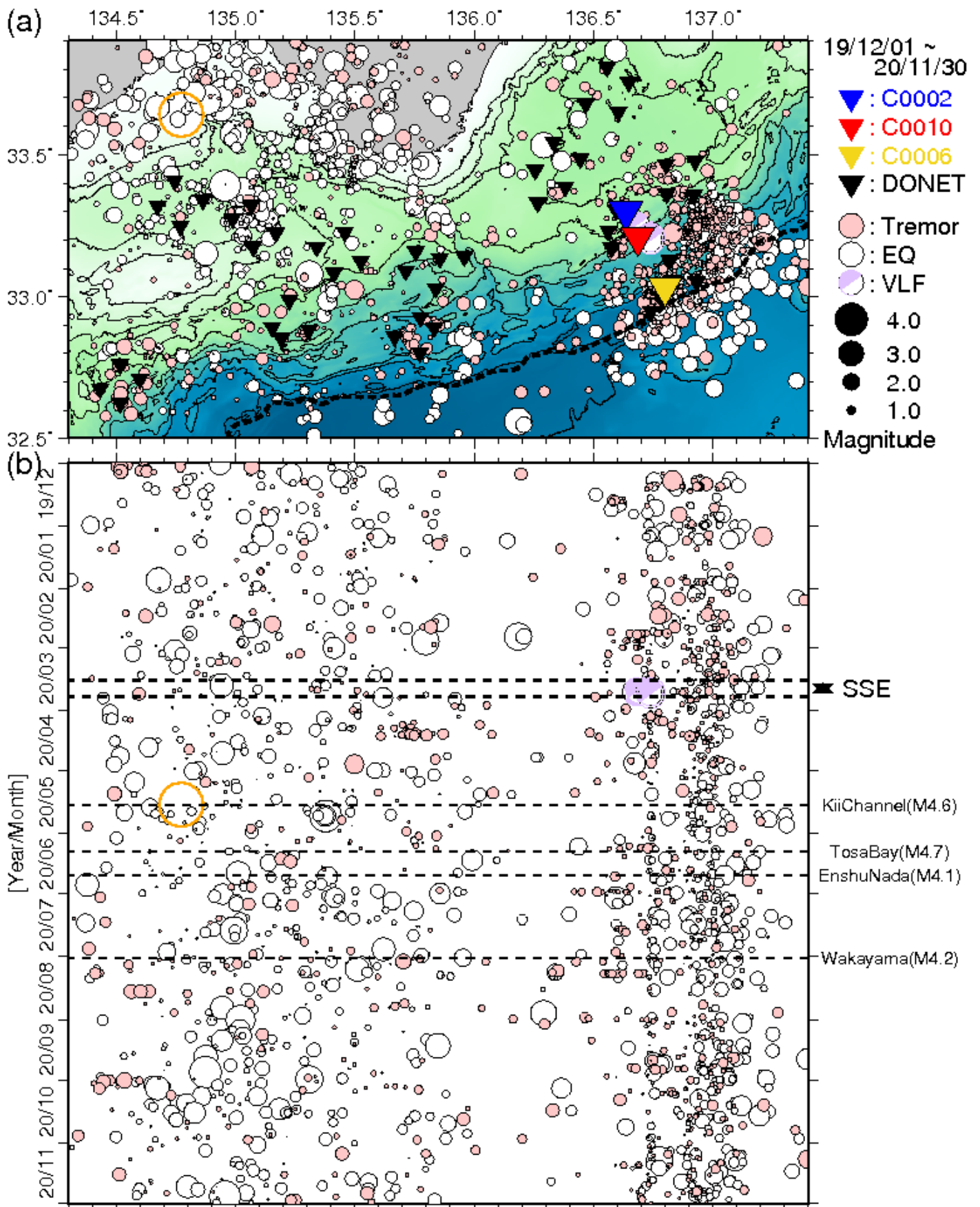
図6 直近1年間において熊野灘から室戸沖にて発生した低周波微動の時空間分布(2019年12月1日~2020年11月30日)。図3と同様のシンボルにて表示している。(a)低周波微動の震央分布図。(b)aに示した震央を経度方向へ投影した低周波微動の時空間分布図。超低周波地震のメカニズム解についても低周波微動と同様に示す。○は2020年5月17日に発生した紀伊水道地震を示す。
