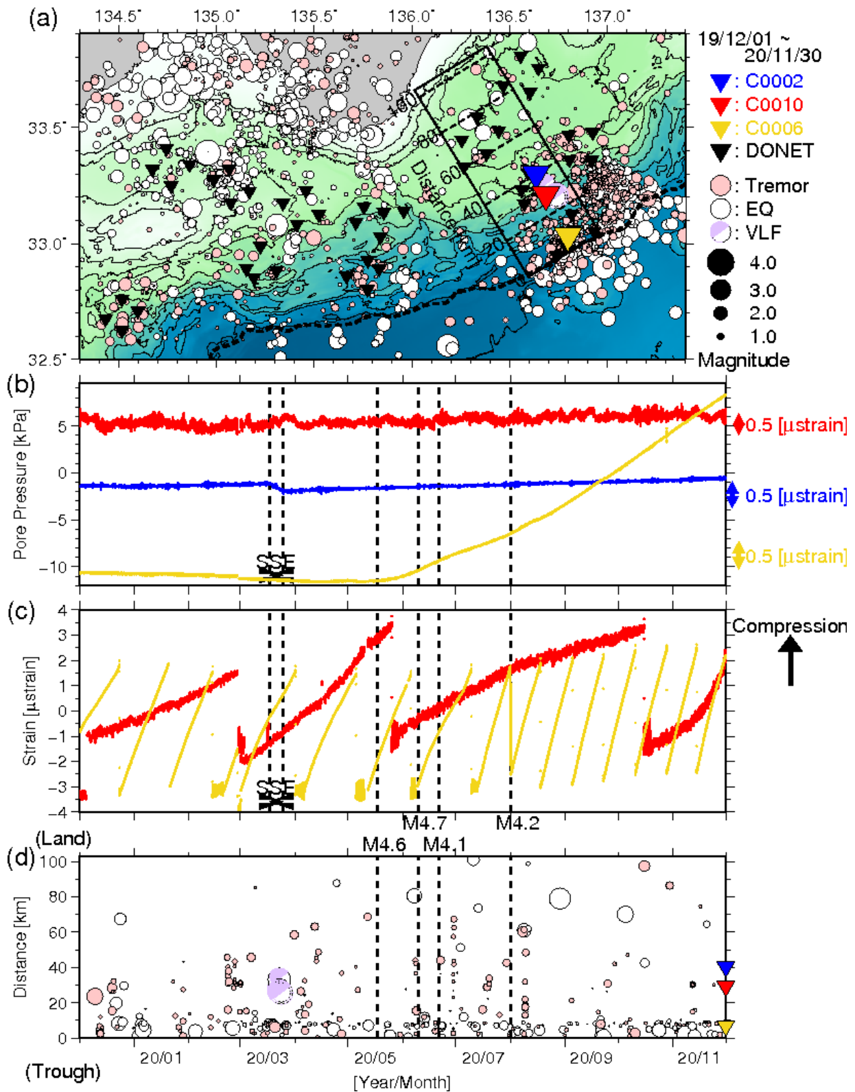
図4 直近1年間のSSE・低周波微動モニタリング（2019年12月1日～2020年11月30日）。図3と同様のシンボルにて表示している。(a) 低周波微動の震央分布図。(b) 間隙水圧変化。(c) 体積歪変化。(d) 低周波微動の時空間分布。超低周波地震のメカニズム解についても低周波微動と同様に示す。体積歪変化は、基準値を超えると歪計内のバルブを開けてリセットするため、相対値のみを使用。なお、2020年2月28日はノードA交換に伴うC0010水圧計の不具合のため、2020年3月2日、16日および4月16日は測器の状態確認や再起動のため、2020年5月10日～12日および6月3日はサーバの不具合のため、各期間において一部データが欠測している。点線で示す地震情報については、図3および図6を参照。
