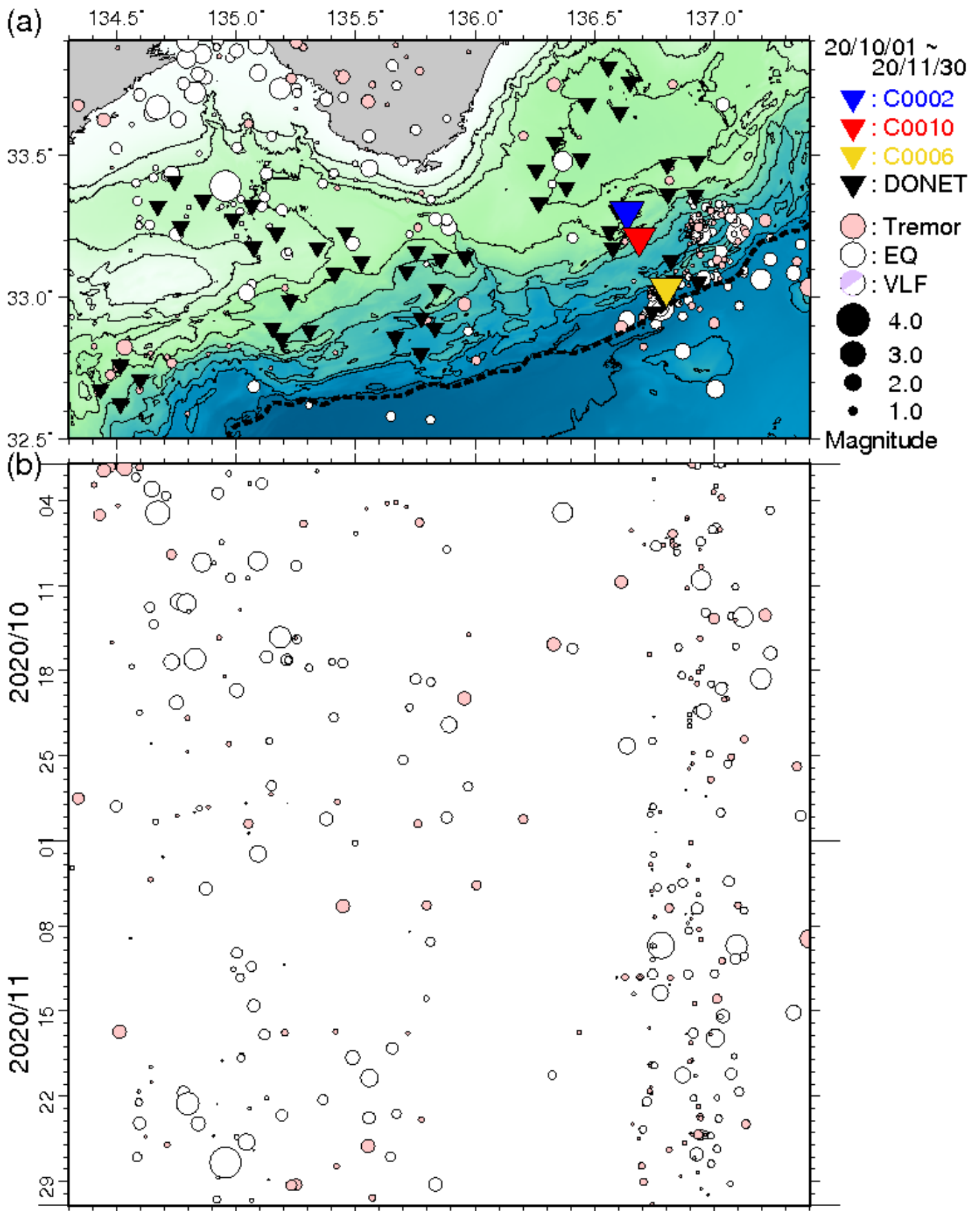
図5 直近2ヵ月間において熊野灘から室戸沖にて発生した低周波微動の時空間分布（2020年10月1日～2020年11月30日）。図3と同様のシンボルにて表示している。(a) 低周波微動の震央分布図。(b) aに示した震央を経度方向へ投影した低周波微動の時空間分布図。
