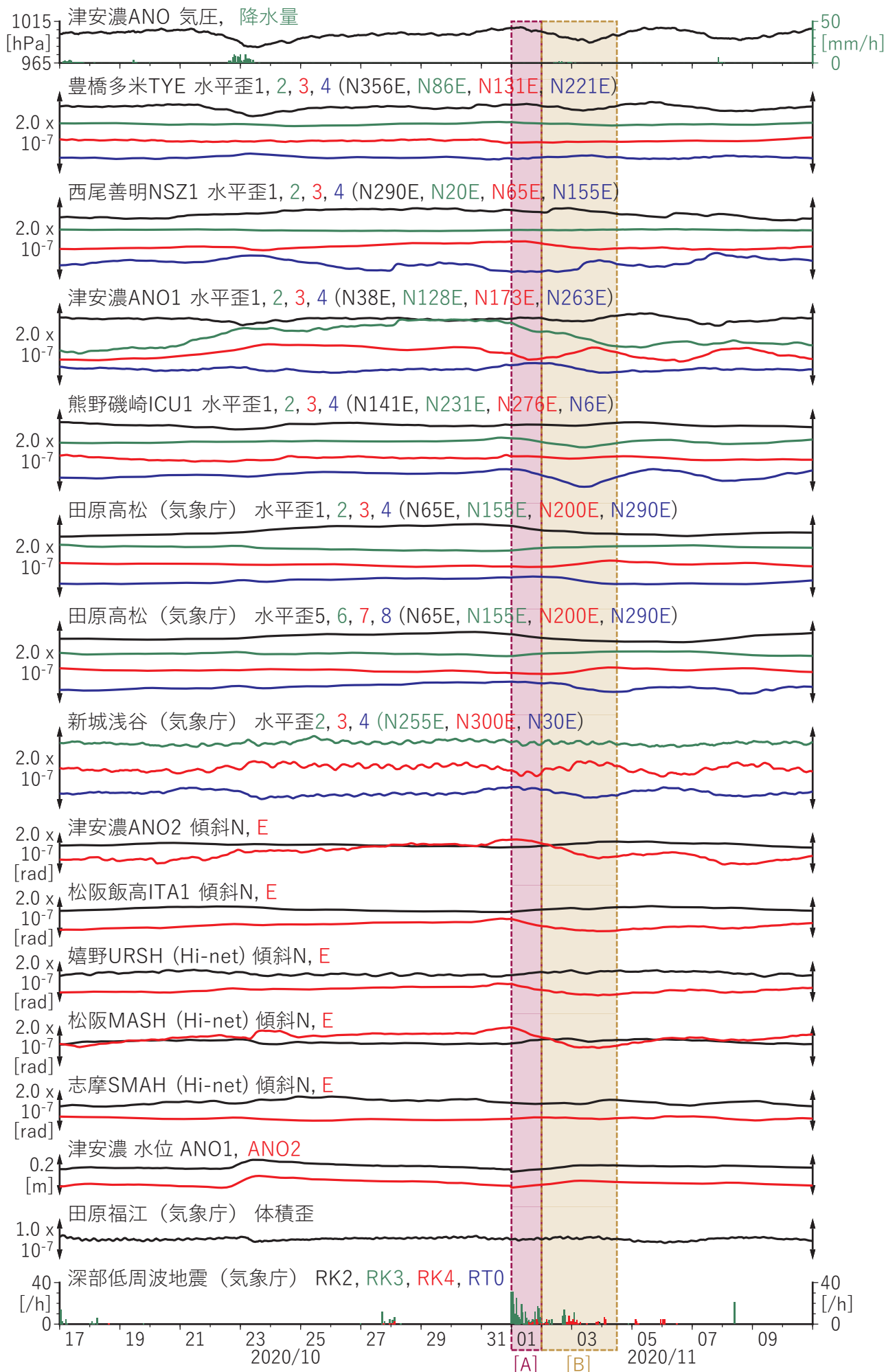
図2 紀伊半島～東海地方における歪・傾斜・地下水観測結果 (2020/10/17 00:00 - 2020/11/11 00:00 (JST)) 産業技術総合研究所 資料
