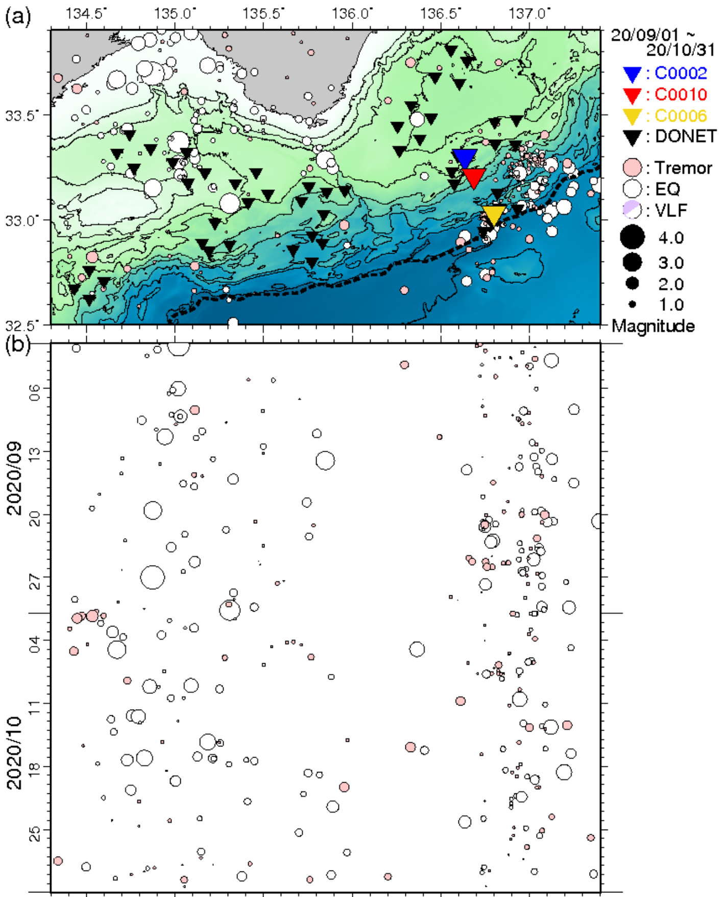
図5 直近2ヵ月間において熊野灘から室戸沖にて発生した低周波微動の時空間分布(2020年9月1日~2020年10月31日)。図3と同様のシンボルにて表示している。(a)低周波微動の震央分布図。(b)aに示した震央を経度方向へ投影した低周波微動の時空間分布図。
