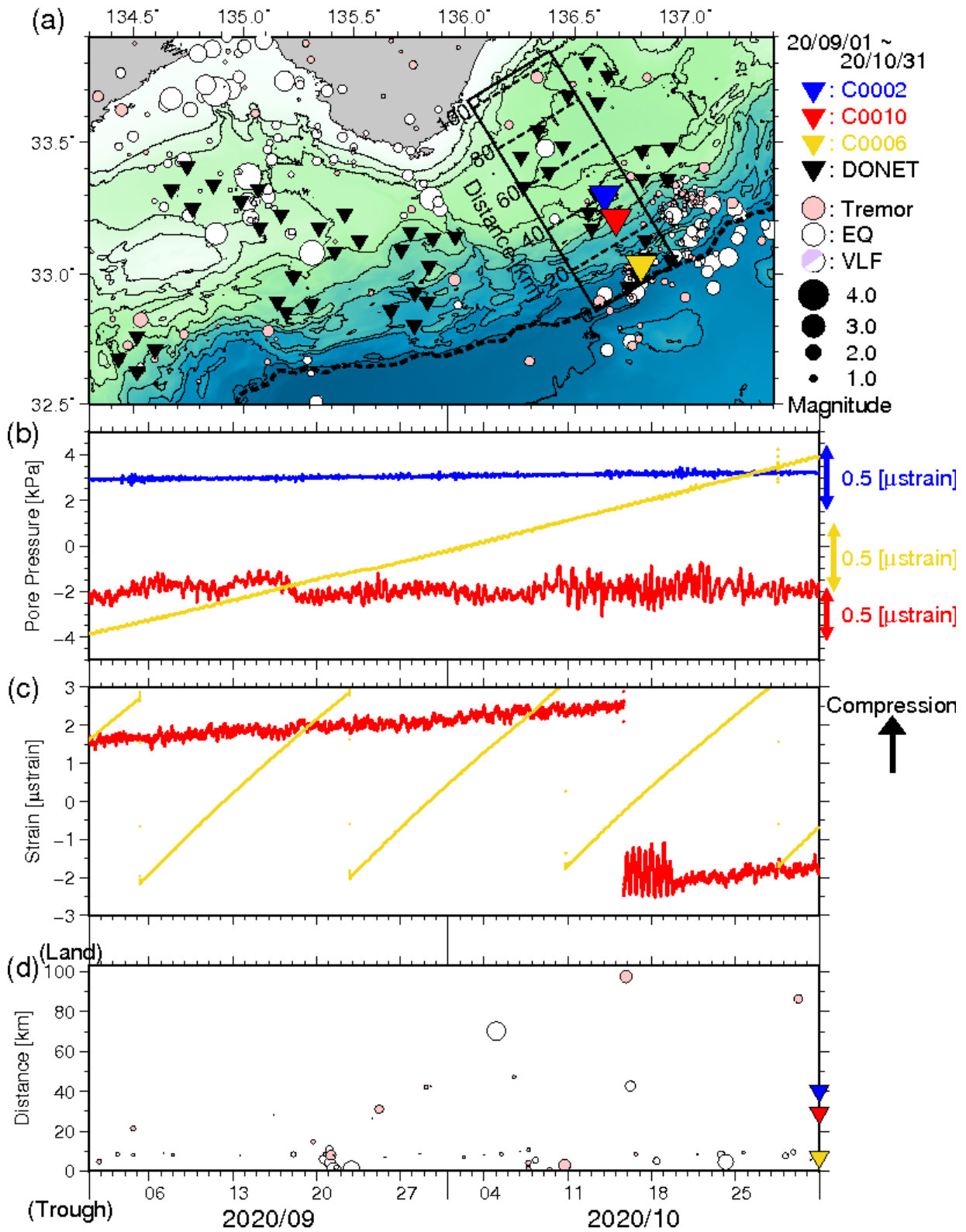
図3 直近2ヶ月間のSSE・低周波微動モニタリング(2020年9月1日~2020年10月31日)。 (a) 低周波微動と通常の地震の震央分布図(●:低周波微動、○:通常の地震)。それぞれの震源深さが、0~15 km及び0~60 kmの範囲に決まったイベントのみを示す。●は、超低周波地震のメカニズム解を示す。▼ ▼ ▼ ▼は、それぞれC0002・C0010・C0006・DONET観測点を示す。破線はトラフ軸を示す。(b) 長期孔内観測点における間隙水圧変化(—:C0002、—:C0010、—:C0006)。(c) 長期孔内観測点における体積歪変化(—:C0010、—:C0006)。(d) 低周波微動と通常地震の時空間分布。図3a中に実線で示した矩形領域内において発生したイベントについて示す。縦軸は、トラフ軸からの距離(km)を示す。
