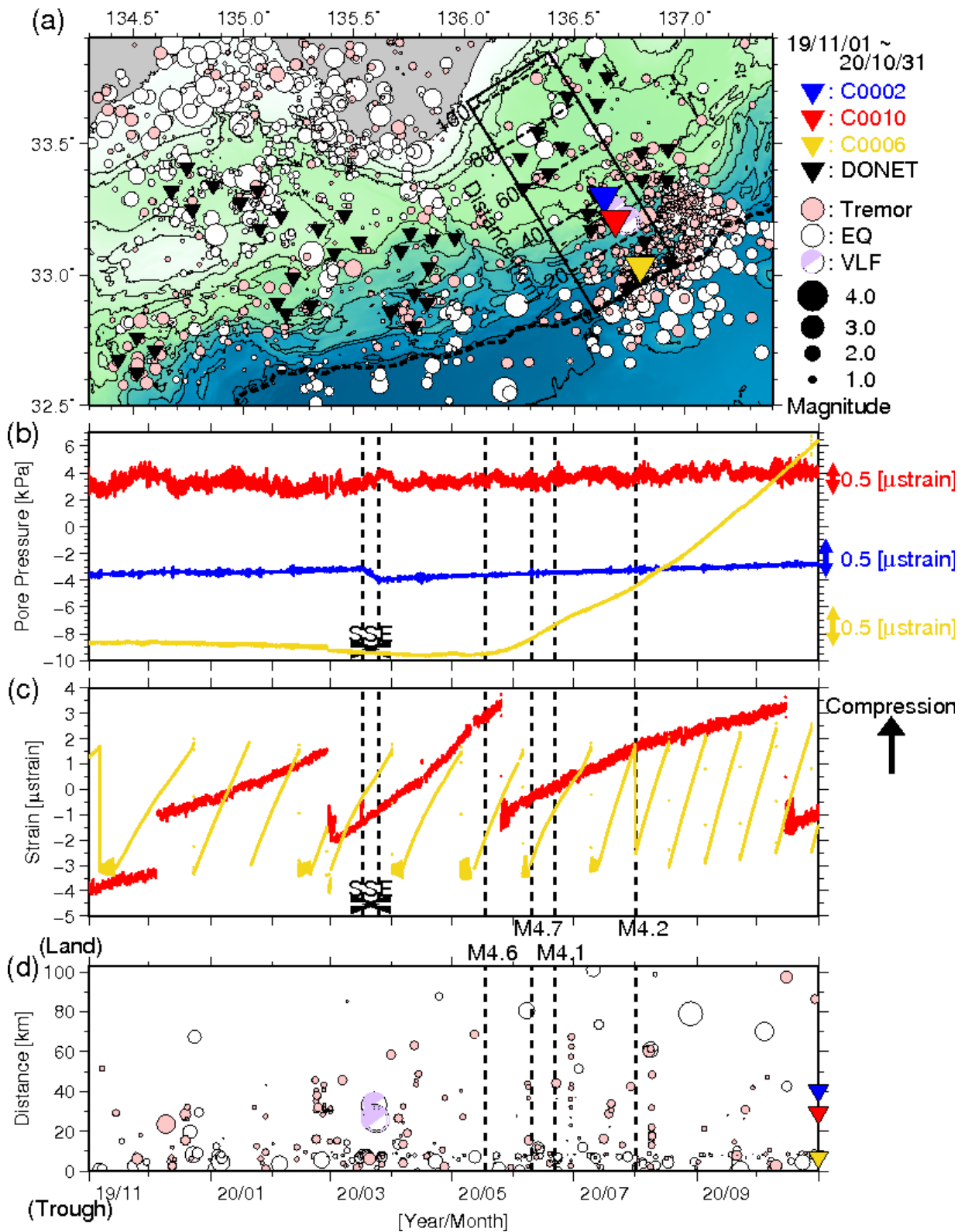
図4 直近1年間のSSE・低周波微動モニタリング(2019年11月1日~2020年10月31日)。図3と同様のシンボルにて表示している。(a)低周波微動の震央分布図。(b)間隙水圧変化。(c)体積歪変化。(d)低周波微動の時空間分布。超低周波地震のメカニズム解についても低周波微動と同様に示す。体積歪変化は、基準値を超えると歪計内のバルブを開けてリセットするため、相対値のみを使用。なお、2020年2月28日はノードA交換に伴うC0010水圧計の不具合のため、2020年3月2日、16日および4月16日は測器の状態確認や再起動のため、2020年5月10日~12日および6月3日はサーバの不具合のため、各期間において一部データが欠測している。点線で示す地震情報については、図3および図6を参照。
