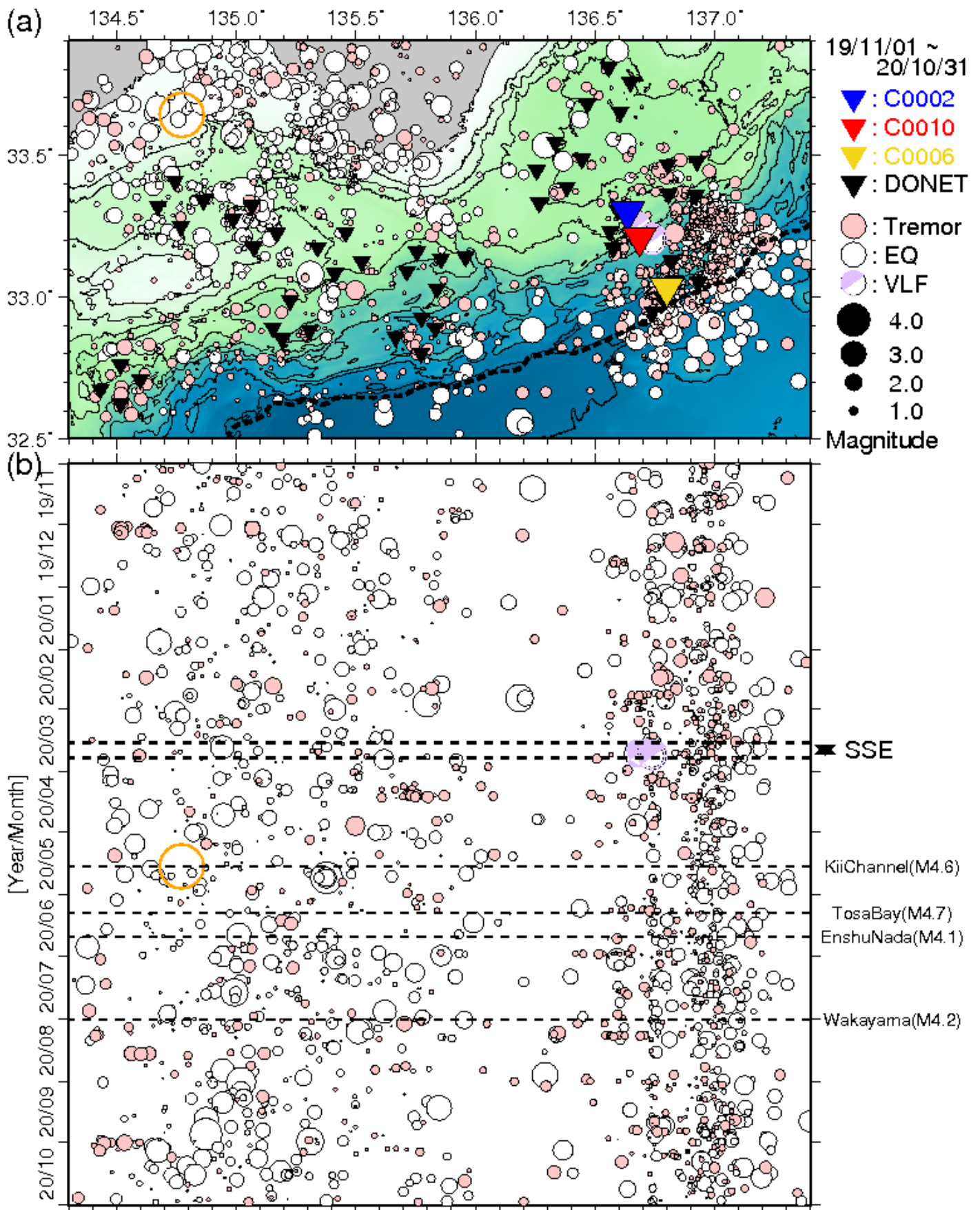
図6 直近1年間において熊野灘から室戸沖にて発生した低周波微動の時空間分布(2019年11月1日~2020年10月31日)。図3と同様のシンボルにて表示している。(a)低周波微動の震央分布図。(b)aに示した震央を経度方向へ投影した低周波微動の時空間分布図。超低周波地震のメカニズム解についても低周波微動と同様に示す。○は2020年5月17日に発生した紀伊水道地震を示す。
