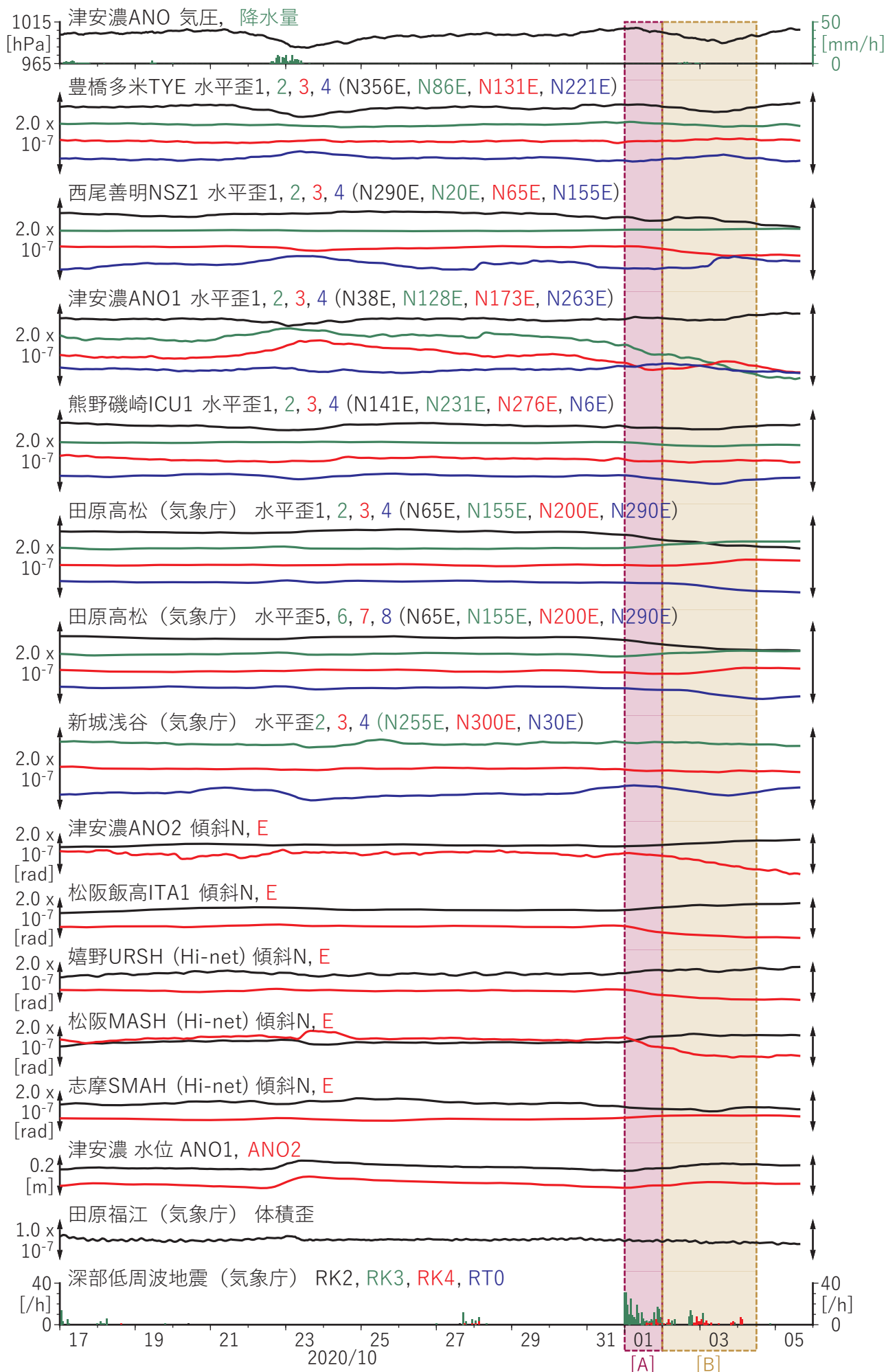
図9 紀伊半島～東海地方における歪・傾斜・地下水観測結果 (2020/10/17 00:00 - 2020/11/06 00:00 (JST)) (低周波地震は2020/11/05 00:00まで) 産業技術総合研究所 資料
