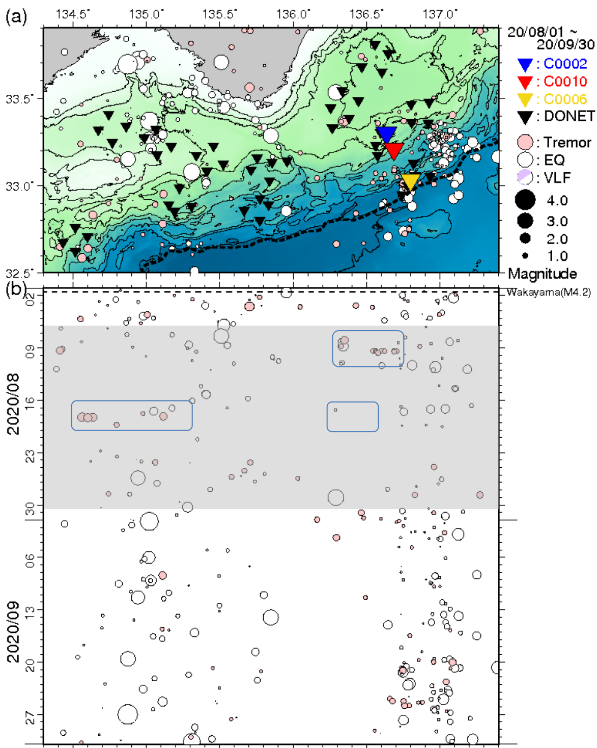
図5 直近2 ヶ月間において熊野灘から室戸沖にて発生した低周波微動の時空間分布(2020年8月1日~2020年9月30日)。図3と同様のシンボルにて表示している。(a) 低周波微動の震央分布図。(b) aに示した震央を経度方向へ投影した低周波微動の時空間分布図。グレーの背景部分はエアガン作業期間を示す。青線で囲んだイベントは、波形からエアガンとして確認されたイベントを示す。
