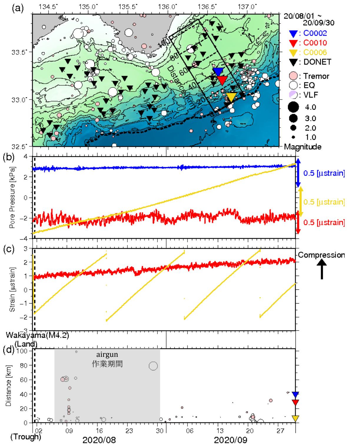
図3 直近2ヶ月間のSSE・低周波微動モニタリング(2020年8月1日~2020年9月30日)。(a) 低周波微動と通常地震の震央分布図(●:低周波微動、○:通常地震)。それぞれの震源深さが、0~15km及び0~60kmの範囲に決まったイベントのみを示す。●は、超低周波地震のメカニズム解を示す。▼▼▼▼は、それぞれC0002・C0010・C0006・DONET観測点を示す。破線はトラフ軸を示す。(b) 長期孔内観測点における間隙水圧変化(—:C0002、—:C0010、—:C0006)。(c) 長期孔内観測点における体積歪変化(—:C0010、—:C0006)。(d) 低周波微動と通常地震の時空間分布。図3a中に実線で示した矩形領域内において発生したイベントについて示す。縦軸は、トラフ軸からの距離(km)を示す。点線は2020年8月1日の和歌山県南部地震の発生時刻を示す。また、グレーの背景部分はエアガン作業期間を示す。
