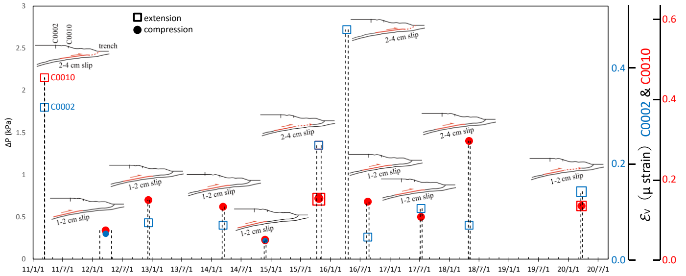
図7 孔内観測点において観測されたSSE 発生時の間隙水圧変化 (Araki et al. (2017) を加筆・修正)。間隙水圧変化 ( \Delta P ) とそれらを体積歪 ( \epsilon_v ) に換算したスケールを縦軸に示している。 ●・□は、それぞれ圧縮・伸長方向の間隙水圧変化を示す。青・赤のシンボルは、それぞれ C0002・C0010 の間隙水圧変化を示す。
