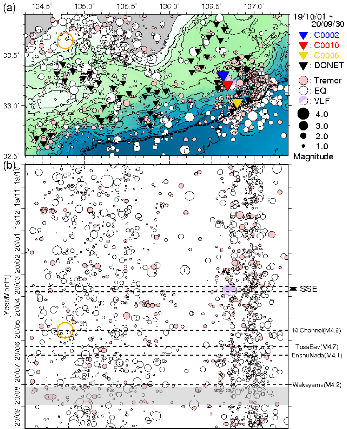
図6 直近1年間において熊野灘から室戸沖にて発生した低周波微動の時空間分布(2019年10月1日~2020年9月30日)。図3と同様のシンボルにて表示している。(a)低周波微動の震央分布図。(b)aに示した震央を経度方向へ投影した低周波微動の時空間分布図。超低周波地震のメカニズム解についても低周波微動と同様に示す。○は2020年5月17日に発生した紀伊水道地震を示す。また、グレーの背景部分はエアガン作業期間を示す。
