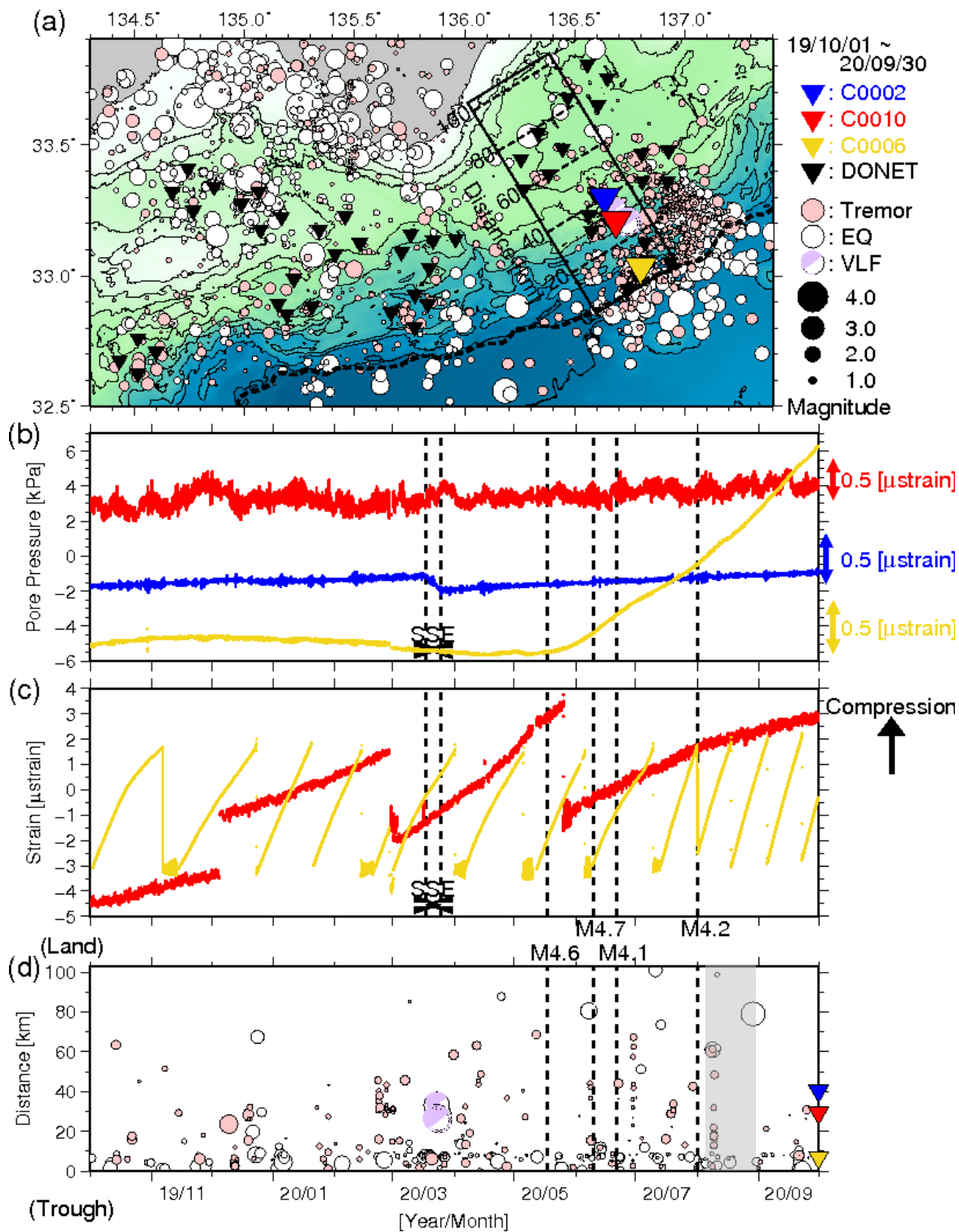
図4 直近1年間のSSE・低周波微動モニタリング(2019年10月1日~2020年9月30日)。図3と同様のシンボルにて表示している。(a)低周波微動の震央分布図。(b)間隙水圧変化。(c)体積歪変化。(d)低周波微動の時空間分布。超低周波地震のメカニズム解についても低周波微動と同様に示す。体積歪変化は、基準値を超えると歪計内のバルブを開けてリセットするため、相対値のみを使用。なお、2020年2月28日はノードA交換に伴うC0010水圧計の不具合のため、2020年3月2日、16日および4月16日は測器の状態確認や再起動のため、2020年5月10日~12日および6月3日はサーバの不具合のため、各期間において一部データが欠測している。点線で示す地震情報については、図3および図6を参照。また、グレーの背景部分はエアガン作業期間を示す。
