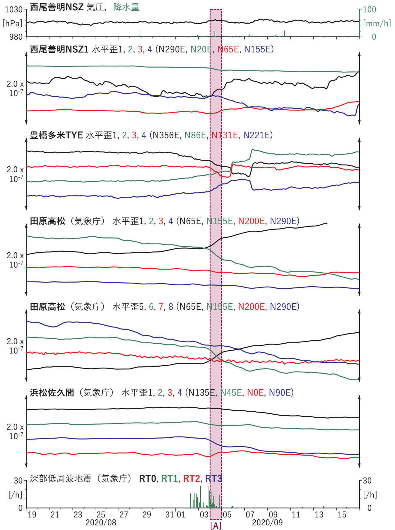
図02 歪の時間変化 (2020/08/19 00:00 - 2020/09/17 00:00 (JST))
