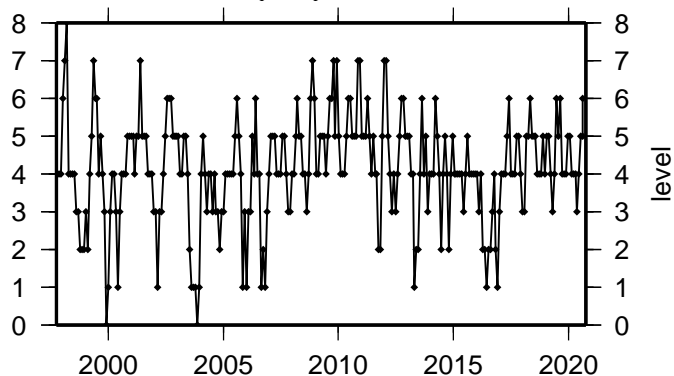
(5) 東海
