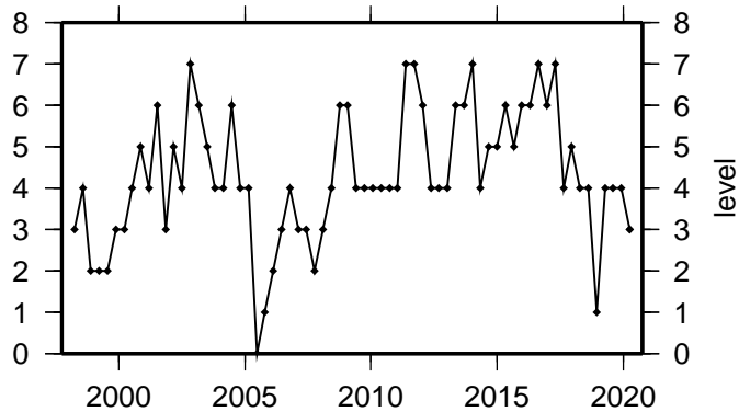
(6) 東南海
