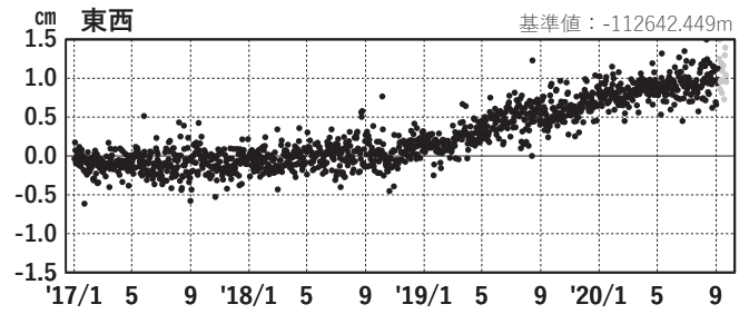
(4) 網野(960640)→香北(950439)
