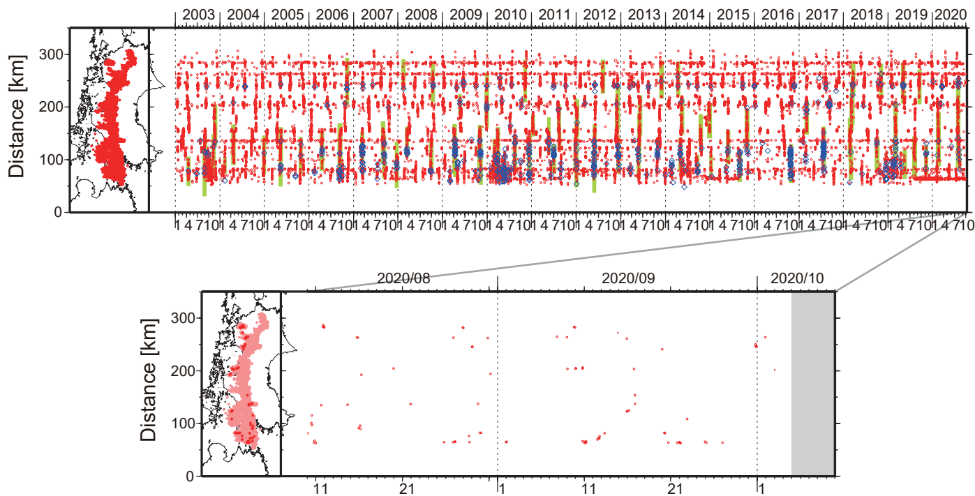
図1. 四国における2003年1月～2020年10月4日までの深部低周波微動の時空間分布(上図). 赤丸はエンベロープ相関・振幅ハイブリッド法 (Maeda and Obara, 2009) およびクラスタ処理 (Obara et al., 2010) によって1時間毎に自動処理された微動分布の重心である. 青菱形は周期20秒に卓越する超低周波地震 (Ito et al., 2007) である. 黄緑色太線は、これまでに検出された短期的スロースリップイベント (SSE) を示す. 下図は2020年9月を中心とした期間の拡大図である. 顕著な活動はとくに見られなかったものの、9月9日～10日頃には愛媛県東部において、9月10～13日頃には豊後水道付近において、9月30日～10月1日頃には愛媛・香川・徳島県境付近において、それぞれ小規模な活動がみられた. 9月9日頃には香川県付近において、9月15～16日頃には愛媛県西部において、9月20～22日頃には豊後水道において、それぞれごく小規模な活動がみられた.
