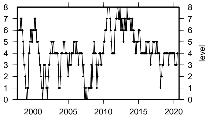
(4) 駿河湾
