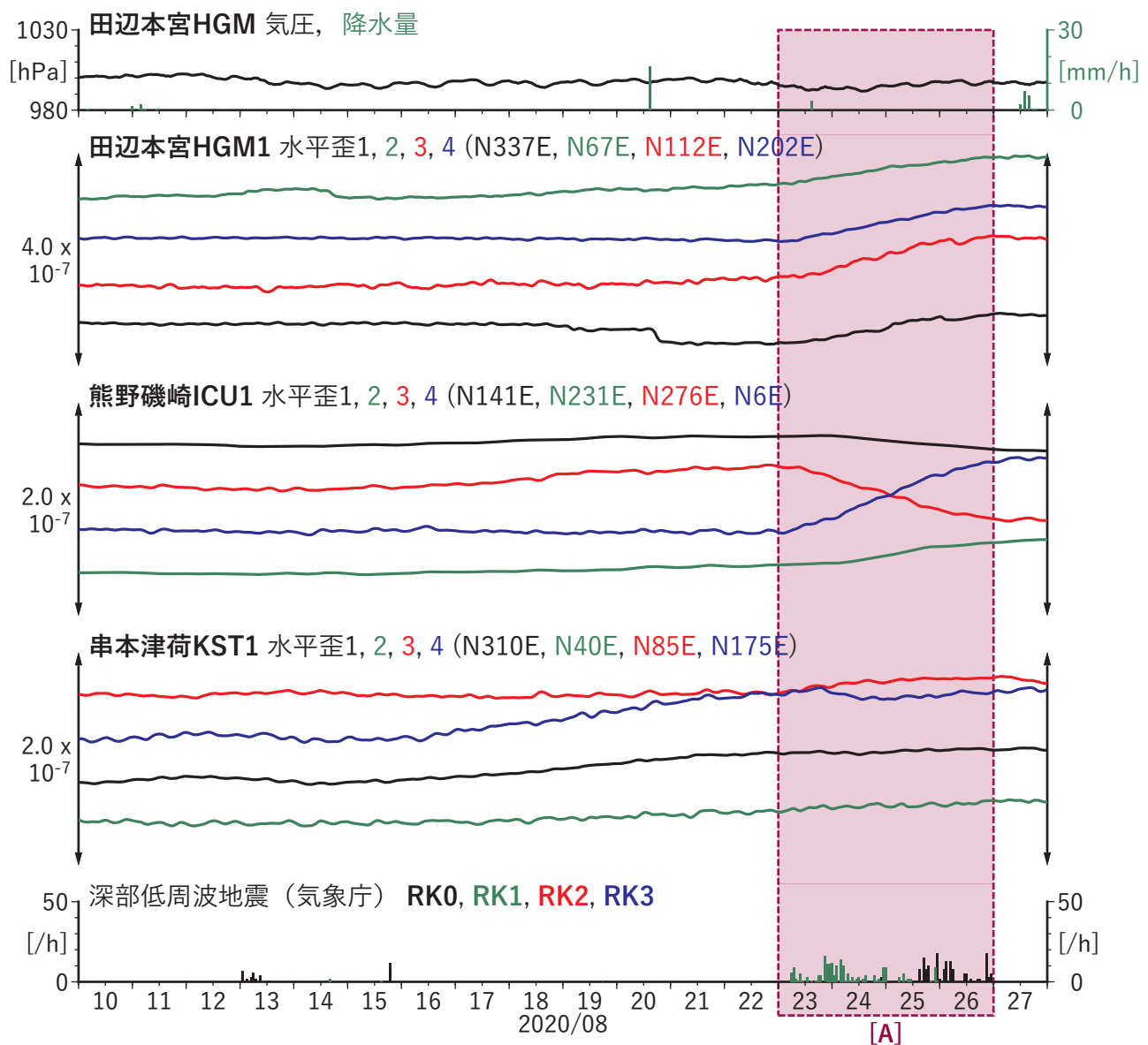
図15 歪の時間変化 (2020/08/10 00:00 - 2020/08/28 00:00 (JST))
