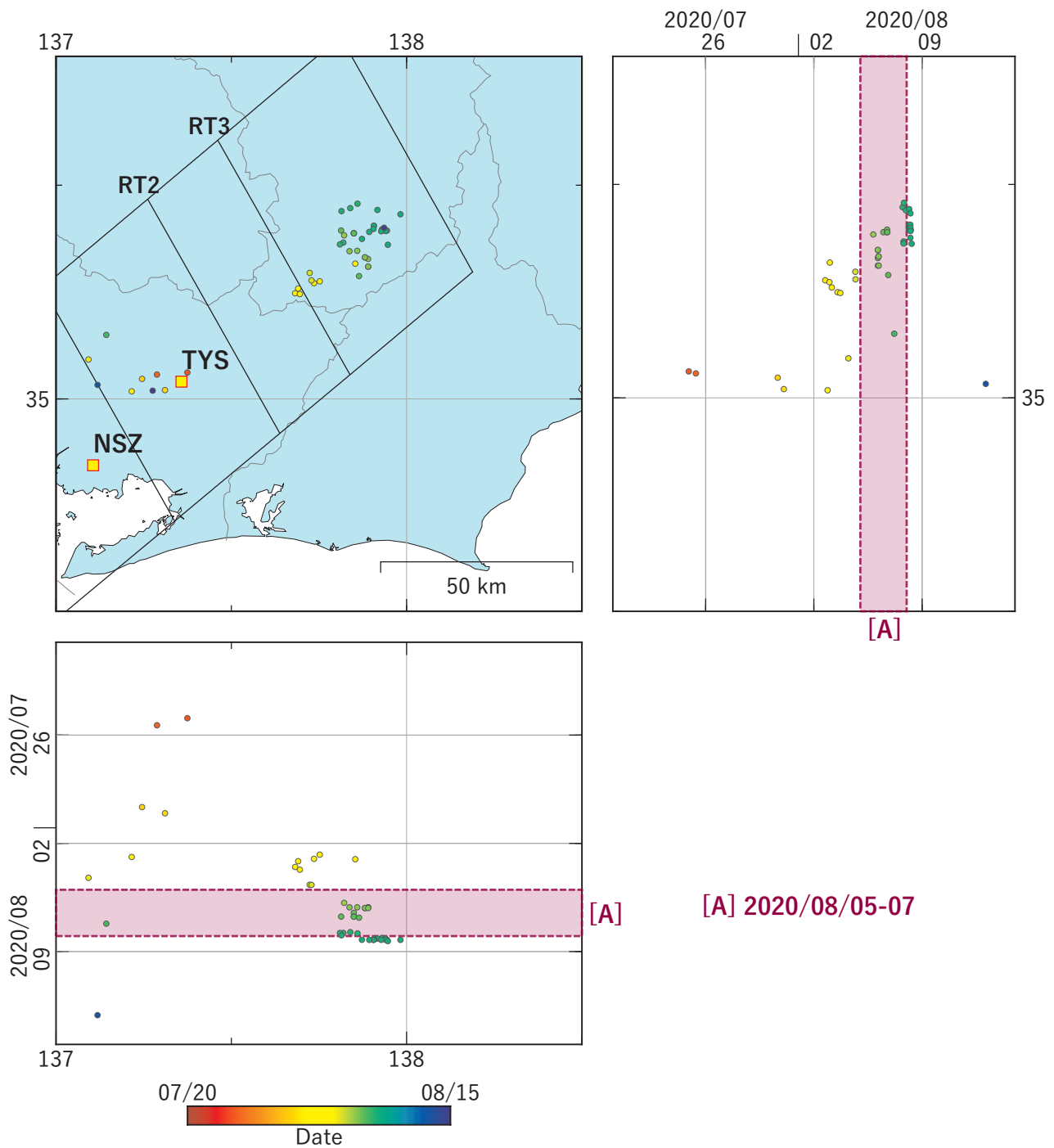
図1 東海地方における深部低周波地震の時空間分布図。 (2020/07/20 00:00 - 2020/08/15 00:00 (JST)) 気象庁カタログによる。
