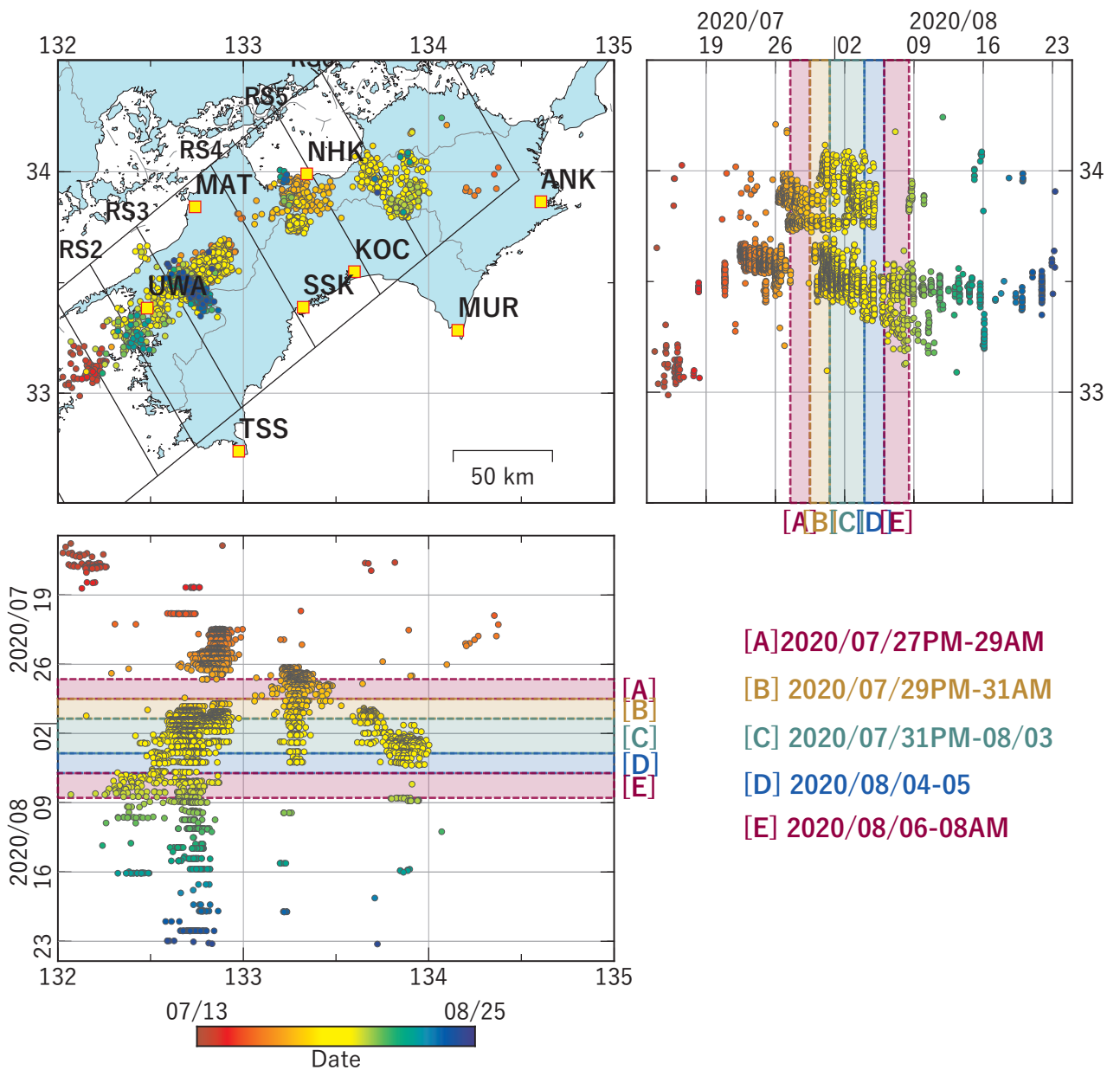
図4 四国地方における深部低周波地震の時空間分布図。 (2020/07/13 00:00 - 2020/08/25 00:00 (JST)) 気象庁カタログによる。
