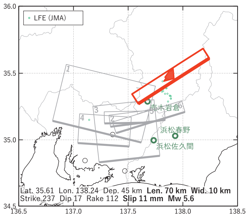
図3 2020/08/05-07 の歪・傾斜変化 (図2[A]) を説明する断層モデル。
