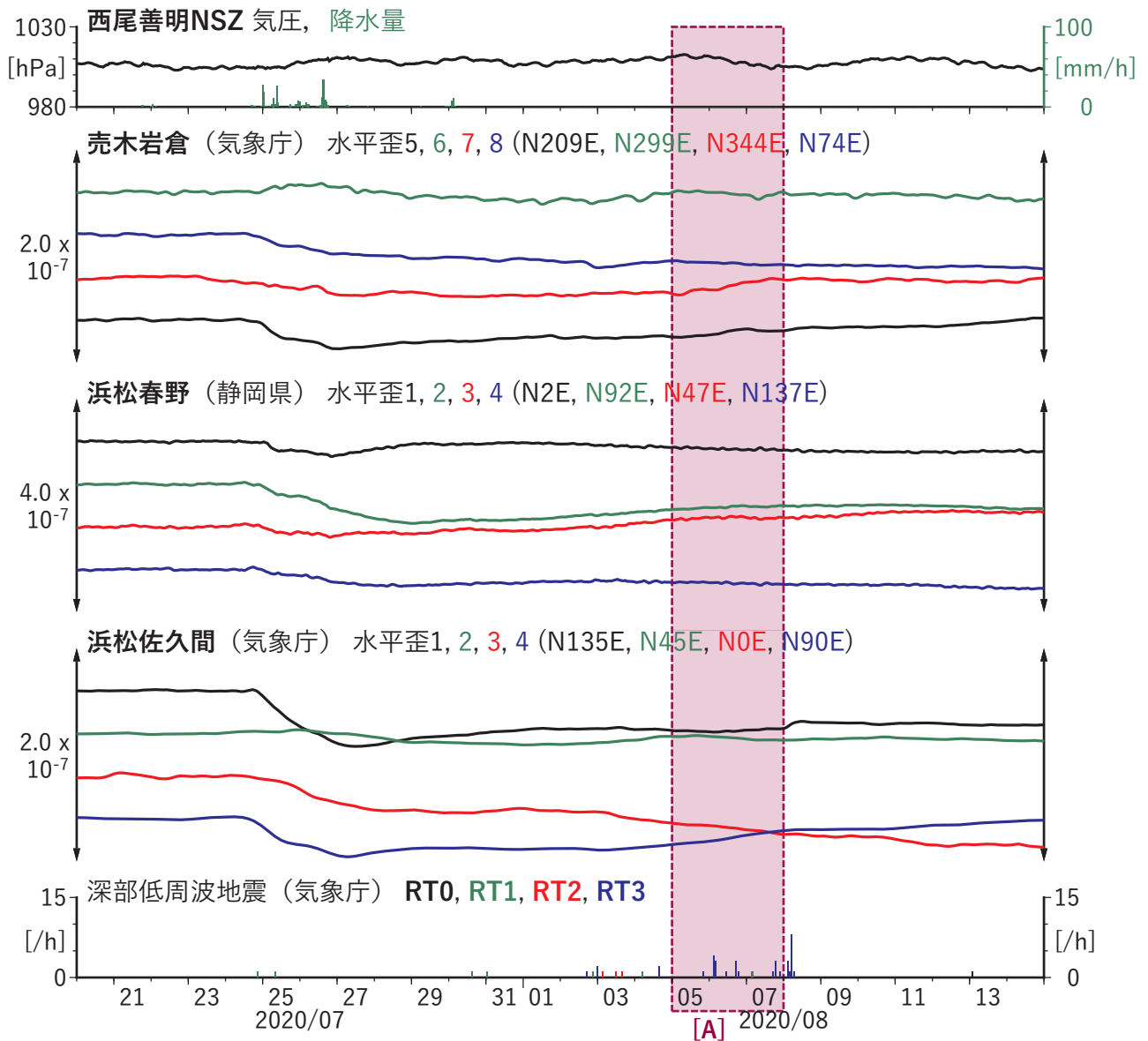
図2 歪の時間変化 (2020/07/20 00:00 - 2020/08/15 00:00 (JST))
