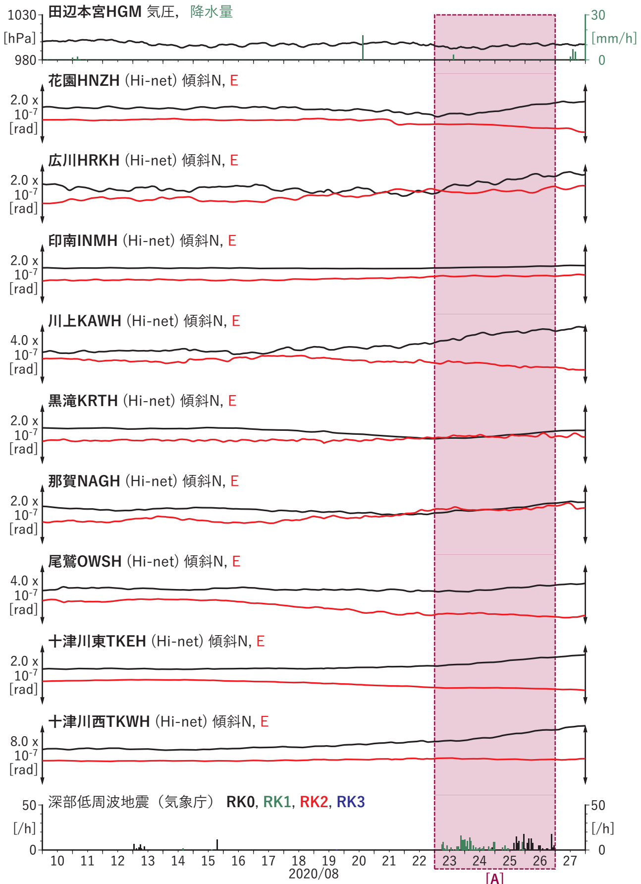
図16 傾斜の時間変化 (2020/08/10 00:00 - 2020/08/28 00:00 (JST))
