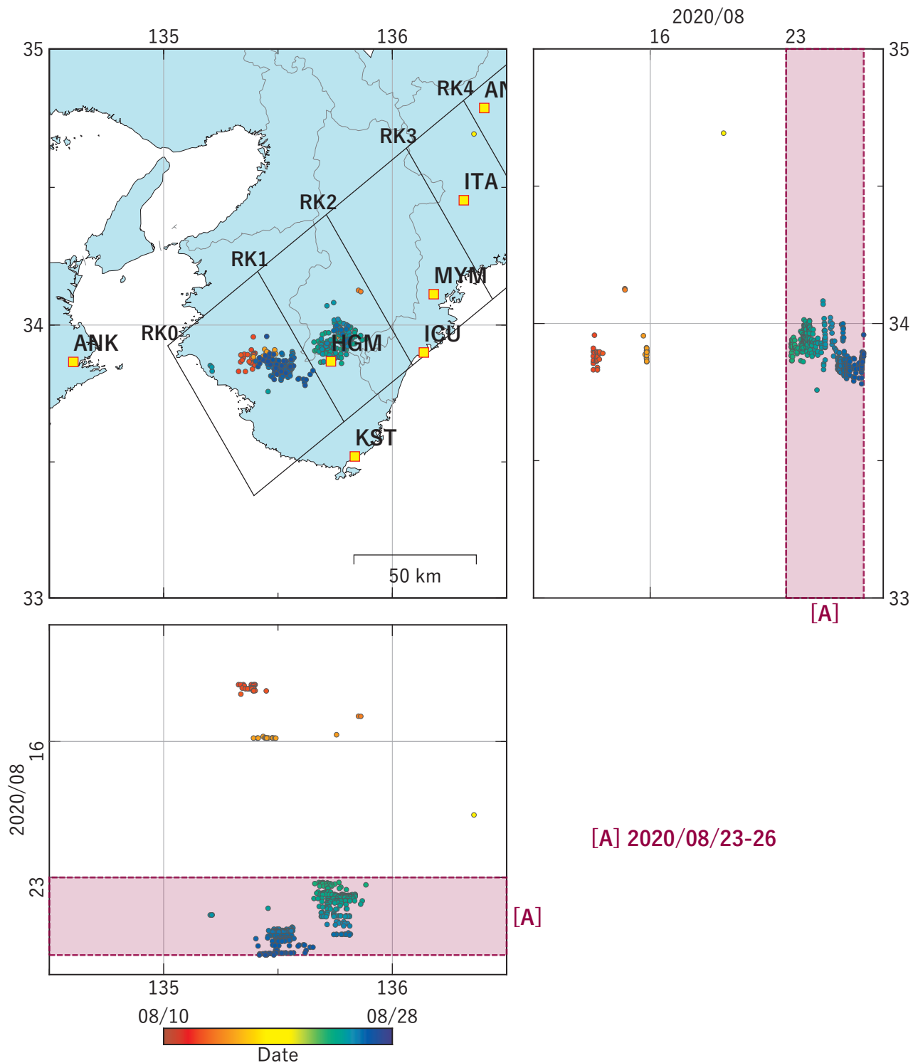
図14 紀伊半島における深部低周波地震の時空間分布図。 (2020/08/10 00:00 - 2020/08/28 00:00 (JST)) 気象庁カタログによる。
