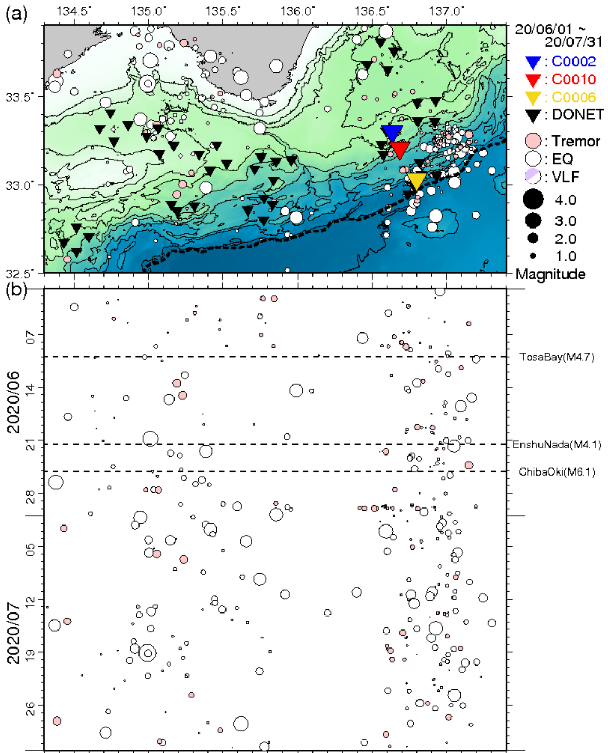
図5 直近2ヵ月間において熊野灘から室戸沖にて発生した低周波微動の時空間分布(2020年6月1日~2020年7月31日)。図3と同様のシンボルにて表示している。(a)低周波微動の震央分布図。(b)aに示した震央を経度方向へ投影した低周波微動の時空間分布図。
