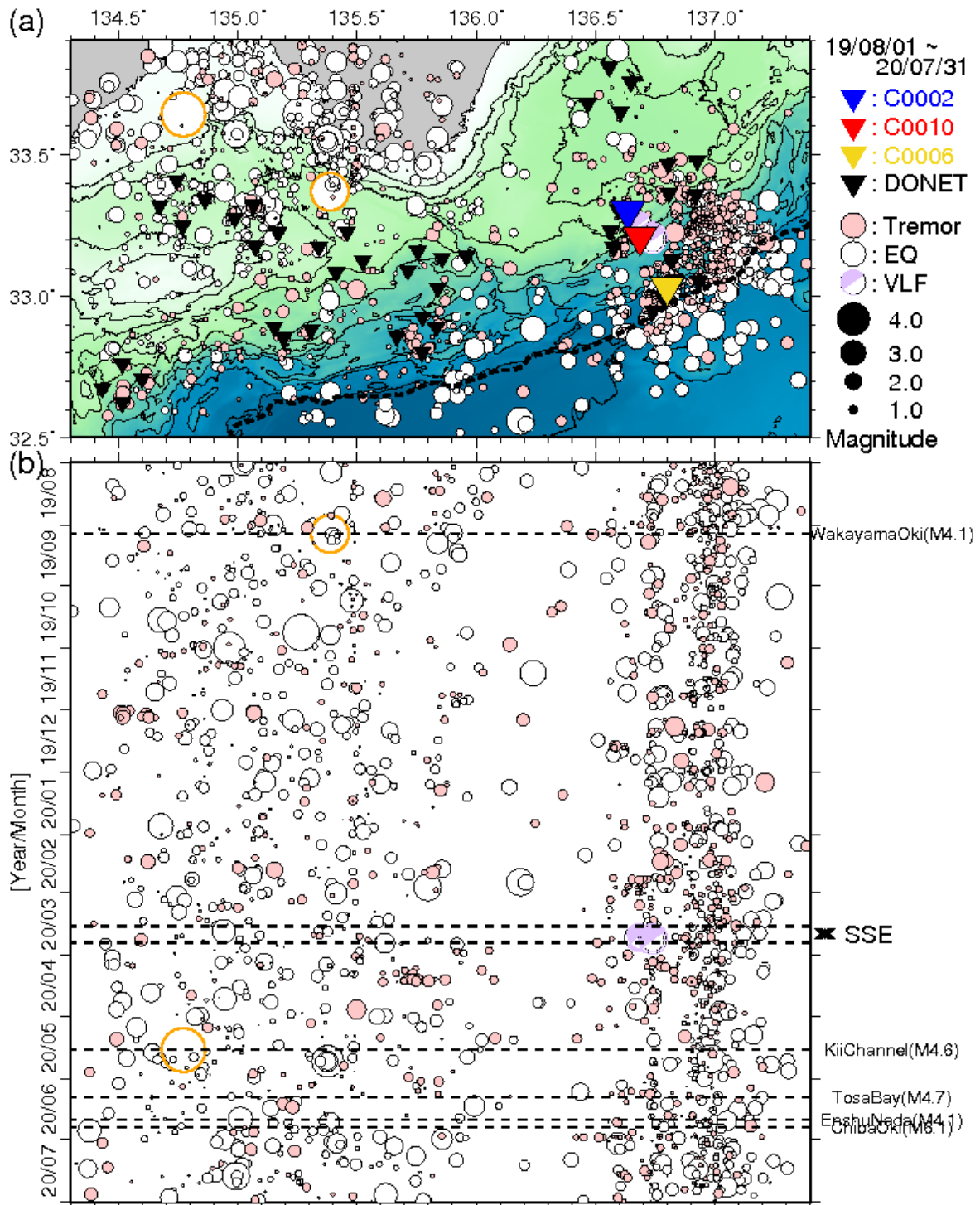
図6 直近1年間において熊野灘から室戸沖にて発生した低周波微動の時空間分布(2019年8月1日~2020年7月31日)。図3と同様のシンボルにて表示している。(a)低周波微動の震央分布図。(b)aに示した震央を経度方向へ投影した低周波微動の時空間分布図。超低周波地震のメカニズム解についても低周波微動と同様に示す。○は2019年9月5日に発生した和歌山沖地震、2020年5月17日に発生した紀伊水道地震をそれぞれ示す。
