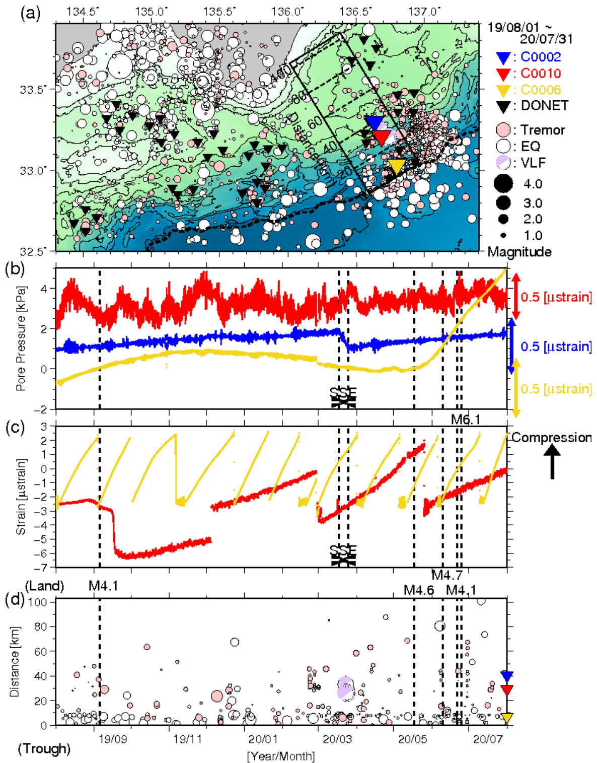
図4 直近1年間のSSE・低周波微動モニタリング(2019年8月1日~2020年7月31日)。図3と同様のシンボルにて表示している。(a)低周波微動の震央分布図。(b)間隙水圧変化。(c)体積歪変化。(d)低周波微動の時空間分布。超低周波地震のメカニズム解についても低周波微動と同様に示す。体積歪変化は、基準値を超えると歪計内のバルブを開けてリセットするため、相対値のみを使用。なお、2020年2月28日はノードA交換に伴うC0010水圧計の不具合のため、2020年3月2日、16日および4月16日は測器の状態確認や再起動のため、2020年5月10日~12日および6月3日はサーバの不具合のため、各期間において一部データが欠測している。点線で示す地震情報については、図3および図6を参照。
