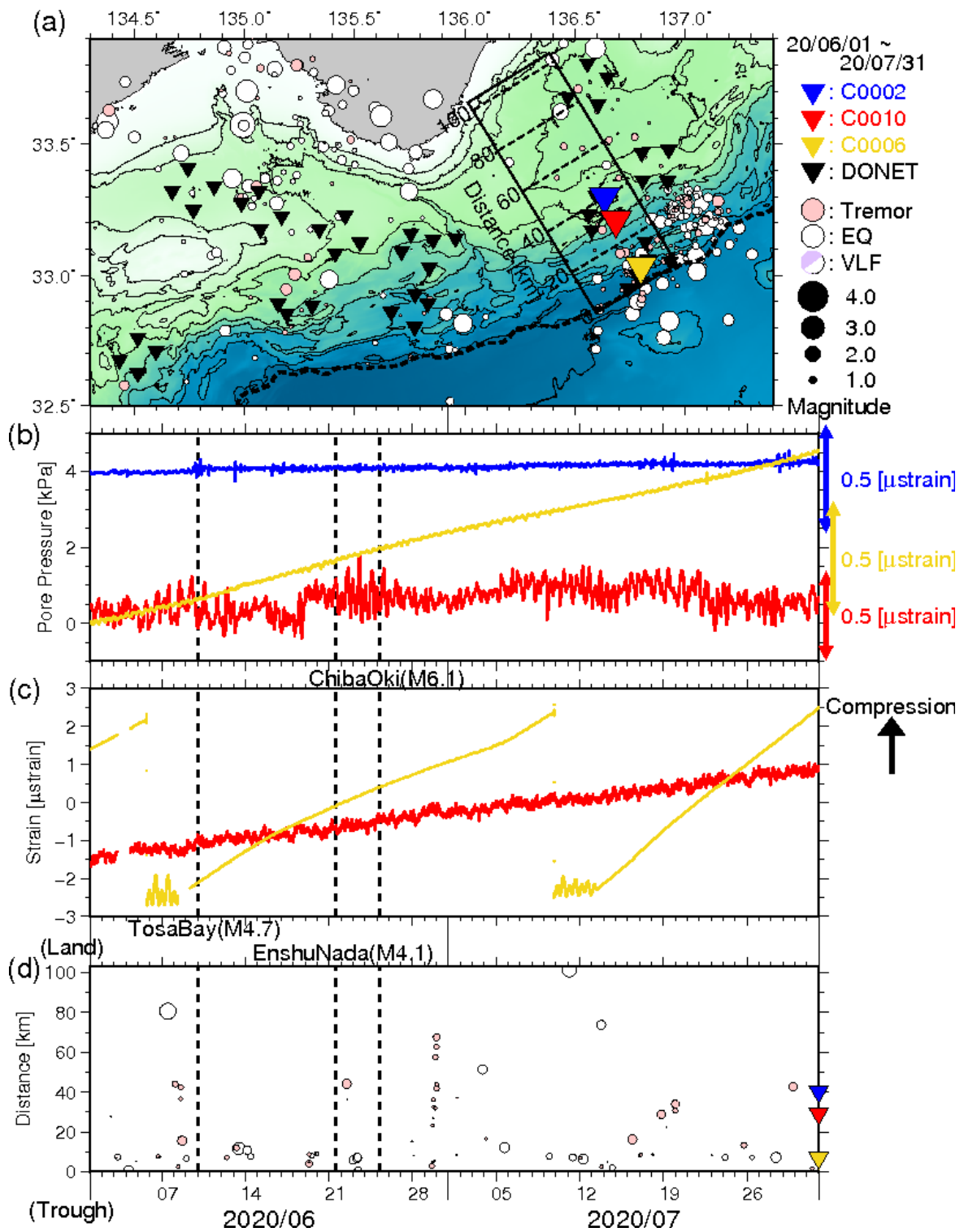
図3 直近2ヶ月間のSSE・低周波微動モニタリング(2020年6月1日~2020年7月31日)。(a) 低周波微動と通常地震の震央分布図(●:低周波微動、○:通常地震)。それぞれの震源深さが、0~15 km及び0~60 kmの範囲に決まったイベントのみを示す。●は、超低周波地震のメカニズム解を示す。▼▼▼は、それぞれC0002・C0010・C0006・DONET観測点を示す。破線はトラフ軸を示す。(b) 長期孔内観測点における間隙水圧変化(—:C0002、—:C0010、—:C0006)。(c) 長期孔内観測点における体積歪変化(—:C0010、—:C0006)。(d) 低周波微動と通常地震の時空間分布。図3a中に実線で示した矩形領域内において発生したイベントについて示す。縦軸は、トラフ軸からの距離(km)を示す。点線は2020年6月10日の土佐湾地震、6月21日の遠州灘地震、6月25日の千葉東方沖地震の発生時刻をそれぞれ示す。
