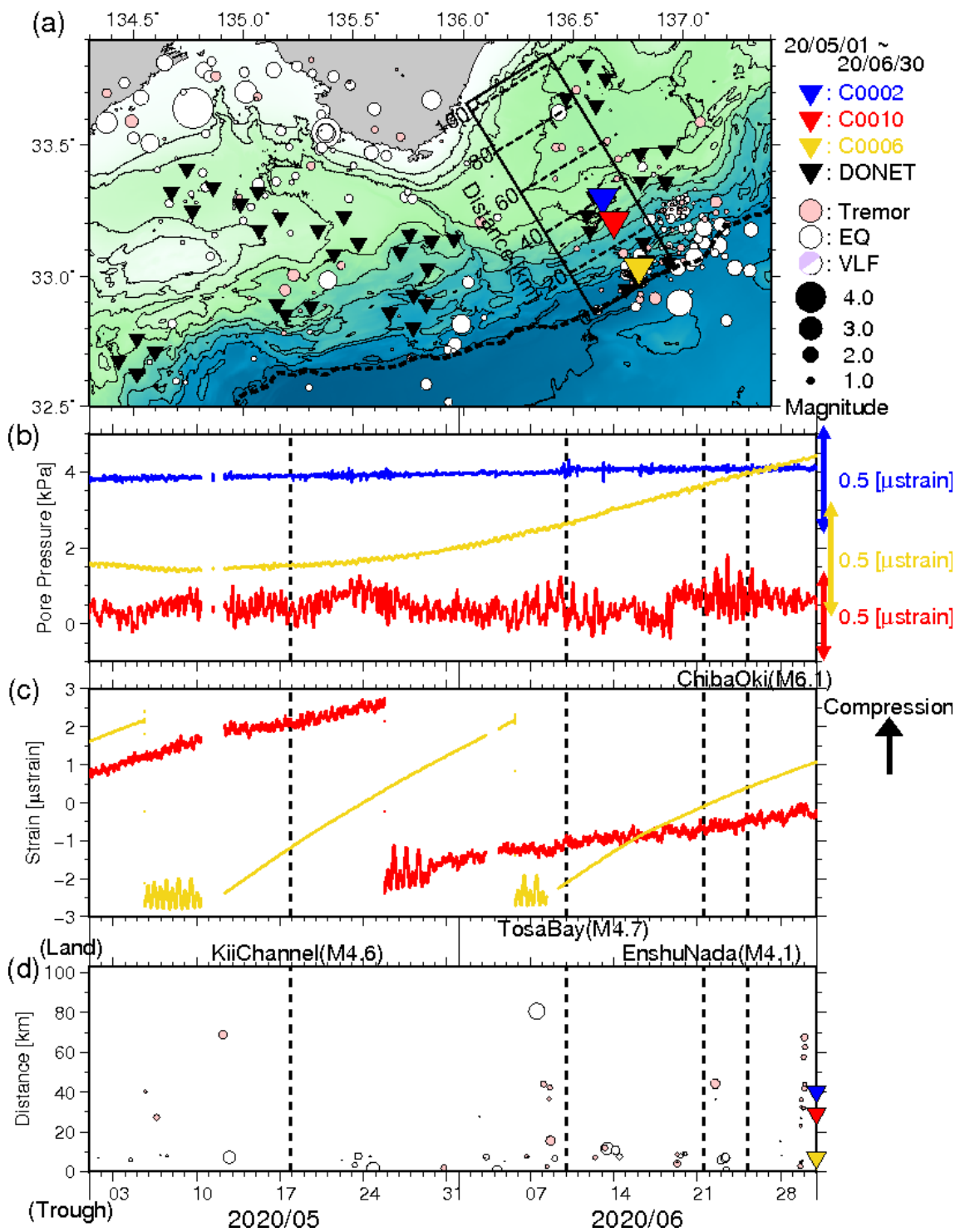
図3 直近2ヶ月間のSSE・低周波微動モニタリング(2020年5月1日~2020年6月30日)。(a) 低周波微動と通常の地震の震央分布図(●:低周波微動、○:通常の地震)。それぞれの震源深さが、0~15km及び0~60kmの範囲に決まったイベントのみを示す。●は、超低周波地震のメカニズム解を示す。▼▼▼は、それぞれC0002・C0010・C0006・DONET観測点を示す。破線はトラフ軸を示す。(b) 長期孔内観測点における間隙水圧変化(—:C0002、—:C0010、—:C0006)。(c) 長期孔内観測点における体積歪変化(—:C0010、—:C0006)。(d) 低周波微動と通常地震の時空間分布。図3a中に実線で示した矩形領域内において発生したイベントについて示す。縦軸は、トラフ軸からの距離(km)を示す。点線は2020年5月17日の紀伊水道地震、6月10日の土佐湾地震、6月21日の遠州灘地震、6月25日の千葉東方沖地震の発生時刻をそれぞれ示す。
