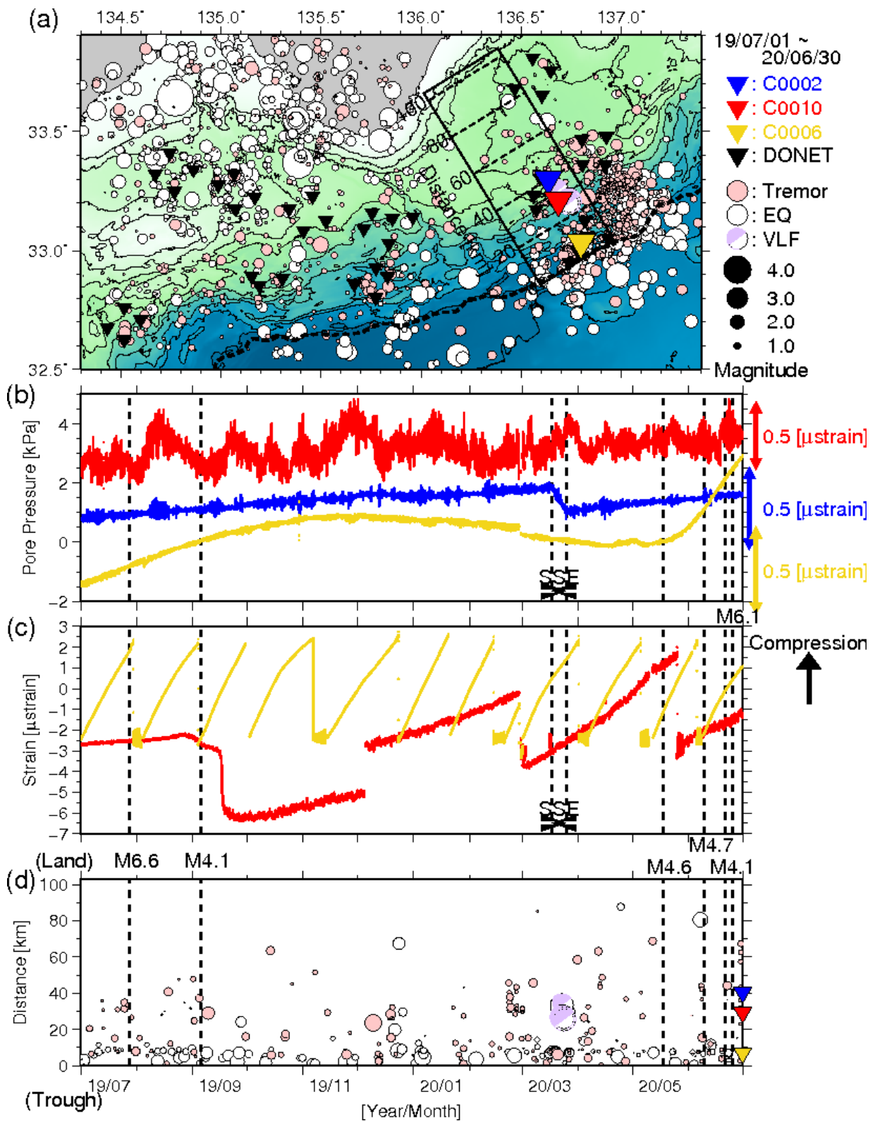
図4 直近1年間のSSE・低周波微動モニタリング(2019年7月1日~2020年6月30日)。図3と同様のシンボルにて表示している。(a)低周波微動の震央分布図。(b)間隙水圧変化。(c)体積歪変化。(d)低周波微動の時空間分布。超低周波地震のメカニズム解についても低周波微動と同様に示す。体積歪変化は、基準値を超えると歪計内のバルブを開けてリセットするため、相対値のみを使用。なお、2020年2月28日はノードA交換に伴うC0010水圧計の不具合のため、2020年3月2日、16日および4月16日は測器の状態確認や再起動のため、2020年5月10日~12日および6月3日はサーバの不具合のため、各期間において一部データが欠測している。点線で示す地震情報については、図3および図6を参照。
