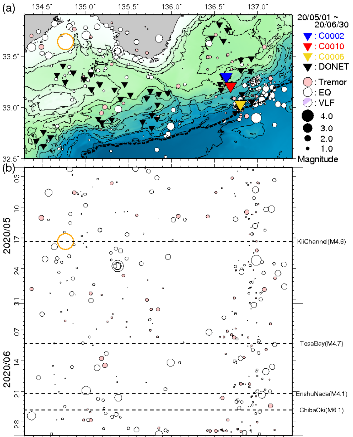
図5 直近2ヵ月間において熊野灘から室戸沖にて発生した低周波微動の時空間分布(2020年5月1日~2020年6月30日)。図3と同様のシンボルにて表示している。(a)低周波微動の震央分布図。(b)aに示した震央を経度方向へ投影した低周波微動の時空間分布図。○は2020年5月17日に発生した紀伊水道地震を示す。
