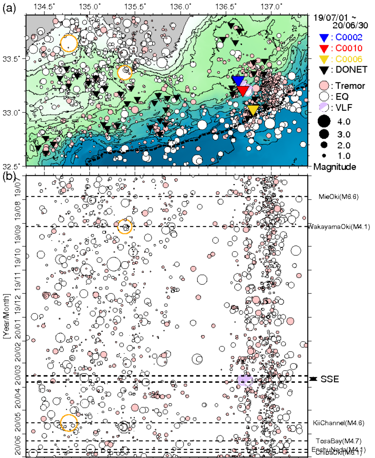
図6 直近1年間において熊野灘から室戸沖にて発生した低周波微動の時空間分布(2019年7月1日~2020年6月30日)。図3と同様のシンボルにて表示している。(a)低周波微動の震央分布図。
