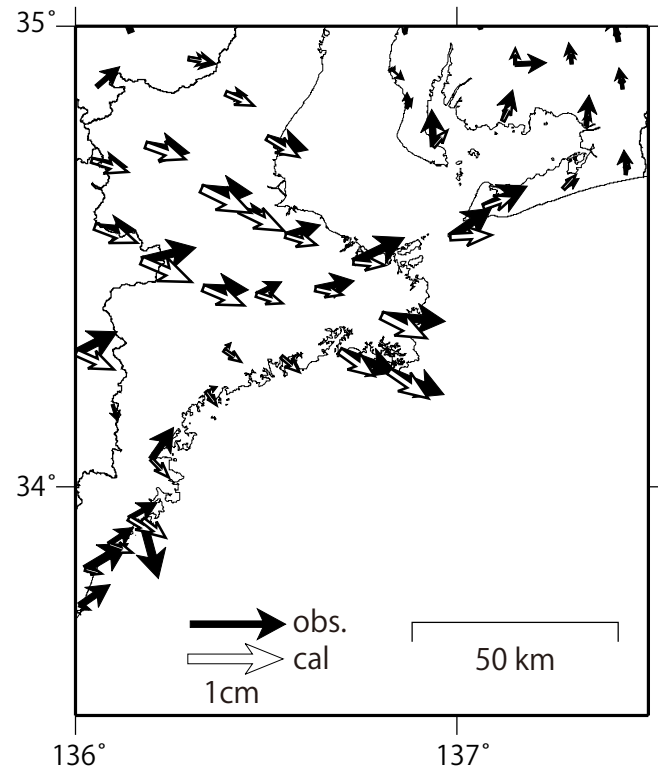
観測値（黒）と計算値（白）の比較 (2019/1/1 - 2020/6/10)
