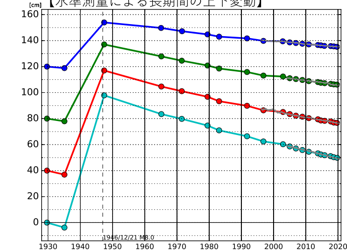
【水準測量による長期間の上下変動】
