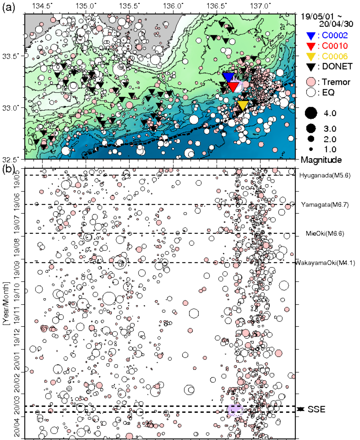
図6 直近1年間において熊野灘から室戸沖にて発生した低周波微動の時空間分布(2019年5月1日~2020年4月30日)。図3と同様のシンボルにて表示している。(a)低周波微動の震央分布図。(b)aに示した震央を経度方向へ投影した低周波微動の時空間分布図。超低周波地震についても同様に示す。
