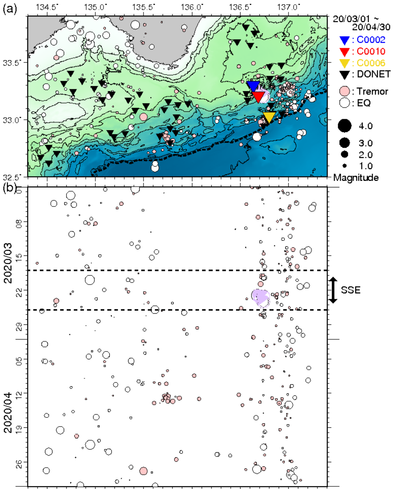
図5 直近2ヵ月間において熊野灘から室戸沖にて発生した低周波微動の時空間分布(2020年3月1日~2020年4月30日)。図3と同様のシンボルにて表示している。(a)低周波微動の震央分布図。(b)aに示した震央を経度方向へ投影した低周波微動の時空間分布図。超低周波地震についても同様に示す。
