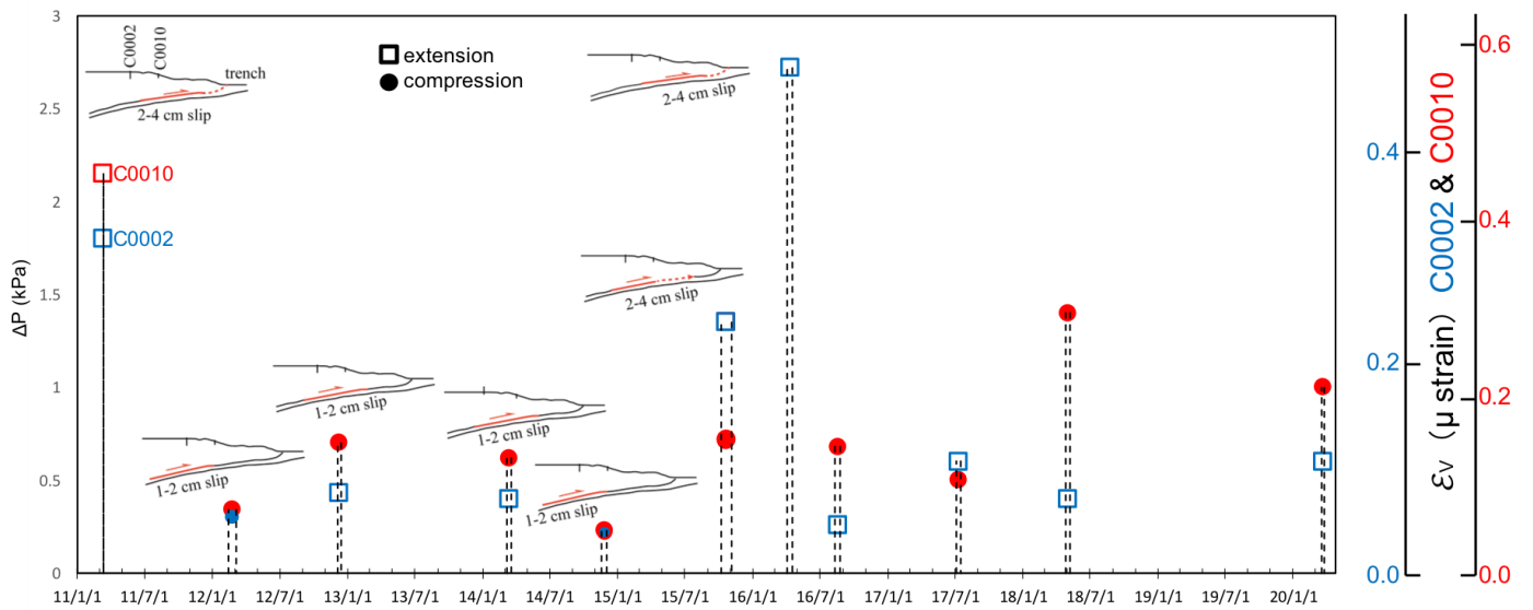
図7 孔内観測点において観測されたSSE 発生時の間隙水圧変化 (Araki et al. (2017) を加筆・修正)。間隙水圧変化 ( \Delta P ) とそれらを体積歪 ( \epsilon_v ) に換算したスケールを縦軸に示している。 \bullet ・ \square は、それぞれ圧縮・伸長方向の間隙水圧変化を示す。青・赤のシンボルは、それぞれ C0002・C0010 の間隙水圧変化を示す。
