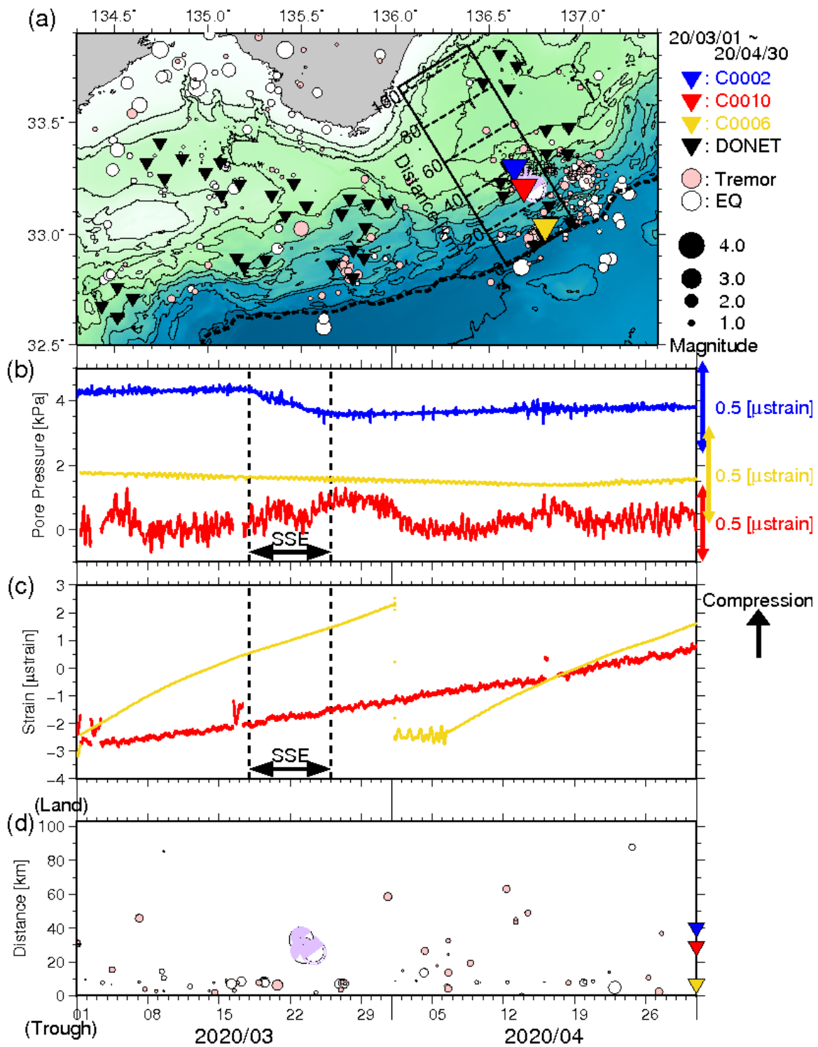
図3 直近2ヶ月間のSSE・低周波微動モニタリング(2020年3月1日~2020年4月30日)。(a) 低周波微動と通常の地震の震央分布図(●:低周波微動、○:通常の地震)。それぞれの震源深さが、0~15km及び0~60kmの範囲に決まったイベントのみを示す。●は、超低周波地震のメカニズム解を示す。▼▼▼は、それぞれC0002・C0010・C0006・DONET観測点を示す。破線はトラフ軸を示す。(b) 長期孔内観測点における間隙水圧変化(—:C0002、—:C0010、—:C0006)。(c) 長期孔内観測点における体積歪変化(—:C0010、—:C0006)。(d) 低周波微動と通常地震の時空間分布。図3a中に実線で示した矩形領域内において発生したイベントについて示す。超低周波地震についても同様に示す。縦軸は、トラフ軸からの距離(km)を示す。
