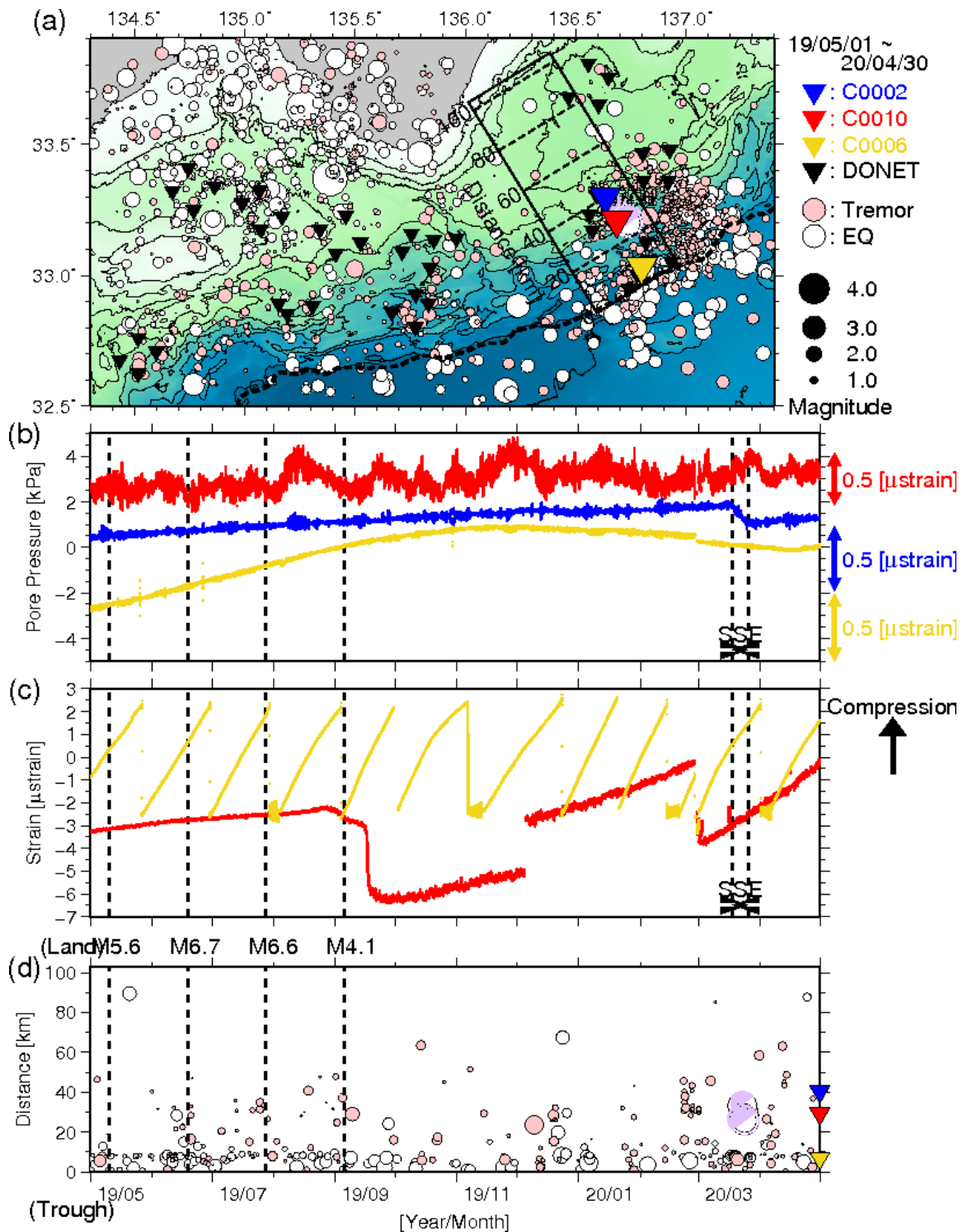
図4 直近1年間のSSE・低周波微動モニタリング(2019年5月1日~2020年4月30日)。図3と同様のシンボルにて表示している。(a)低周波微動の震央分布図。(b)間隙水圧変化。(c)体積歪変化。(d)低周波微動の時空間分布。超低周波地震についても、同様に示す。体積歪変化は、基準値を超えると歪計内のバルブを開けてリセットするため、相対値のみを使用。なお、2020年2月28日はノードA交換に伴うC0010水圧計の不具合のため、2020年3月2日、16日および4月16日は測器の状態確認や再起動などの実施により、各期間において一部データが欠測している。
