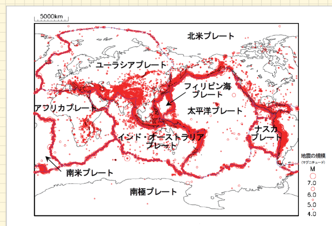
図：気象庁 https://www.data.jma.go.jp/eqev/data/jishin/about_eq.html ※2014年から2023年の間に発生した地震の震央分布。震源データは、米国地質調査所による。
