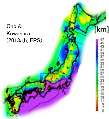
図1 列島を弾性層・粘弾性層の2層構造に分けた時の、弾性層の厚さ分布。これまでに得られた、微小地震の震源分布、地殻・マントル構造、GNSSIによる歪速度等のデータを総合して作成。
