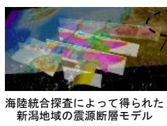
海溝型巨大地震と内陸地震の関係
