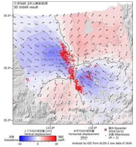
3次元SAR干渉解析による2016年鳥取県中部の地震に伴う三次元地殻変動分布 (矢印は水平変位、色は上下変動)
