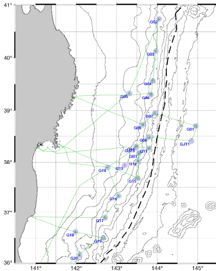
「よこすか」を用いて行われた日本海溝沿いの海底地殻変動観測航海(YK16-02)の航跡図
