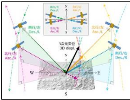
3次元SAR干渉解析の原理
