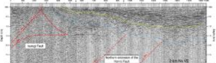
石動断層 法林寺断層(伏在)
