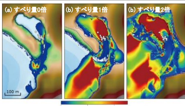
日向灘セグメントのすべり量に応じた大分県龍神池周辺の土砂堆積分布の変化。○は津波堆積物が発見された位置
