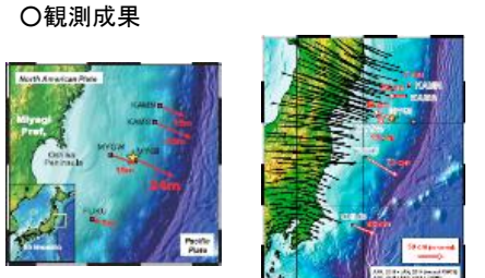
東北地方太平洋沖地震時の海底の変動
