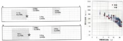
長大な断層の「レシピ」の検証
