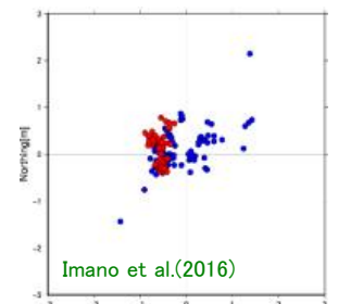
初期アレイ形状を修正することで、任意の位置からの測距ではRMS 0.5m以下の精度が得た。
