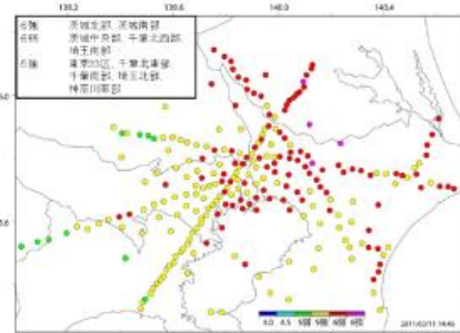
MeSO-net記録による計測震度相当値
