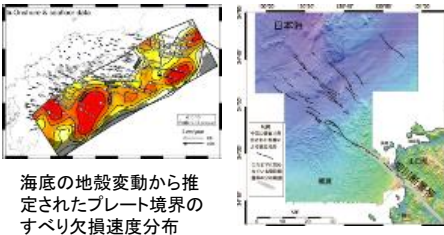
海底地形調査から確認された菊川断層帯の延長部
