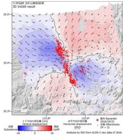
3次元SAR干渉解析による2016年鳥取県中部の地震に伴う三次元地殻変動分布 (矢印は水平変位、色は上下変動)
