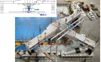
H23・24(建築基準整備促進事業)：長周期地震動に対する免震建築物の安全性検証
