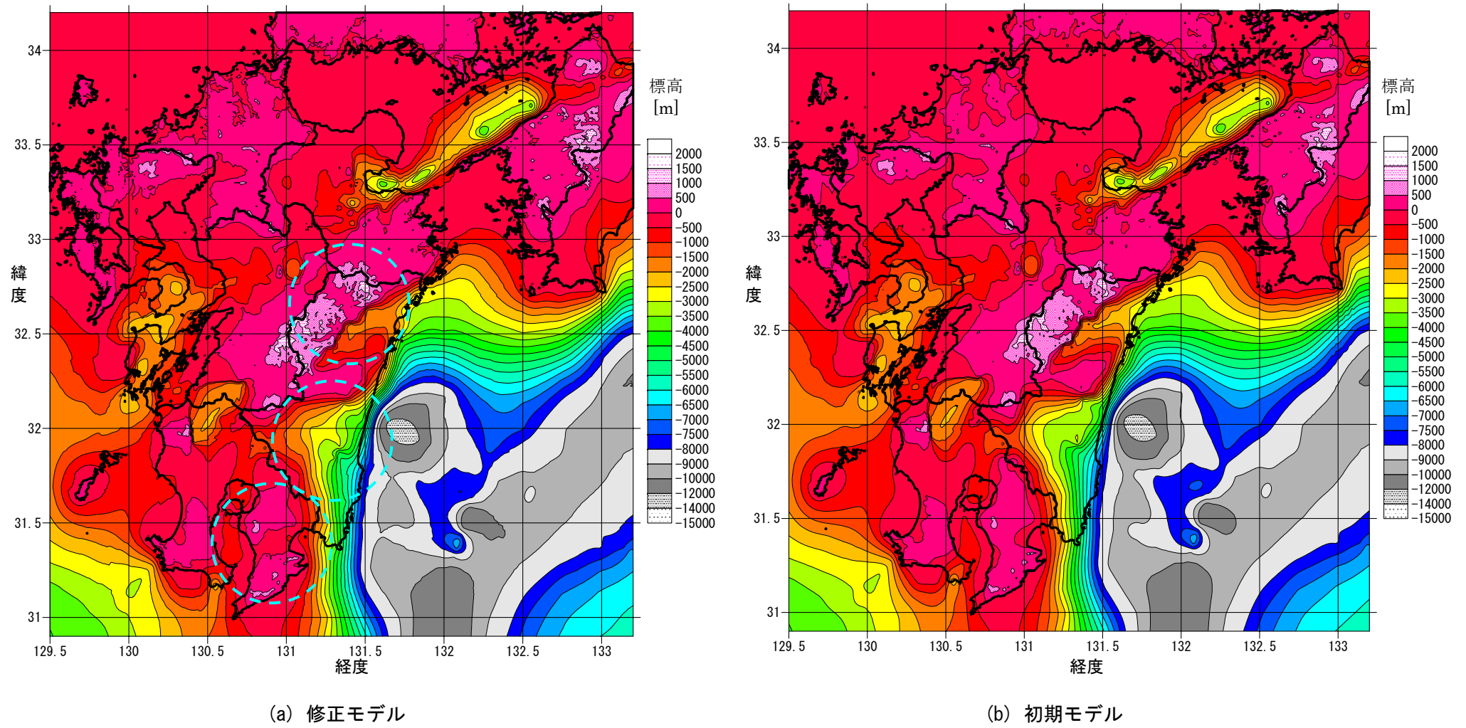
図 20-1 修正前後での三次元地下構造モデルの比較 (P 波速度 5.0km/s 層上面標高、水色の破線で囲った領域は主な修正領域を示す。)
