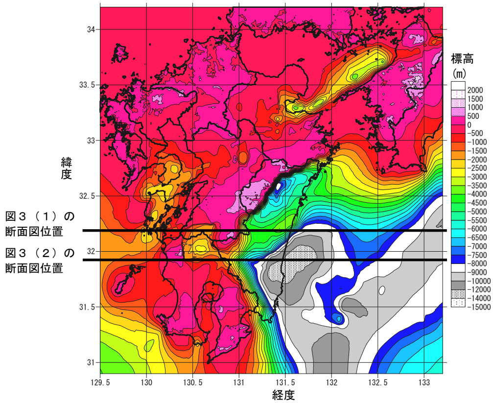
図4-1 地震基盤 (P波速度 5.5km/s 層上面) の深さ分布図 (上図は初期モデル、下図は観測記録を用いて修正したモデル)
