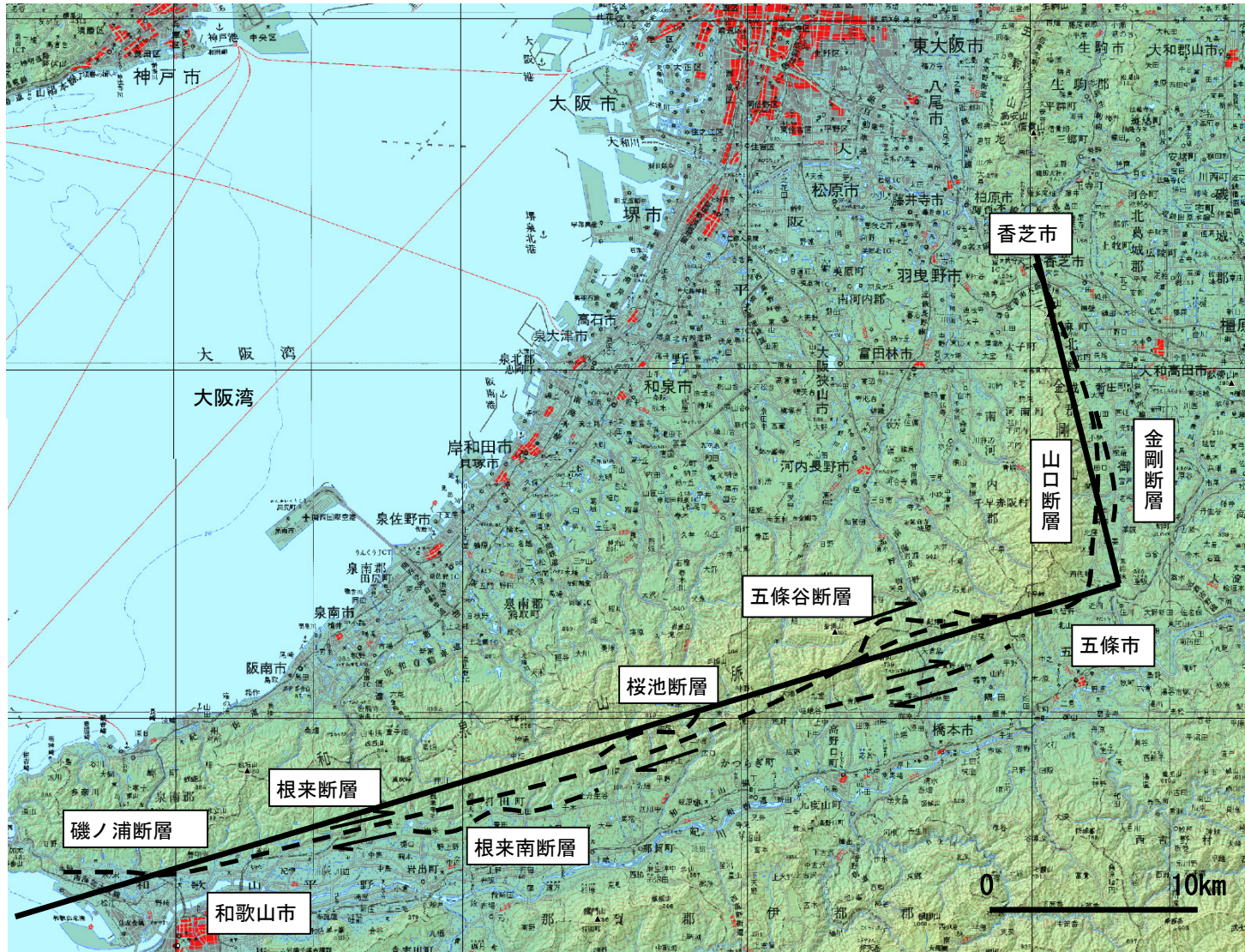
図1 中央構造線断層帯（金剛山地東縁－和泉山脈南縁）の活断層位置図（破線）と強震動評価に用いた震源断層モデルの地表トレース（実線）（地震調査委員会（2003a）に加筆）
