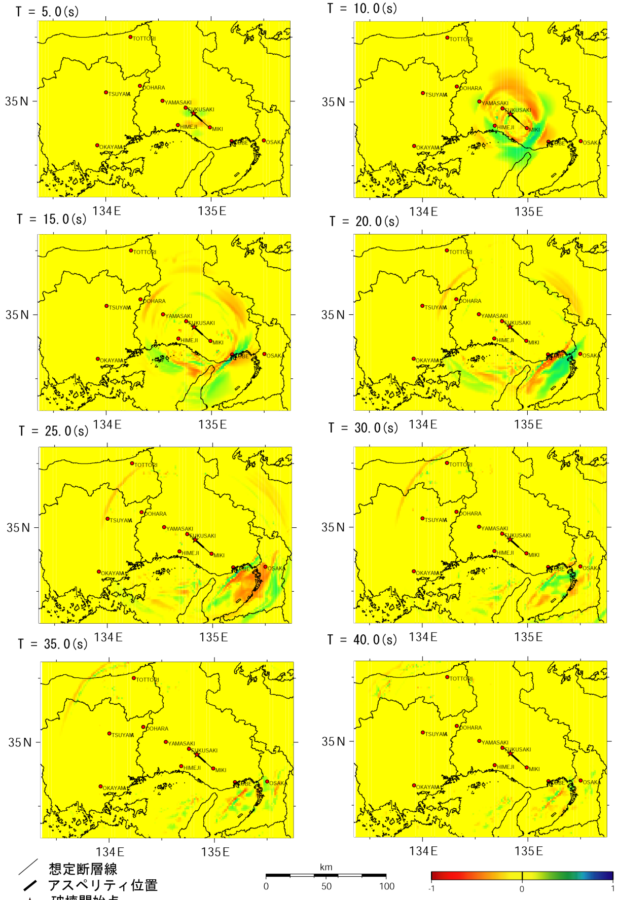
図 15-4 有限差分法による計算結果例 (モデル3、「詳細法工学的基盤」 ( V_s=550\text{m/s} 、 V_s=590\text{m/s} ) 上の速度振幅のスナップショット、NS 成分)
