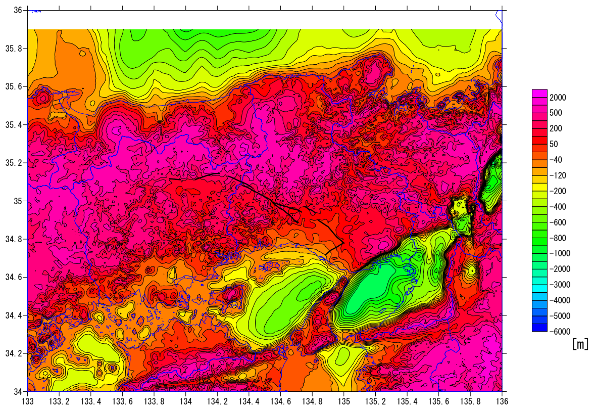
図 13-2 想定した震源断層の周辺地域における「深い地盤構造」の速度層構造 (速度層上面標高コンター、上 : V_p=2.2 \text{ km/s} ( V_s=0.71 \text{ km/s} )、下 : V_p=2.5 \text{ km/s} ( V_s=0.88 \text{ km/s} ))
