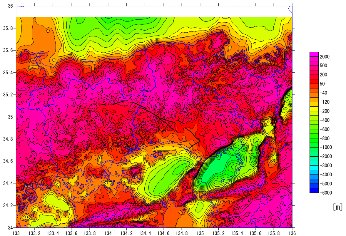
図 1 3 - 1 想定した震源断層の周辺地域における「深い地盤構造」の速度層構造 (速度層上面標高コンター、上 : V_p=1.8\text{km/s} ( V_s=0.55\text{km/s} )、下 : V_p=2.0\text{km/s} ( V_s=0.59\text{km/s} ))
