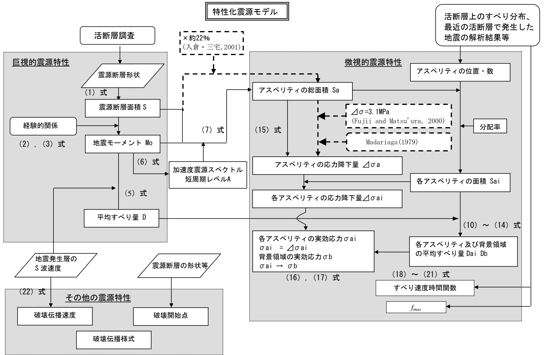
図9 活断層で発生する地震の震源特性の設定の流れ (式は付録「活断層地震の強震動評価のレシピ」の式番号に対応する。破線は今回試行的に行ったケースを表す。)
