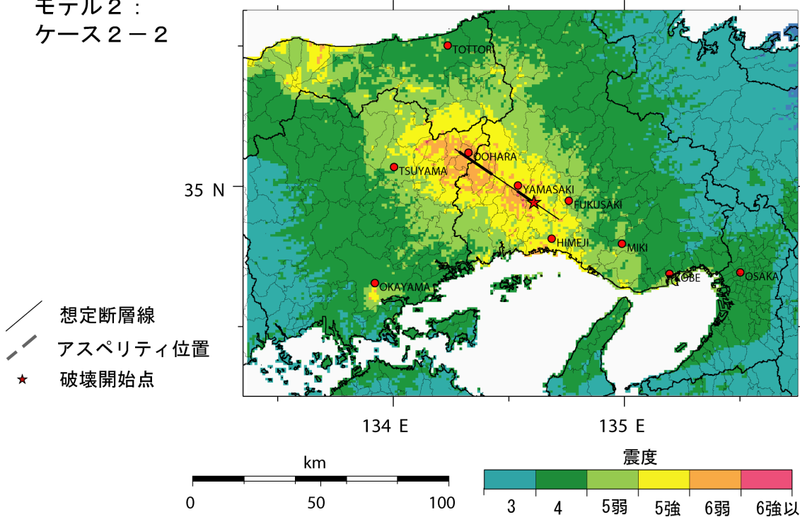
図5-2 詳細法による強震動予測結果：地表の震度分布（モデル2：ケース2-1、2-2）
