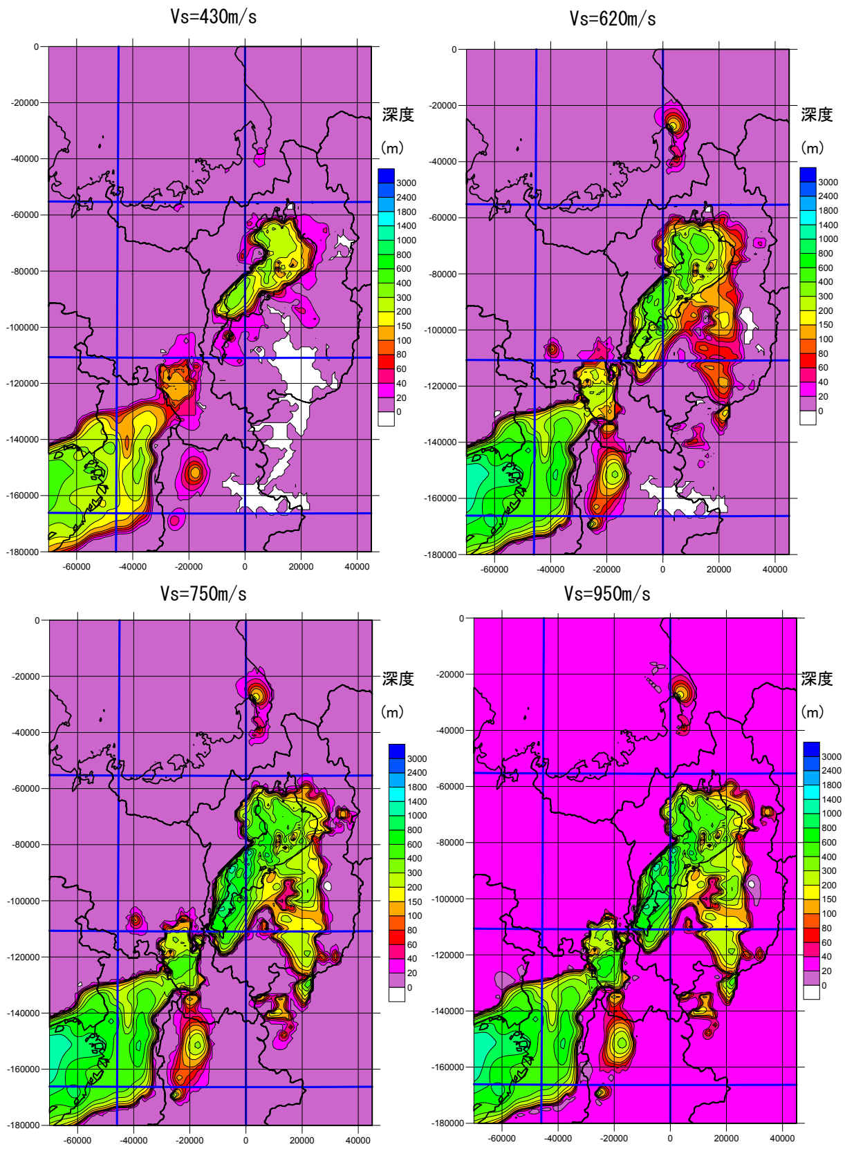
図3-1 「深い地盤構造」モデル (各速度層上面の深さ分布)
