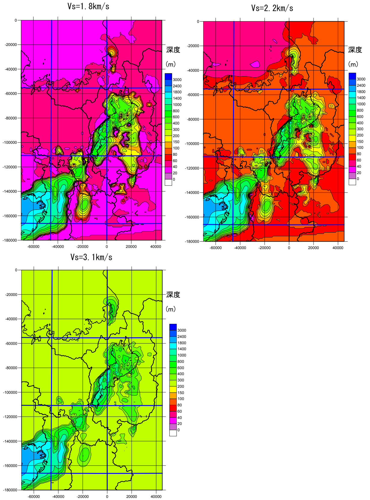
図3-2 「深い地盤構造」モデル (各速度層上面の深さ分布)
