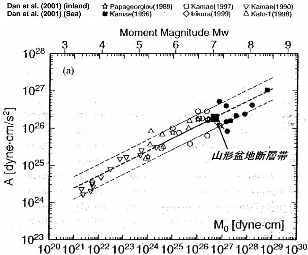
図 10 - 2 地震モーメントと短周期レベルの関係 [壇・他(2001)に加筆]
