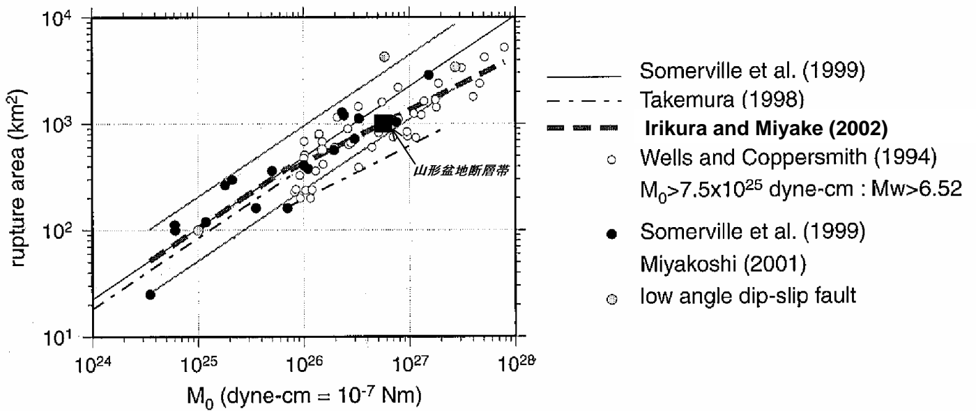
図 10 - 1 震源断層面積と地震モーメントとの関係 [入倉・三宅(2002)に加筆]
